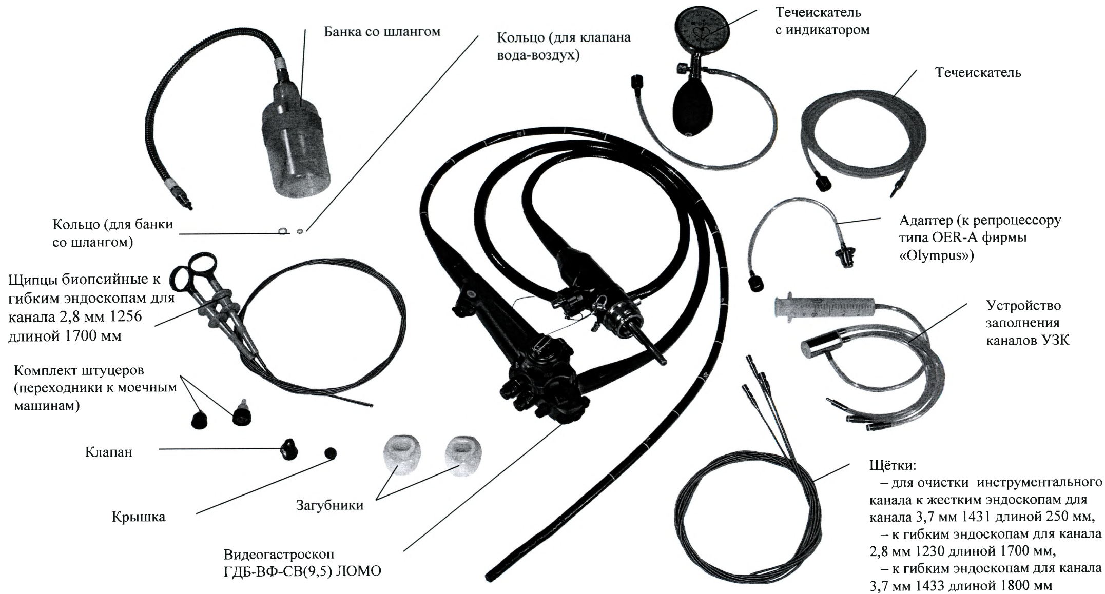
Видеогастроскоп ГДБ-ВФ-СВ(9,5) ЛОМО с принадлежностями и инструментом
