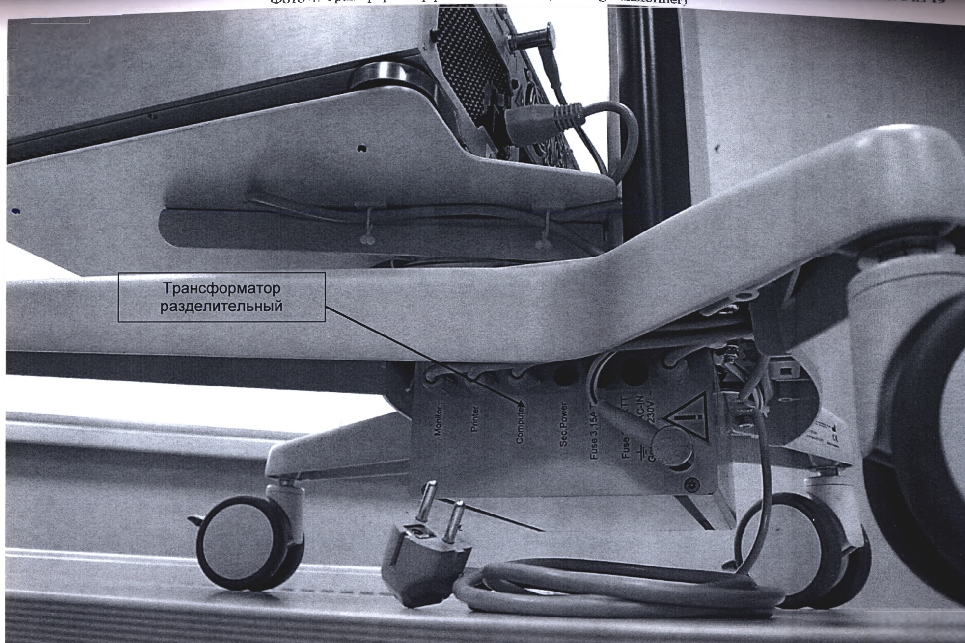
Фото 4. Трансформатор разделительный (Isolating transformer)
