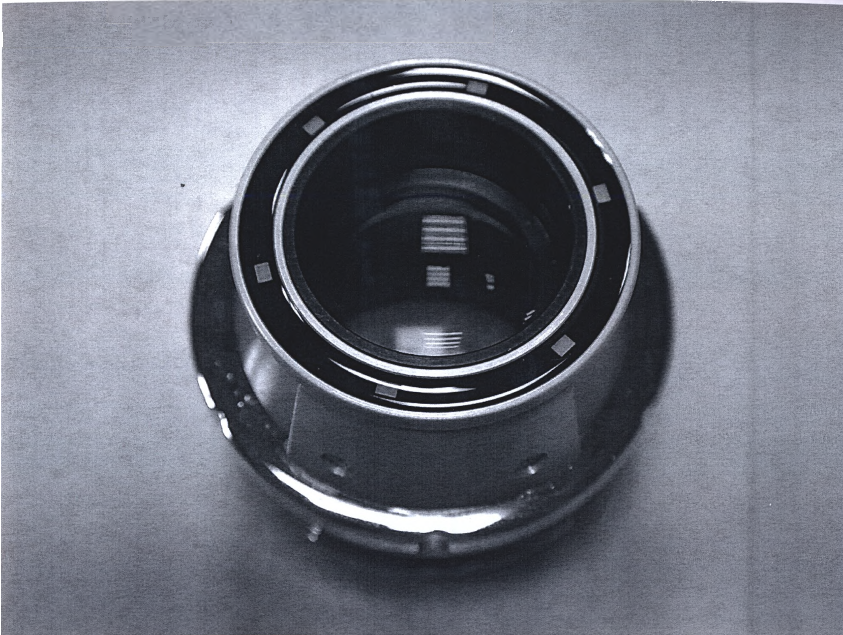
Фото 6. Объектив для дерматоскопии "Ди-Скоуп 2 Плюс Ленс" (D-Scope II Plus Lens)
