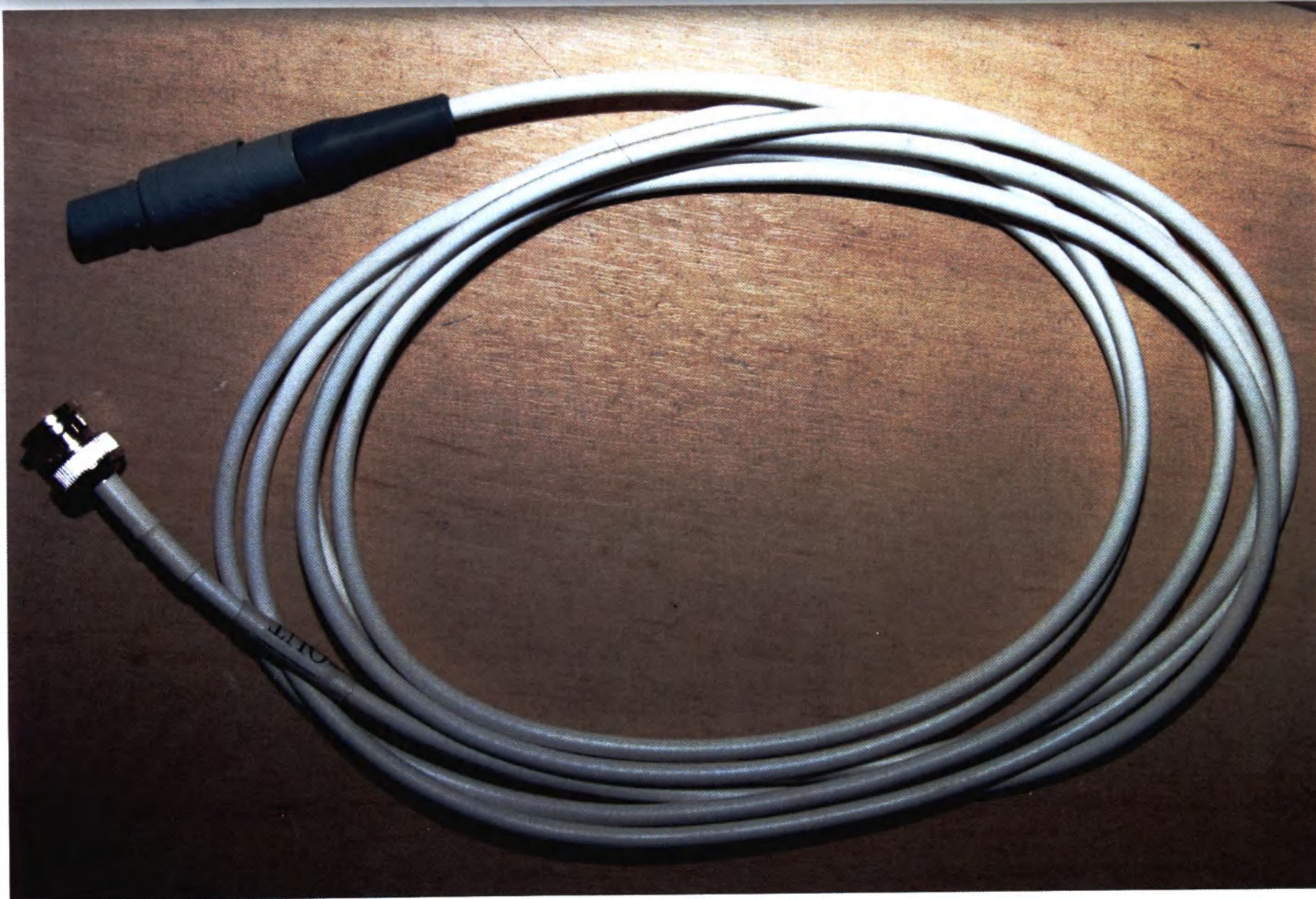
Кабель синхронизации «Нейро-ТЭС» с оборудованием других производителей (синхровыход BNC)
