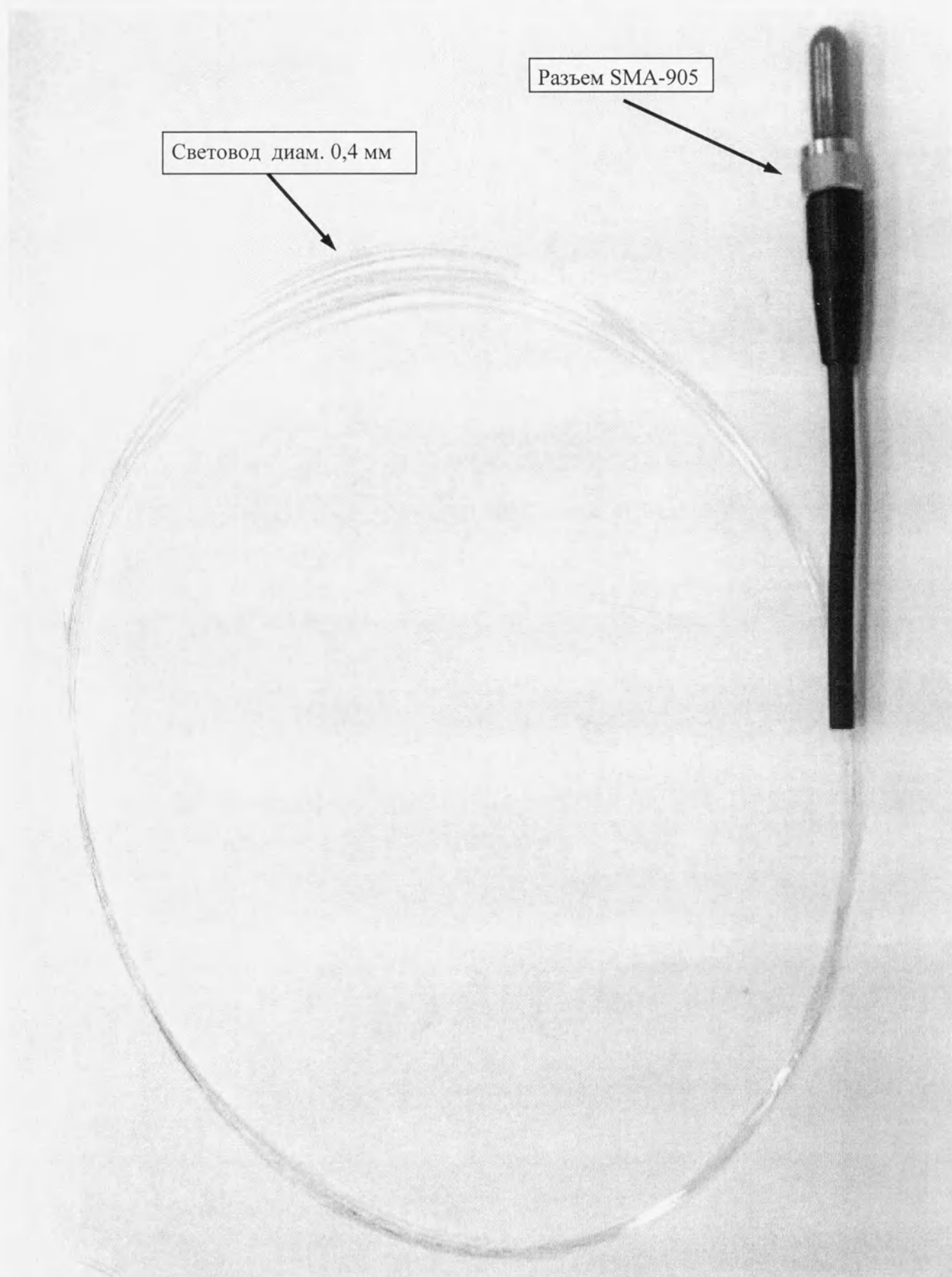
Фотография. Световод для лазерной хирургии и косметологии СЛХК 0.4
