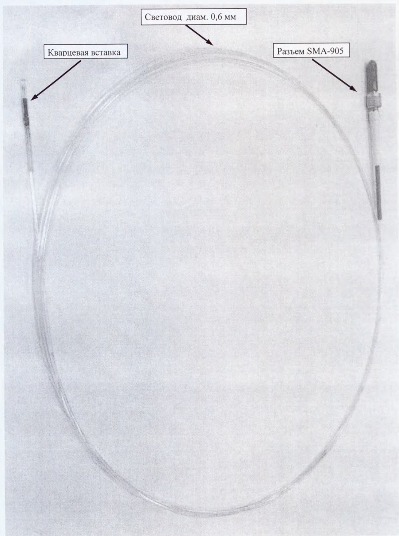
Фотография. Световод для лазерной хирургии и косметологии СЛХК 0.6-2
