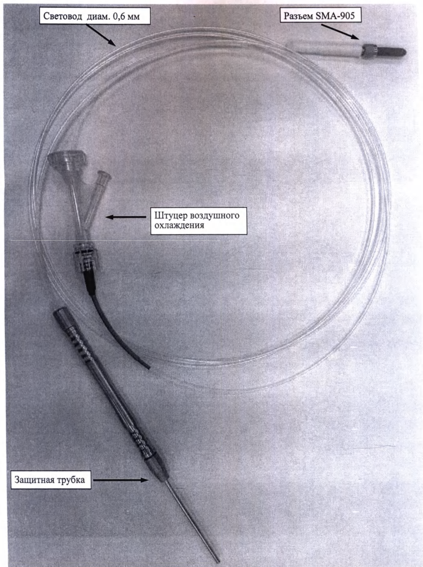
Фотография. Световод для лазерной хирургии и косметологии СЛХК 0.6-1
