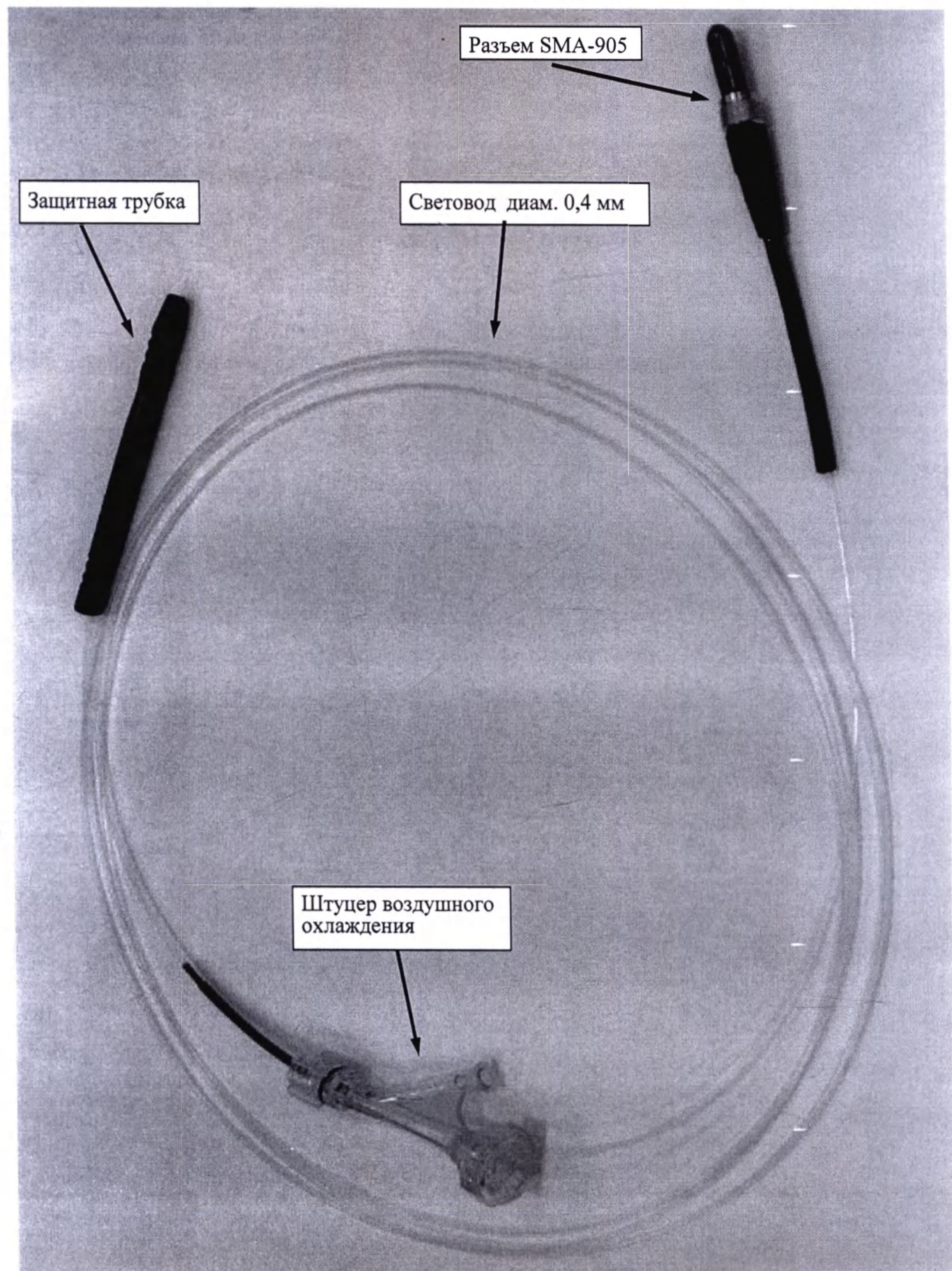
Фотография. Световод для лазерной хирургии и косметологии СЛХК 0.4-1
