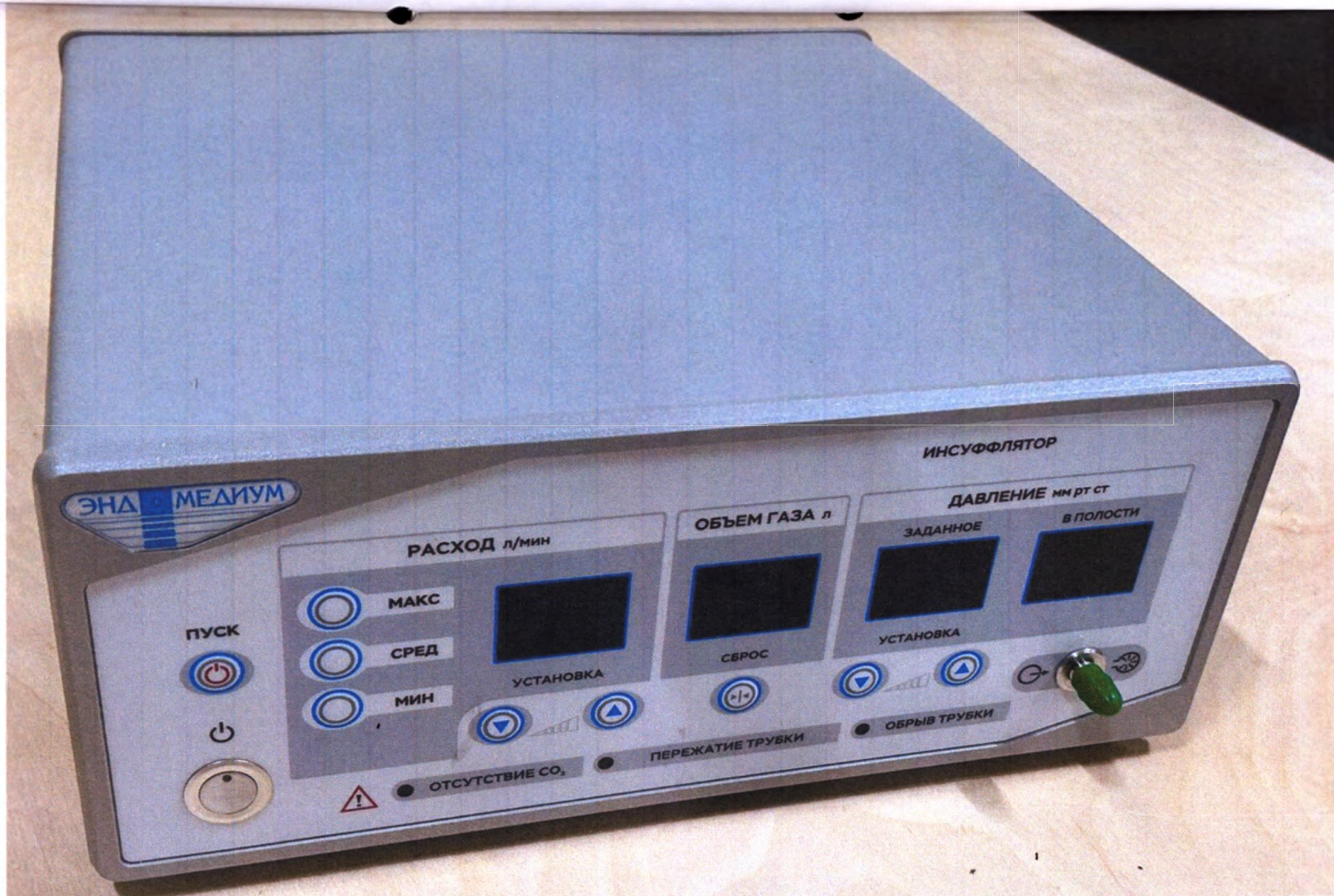
Фото 1.1 Инсуффлятор EndoSteam® I (вид спереди)
