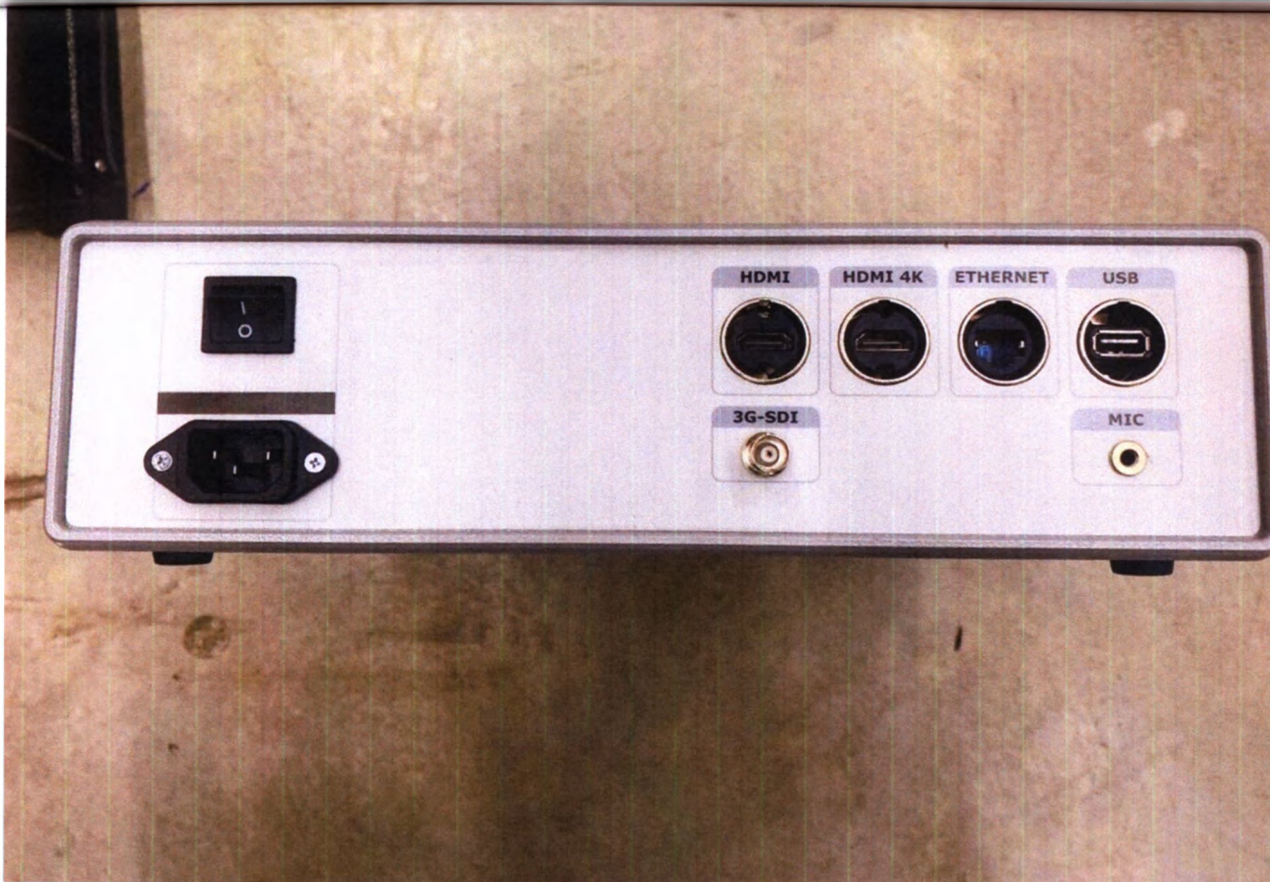
Фото 9.2 Блок обработки видеосигнала EndoGlance® ULTRA HD (задняя панель)
