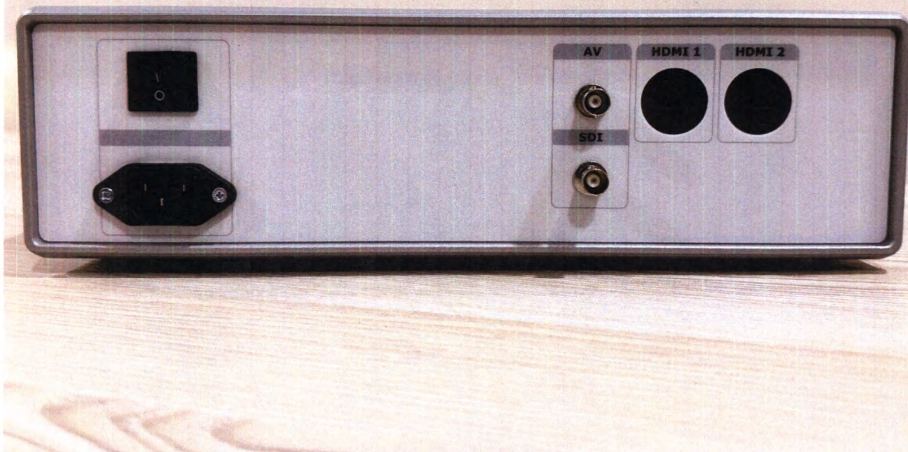
Фото 12.2 Блок обработки видеосигнала EndoGlance® HD (задняя панель)
