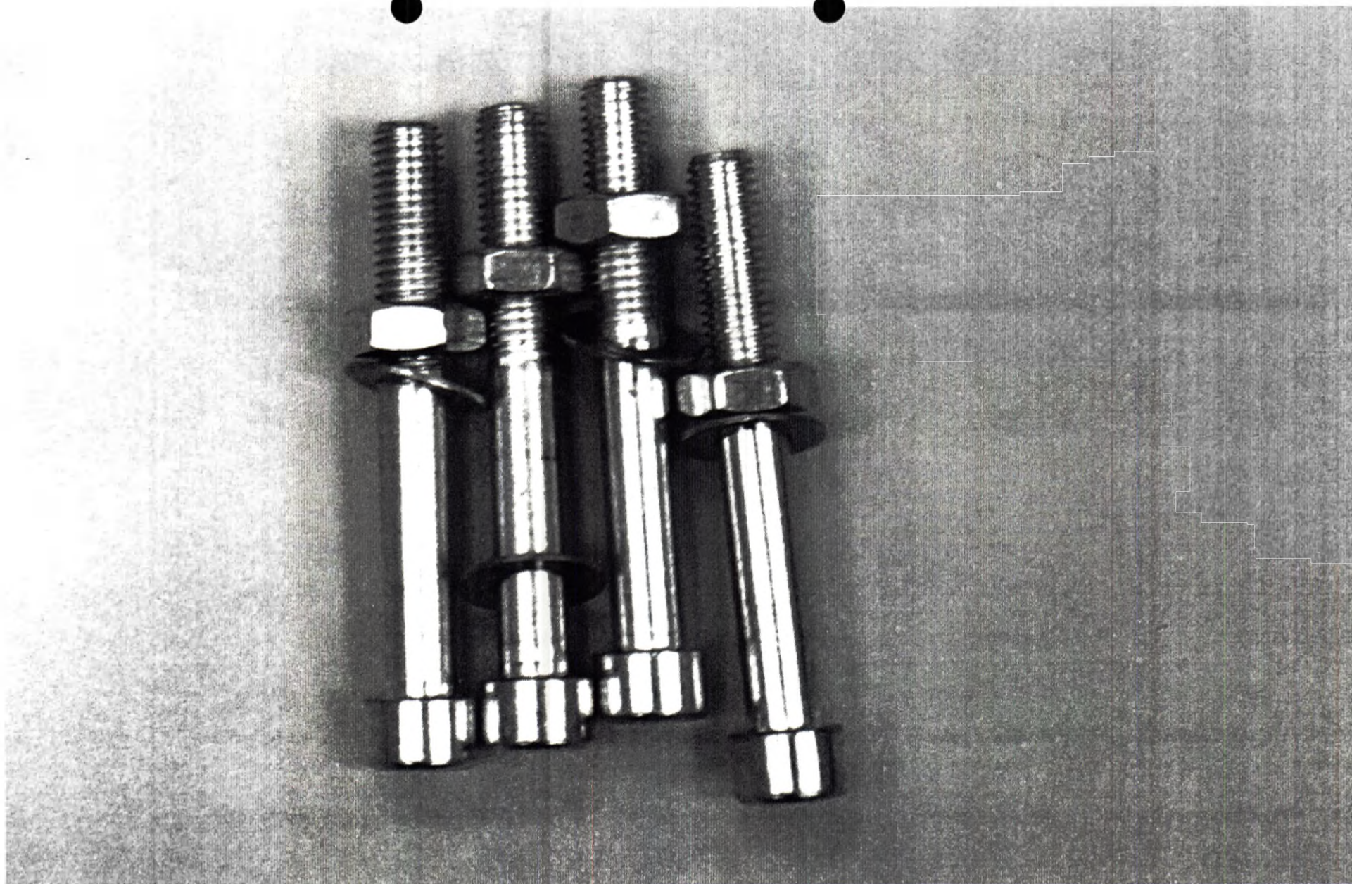
Стол медицинский с электроприводом СО-1 по ТУ 32.50.30-008-01324118-2021 с принадлежностями. Принадлежности: болт (Ø8, L=65 мм) крепления опоры с шайбой и гайкой
