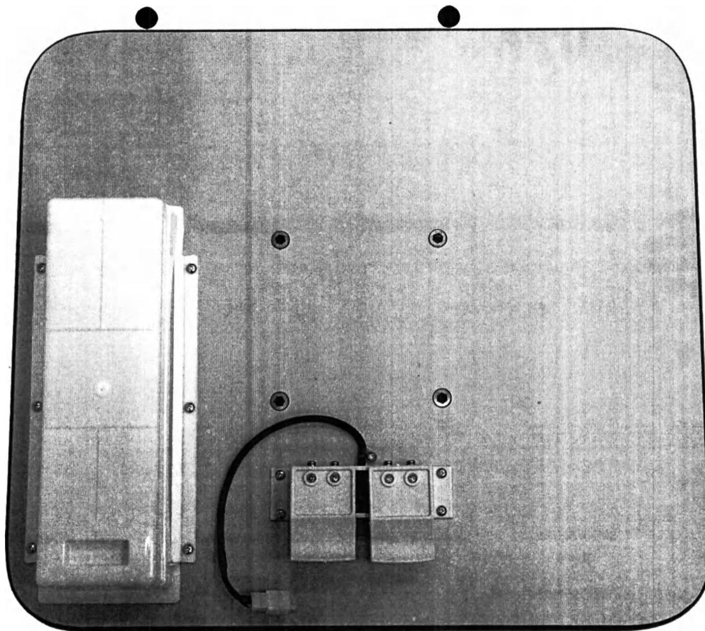
Стол медицинский с электроприводом СО-1 по ТУ 32.50.30-008-01324118-2021 с принадлежностями. Столешница (вид снизу)
