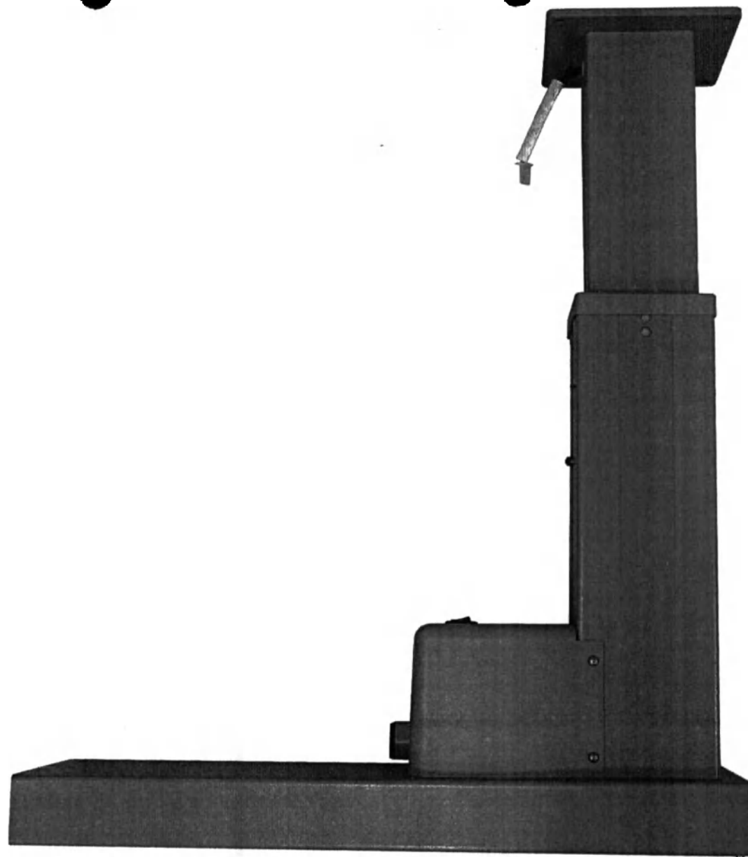
Стол медицинский с электроприводом СО-4 по ТУ 32.50.30-008-01324118-2021 с принадлежностями. Основание стола с механизмом подъёма в сборе
