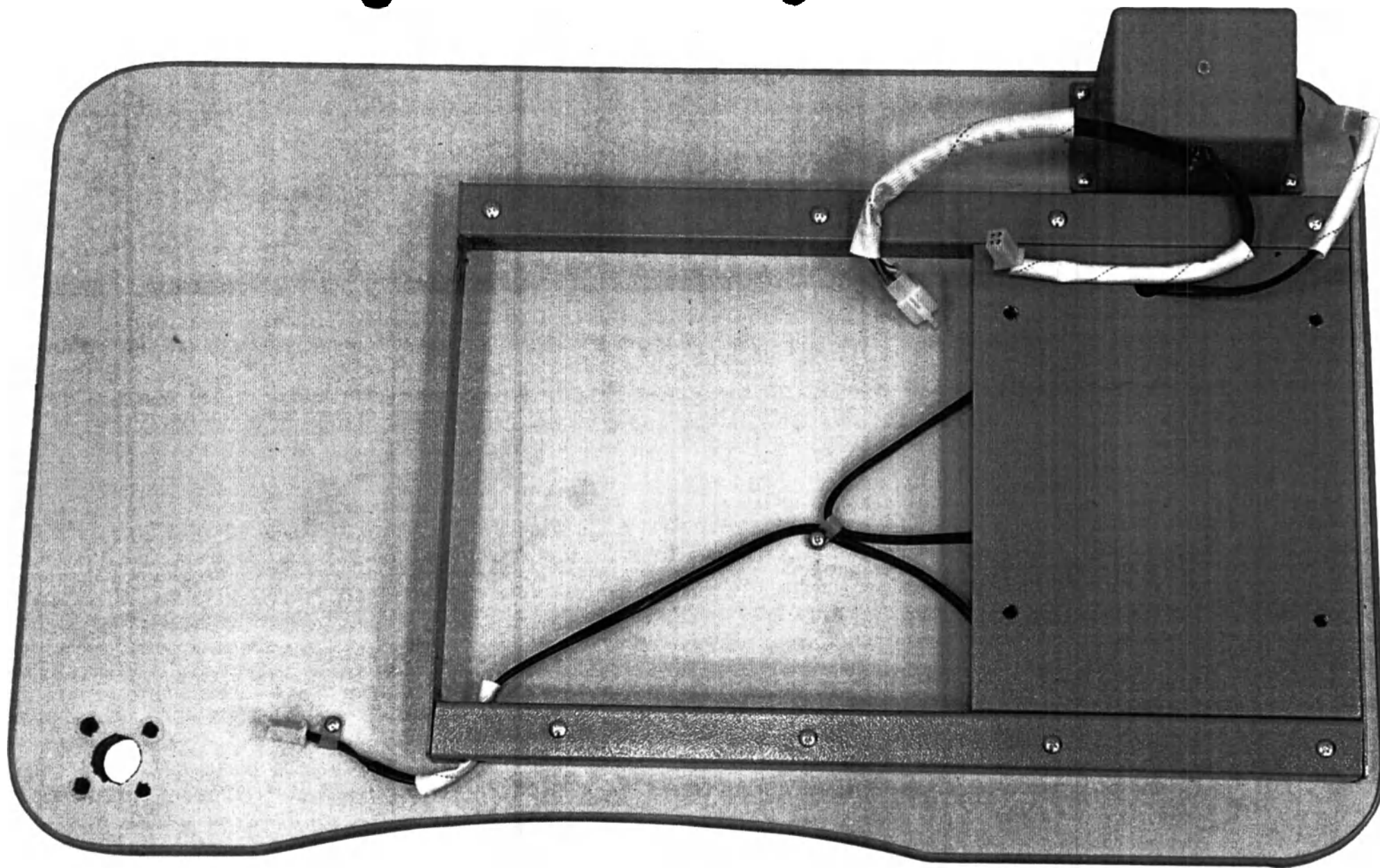
Стол медицинский с электроприводом СО-3 по ТУ 32.50.30-008-01324118-2021 с принадлежностями. Столешница (вид снизу)
