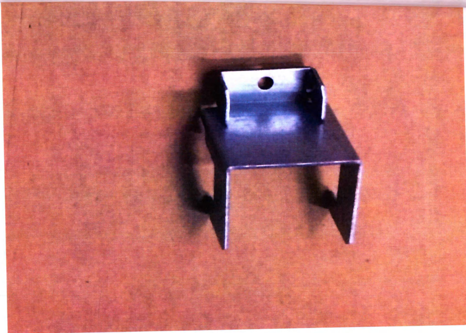
Стальной крепеж коннектора батареи для удержания в разъеме ИБП
