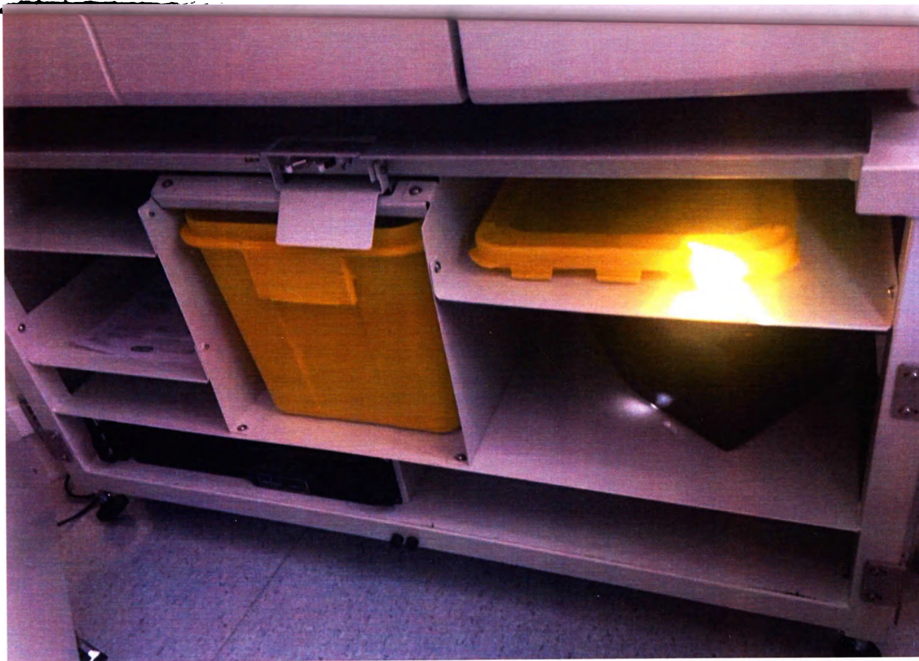
Установочный стол IH-500 с рабочей станцией и бункером для твердых отходов (IH-500 optional table with workstation and solid waste bin) (дверца открыта)
