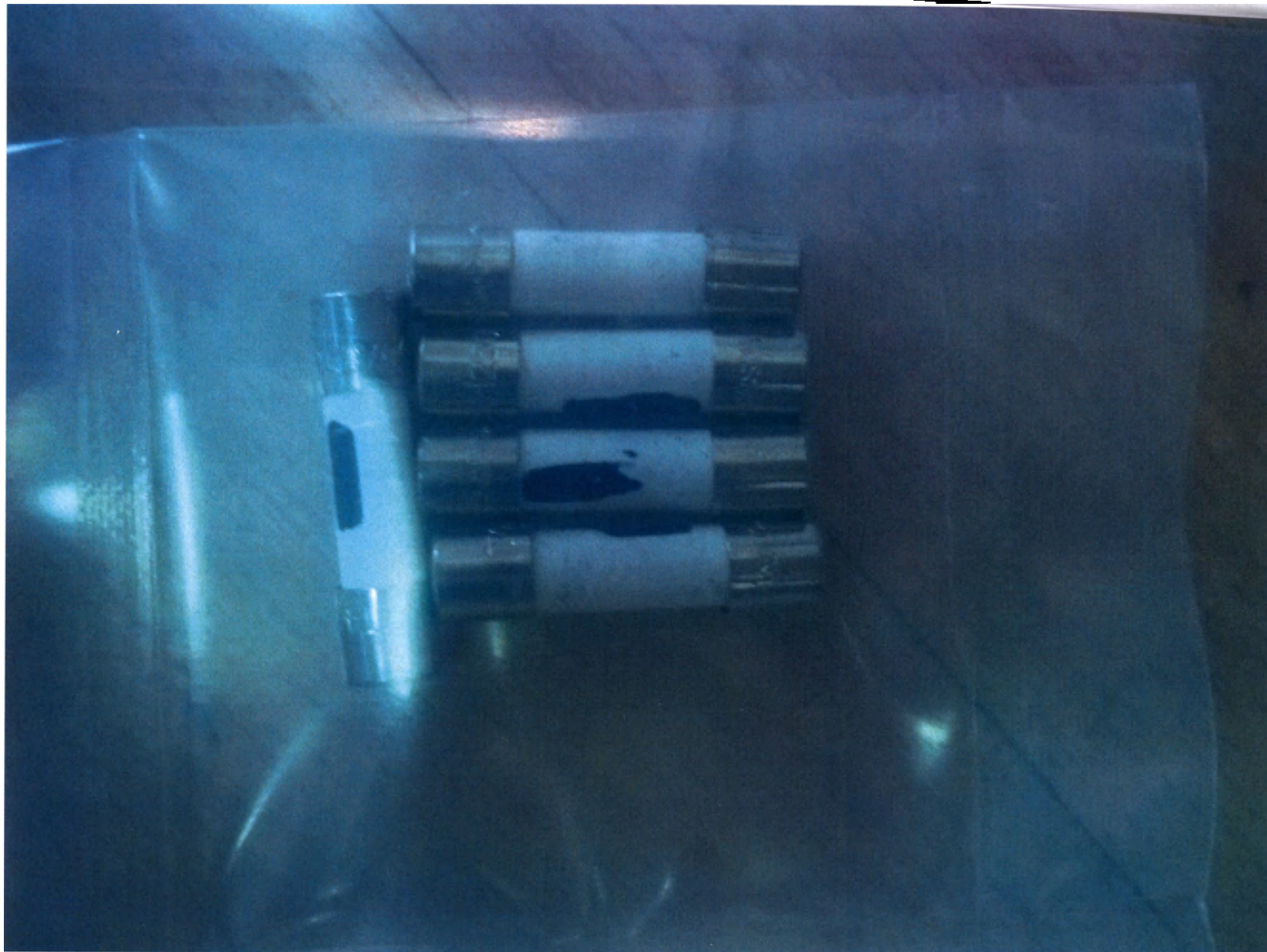
Фото 7. Предохранитель плавкий Т4А НРС
