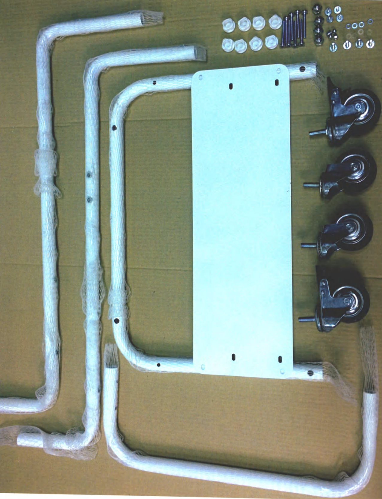
Комплект для сборки подвижного основания
