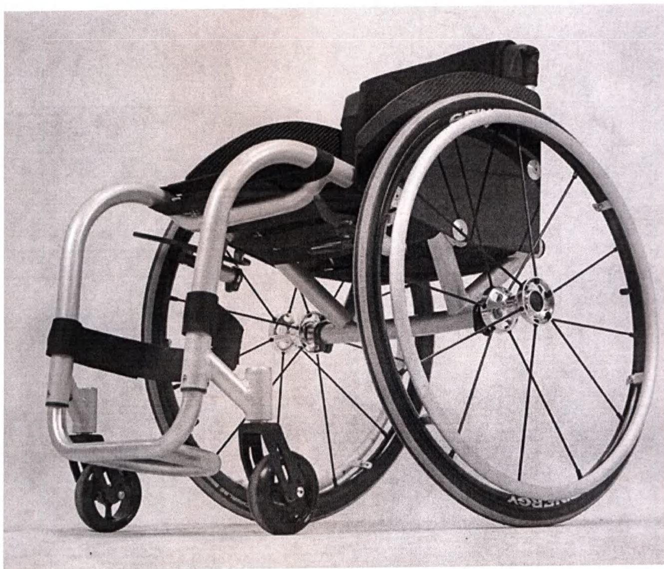
Рисунок 2. Кресло-коляска механическая NAVIK, вариант исполнения: NAVIK N2 в сборе
