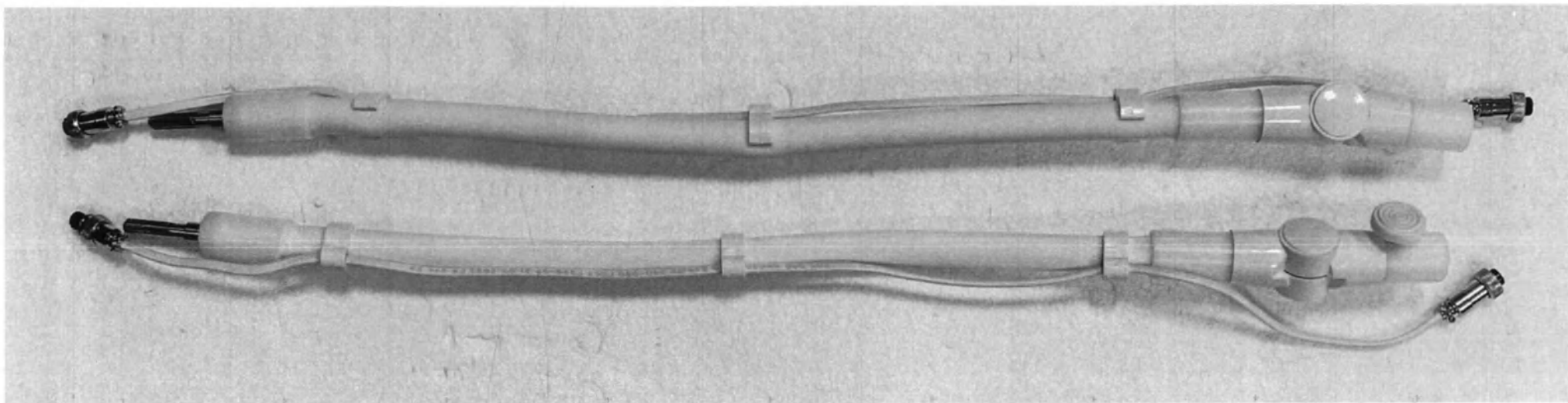
Гибкий индуктородержатель (в сборе)
