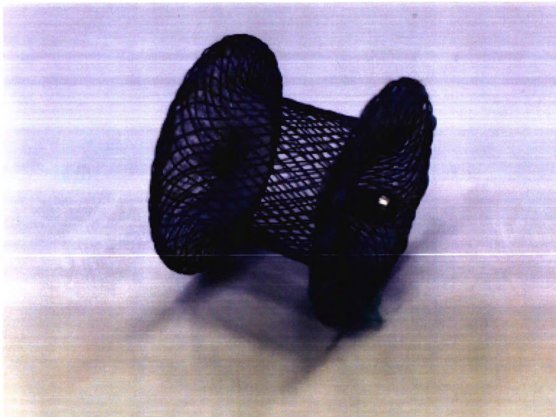
Вариант исполнения медицинского изделия «Окклюдер кардиологический «TVA Plug» по ФСПБ. 942511.001 ТУ». Окклюдер для закрытия мышечного дефекта межжелудочковой перегородки симметричный (VSD-MUSC-S). Внешний вид.
