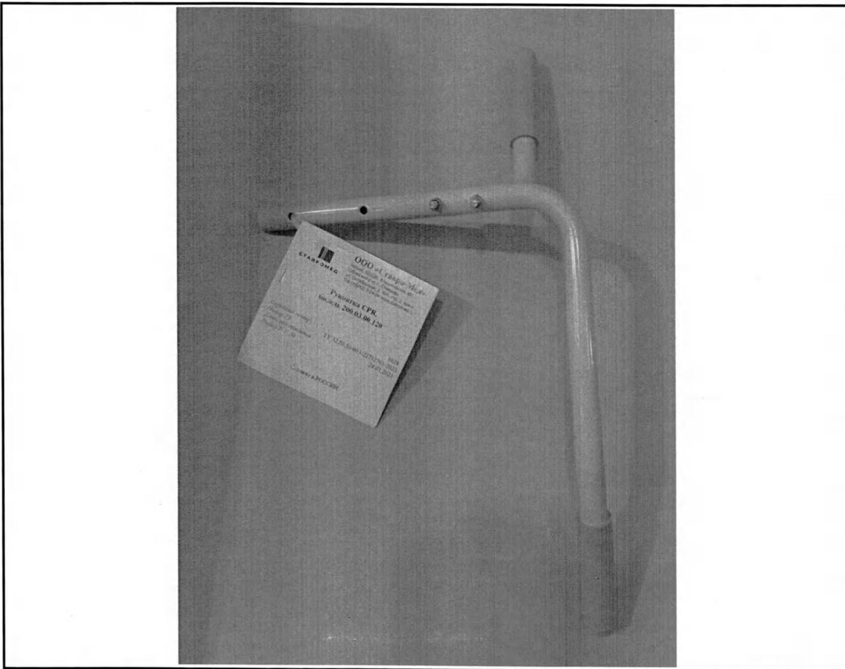
Рукоятка CPR, модель 200.03.00.120.
