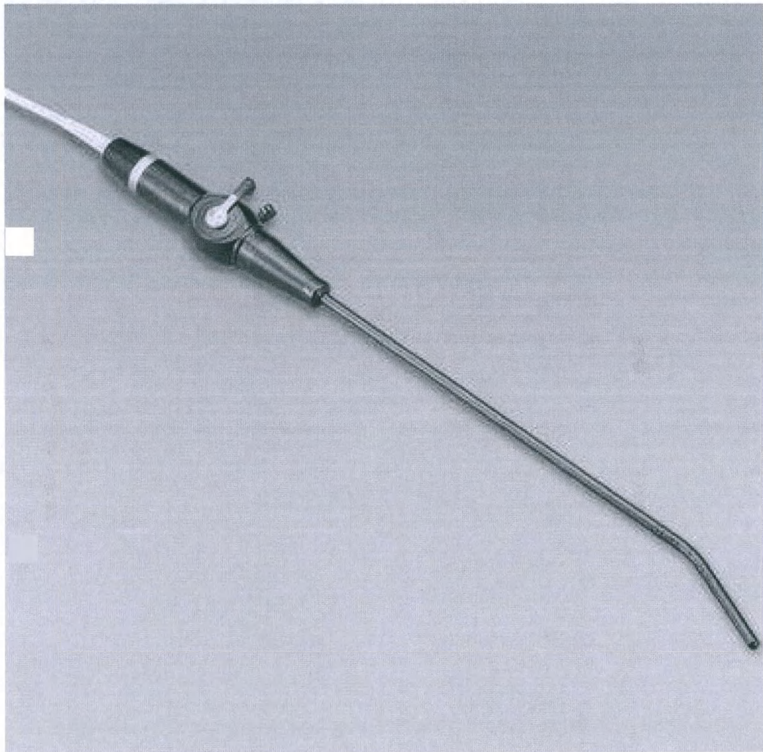
68. Линейный лапароскопический датчик UST-5550 для аппарата ультразвукового диагностического, с диапазоном частот 4-13 МГц и апертурой 30 мм.
