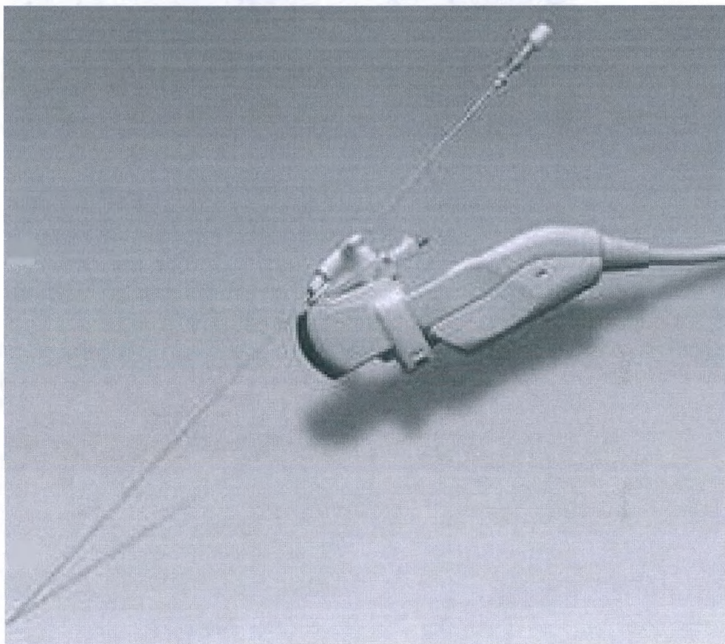
19. Конвексный абдоминальный датчик С22Р для аппарата ультразвукового диагностического, с диапазоном частот 1-6 МГц и углом обзора 74°.
