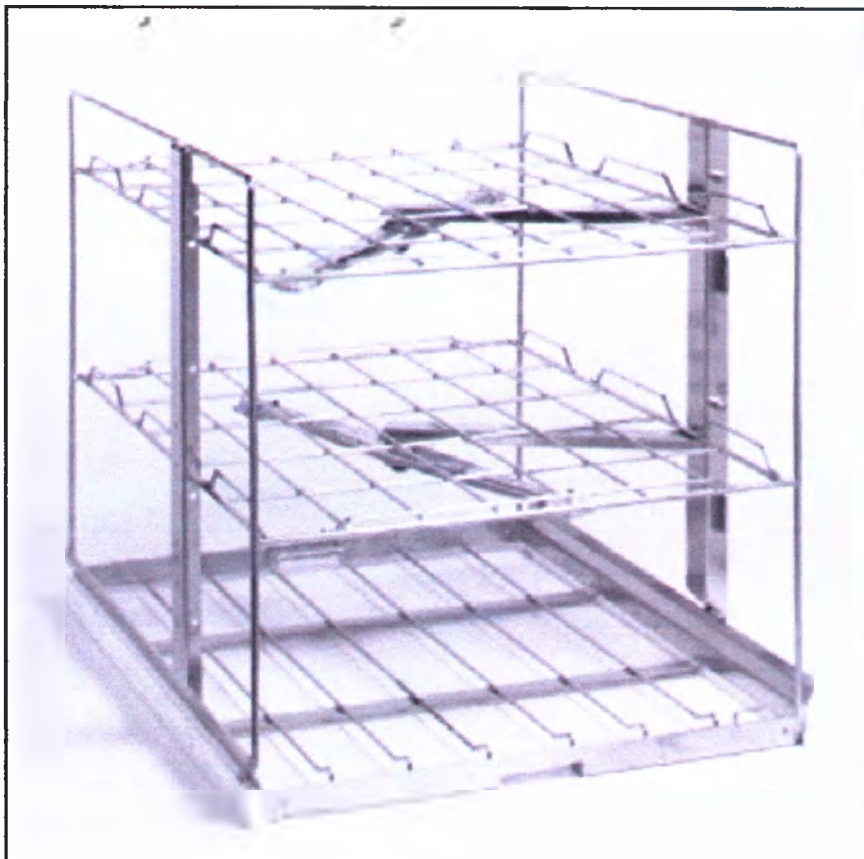
66. Вставка трехуровневая с двумя моечными коромыслами
