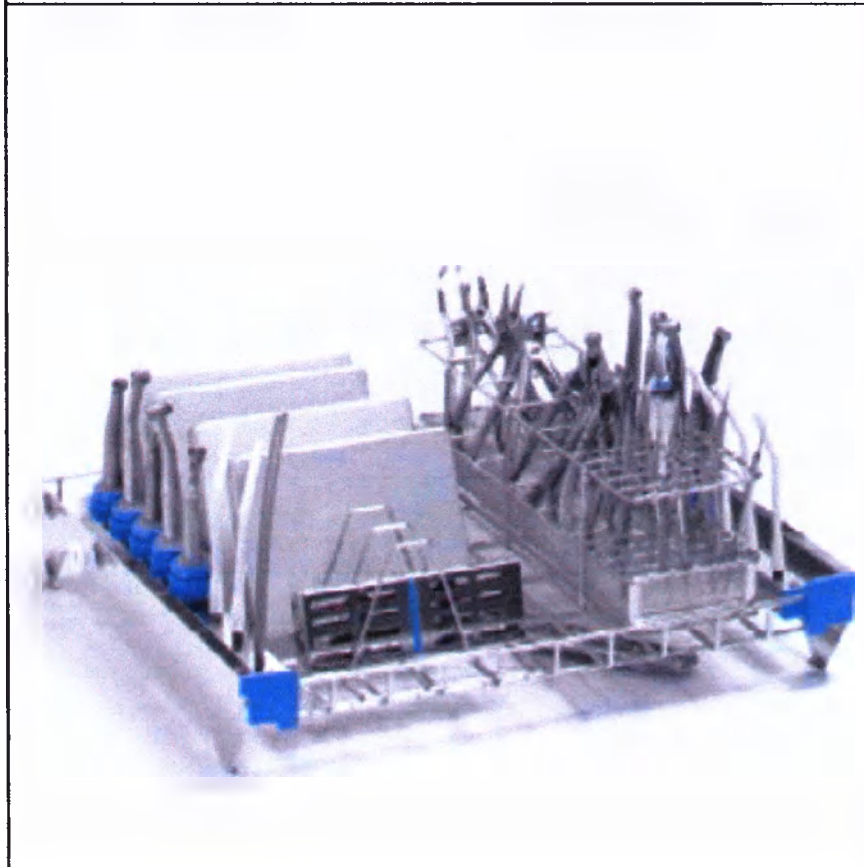
48. Вставка дентальная верхняя для 10 промывочных втулок и 6 инжекторных сопел
