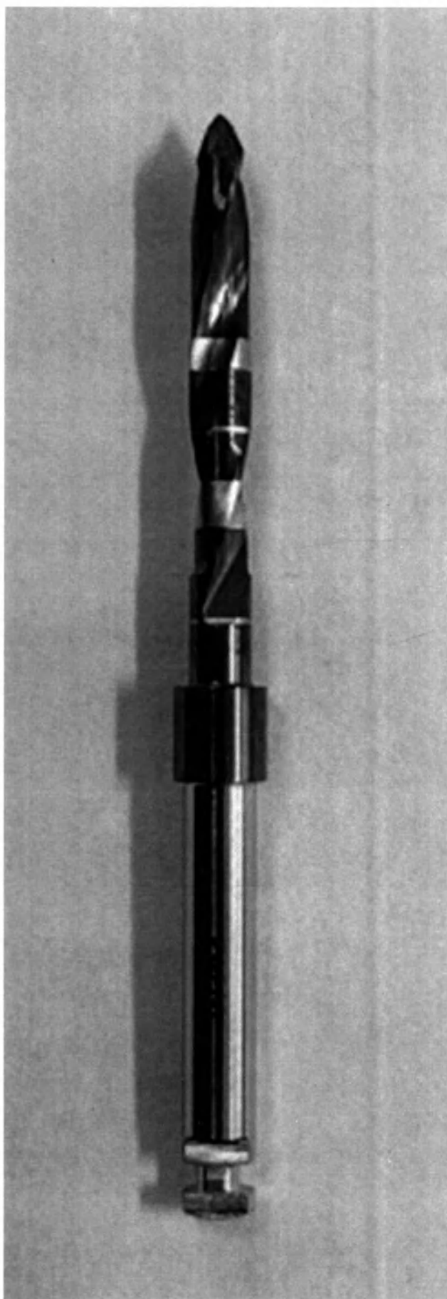
Рисунок 1 - Сверло IF/CF пилотное среднее диаметр 2 мм, Сверло IF/CF пилотное длинное диаметр 2 мм, Сверло IF/CF пилотное короткое диаметр 2 мм
