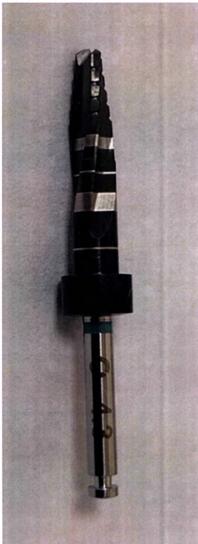
Рисунок 4 - Сверло IF/CF коническое среднее для имплантата диаметром 4,3 мм с ограничителем, Сверло IF/CF коническое длинное для имплантата диаметром 4,3 мм с ограничителем, Сверло IF/CF коническое короткое для имплантата диаметром 4,3 мм с ограничителем
