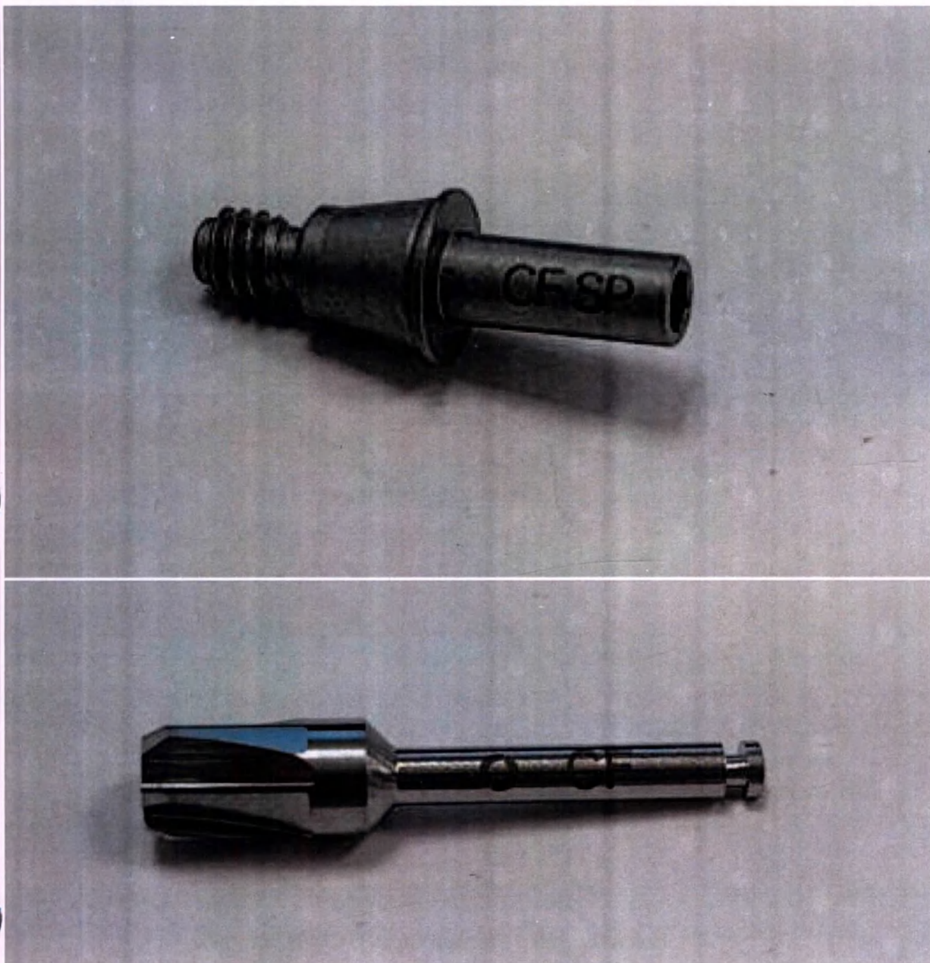
Рисунок 17 - Сверло профильное с направляющей CF SP
