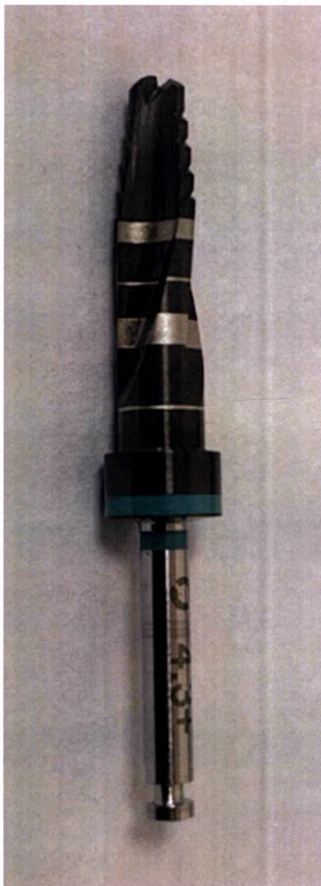
Рисунок 8 - Сверло IF/CF коническое для плотной кости для имплантата диаметром 4,3 мм с ограничителем
