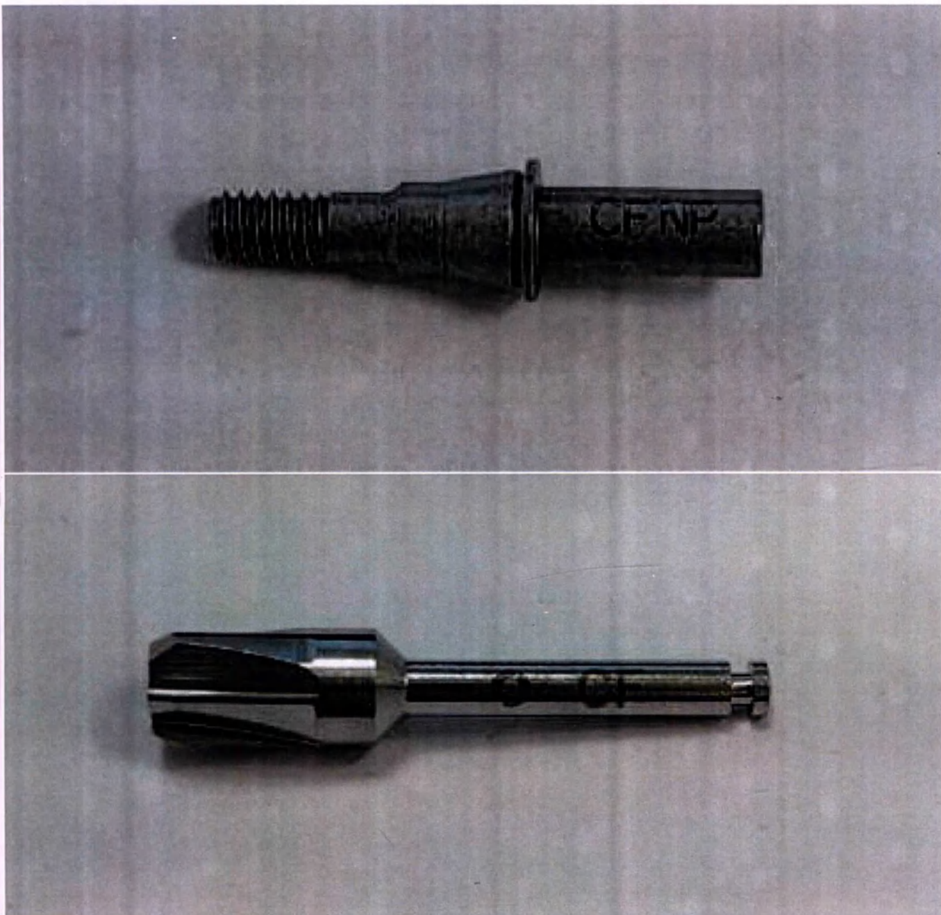
Рисунок 18 - Сверло профильное с направляющей CF NP
