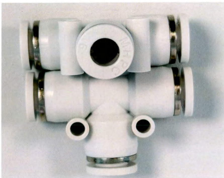
Блок трехходовой РЕ-6
