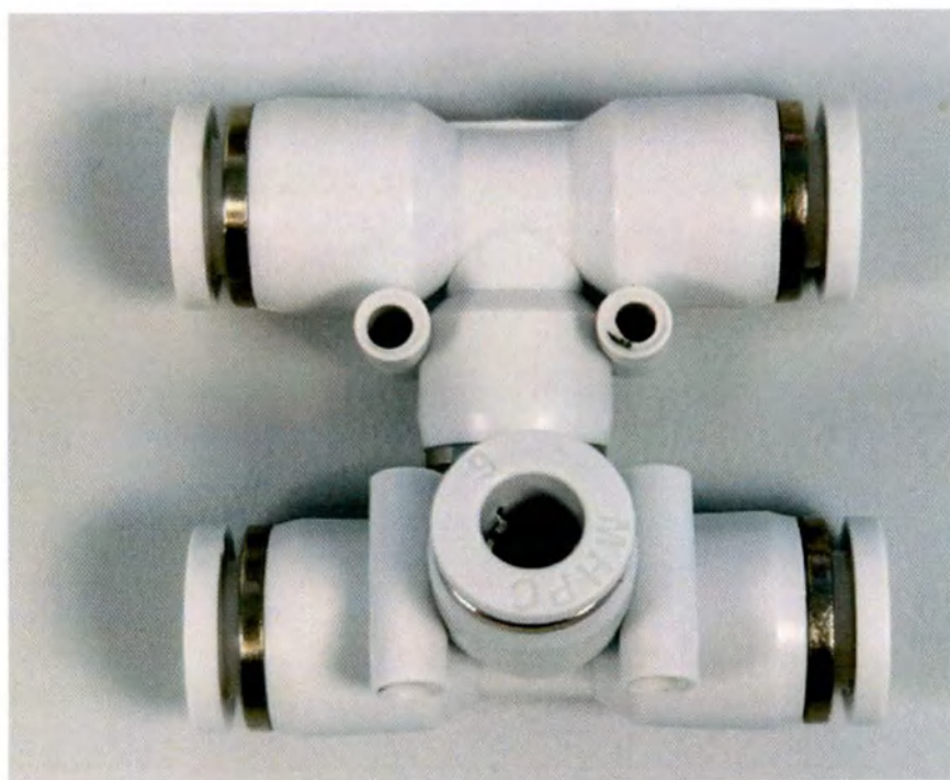
Блок трехходовой PEG8-6-8
