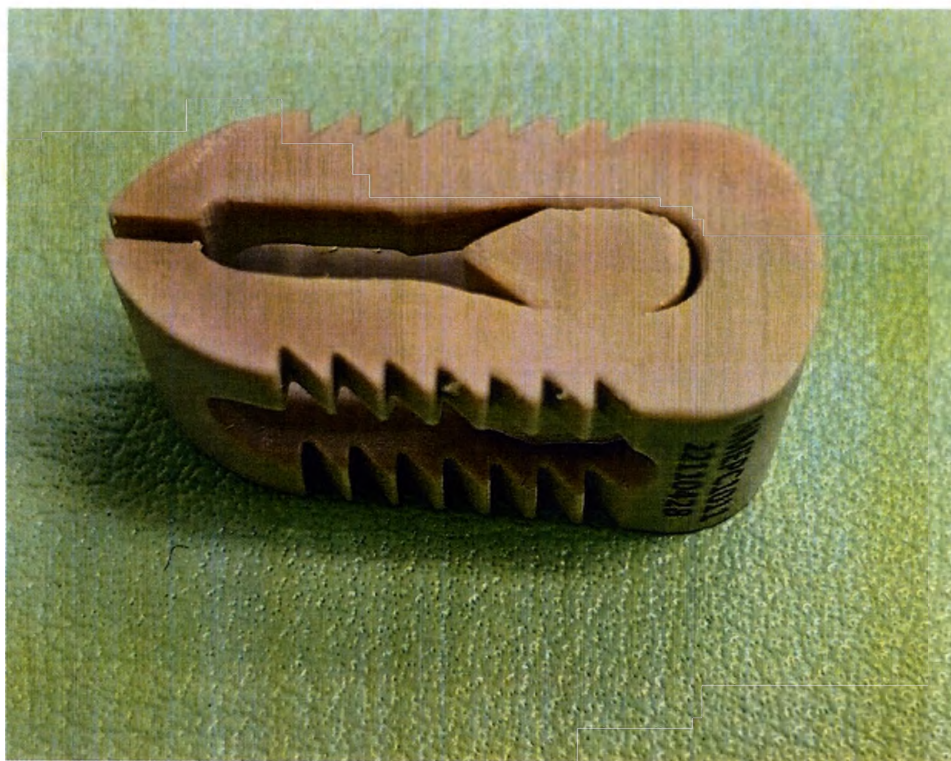
Рис.6. Медицинское изделие: Кейдж Normmed межтеловой, расширяемый, Alligator, груднопоясничный, размер: (H) 11 мм x (L) 24 мм x (W) 10 мм.
