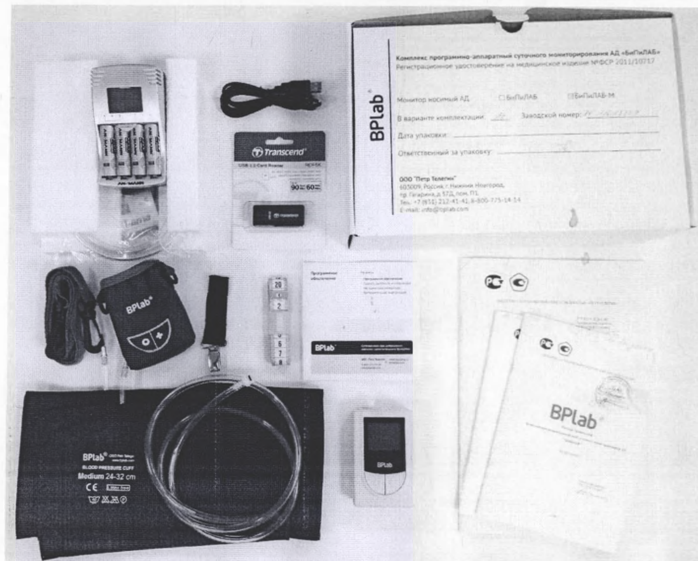
Комплекс программно-аппаратный суточного мониторинга АД "БиПиЛАБ" по ТУ 9441-002-39238870-2010, производства ООО «Петр Телегин», Россия, РУ № ФСР 2011/10717
