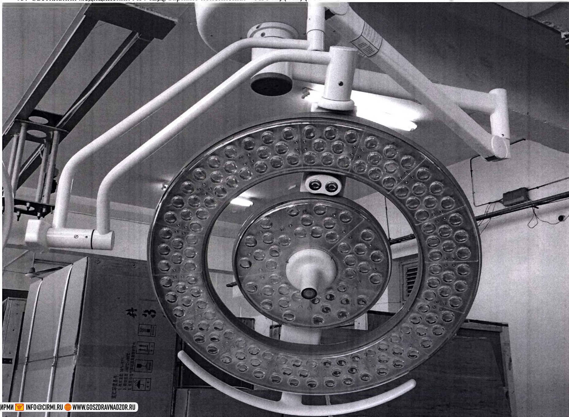
13. Светильник медицинский АРМЕД, вариант исполнения – АРМЕД-ЛЕД 750-ТВ
