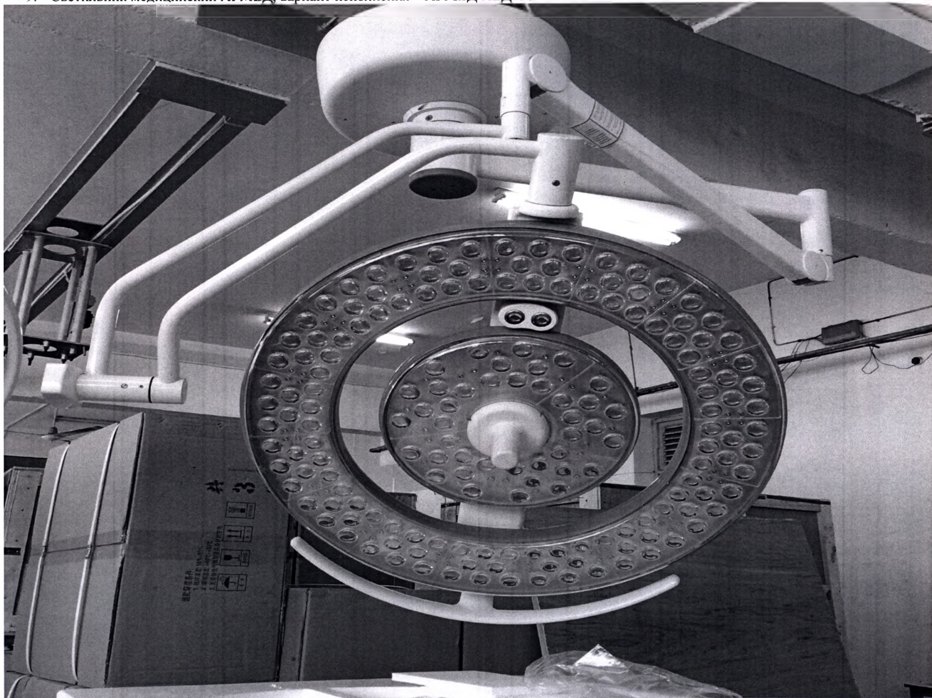
9. Светильник медицинский АРМЕД, вариант исполнения – АРМЕД-ЛЕД750
