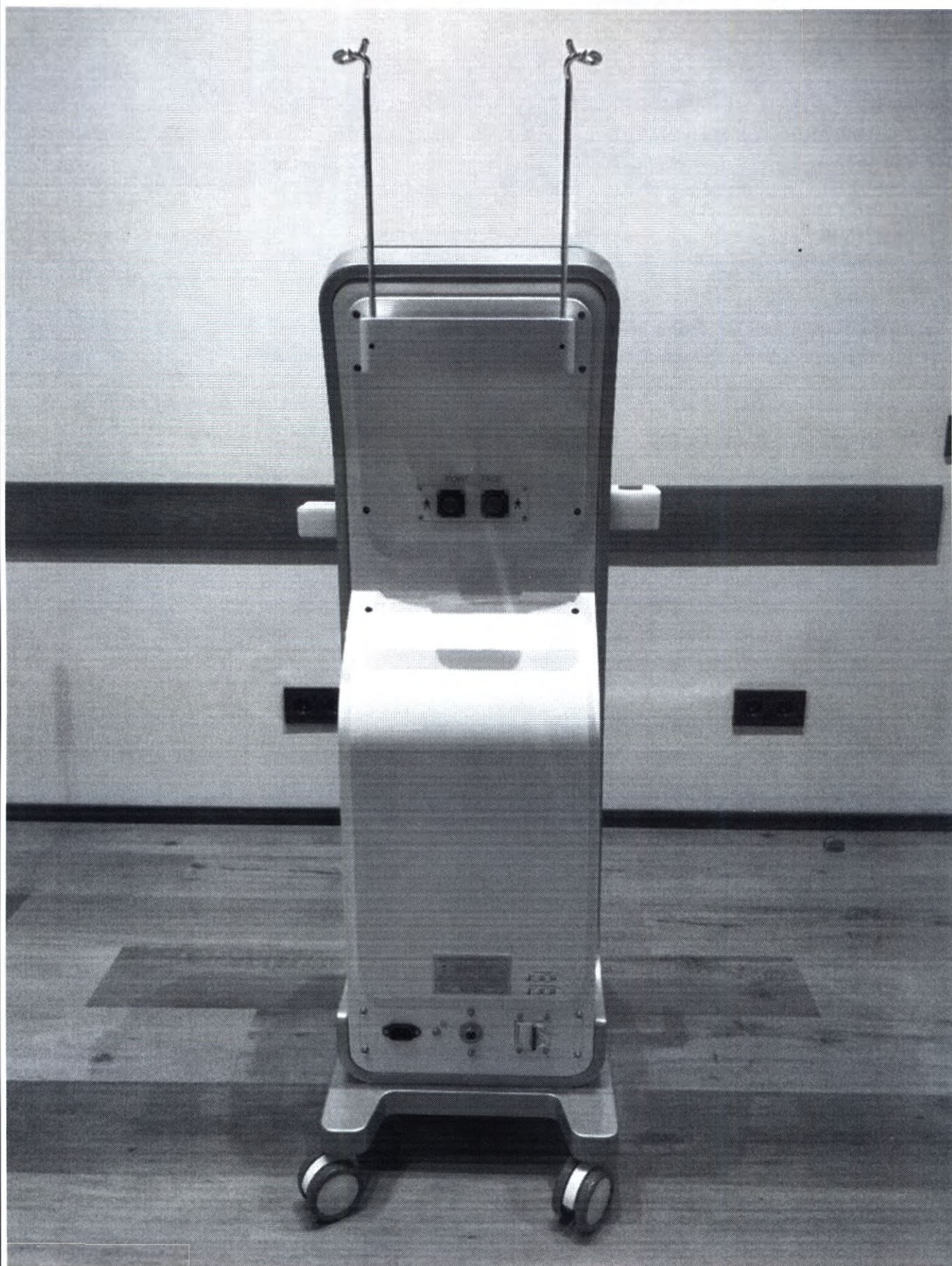
Блок основной HI-REX в сборе . Вид сзади
