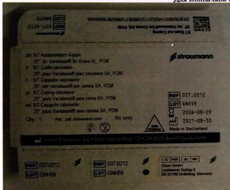
Маркировка потребительской упаковки
