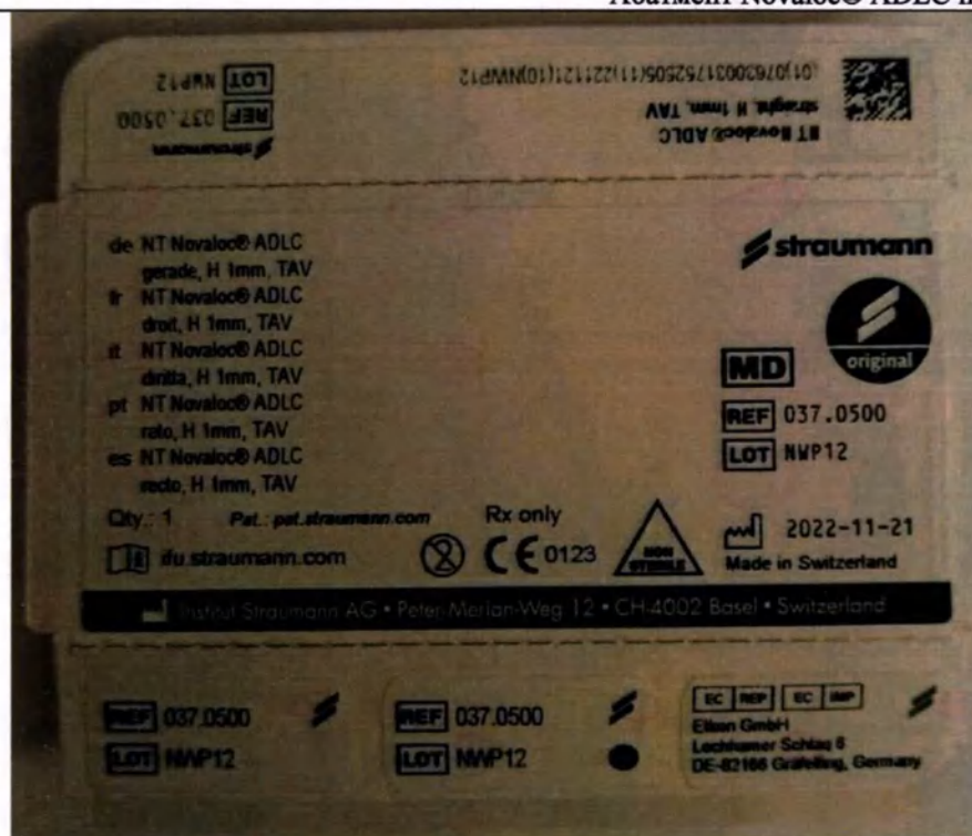
Маркировка потребительской упаковки (на примере Абатмент Novaloc® ADLC прямой, NT, высота 1 мм)
