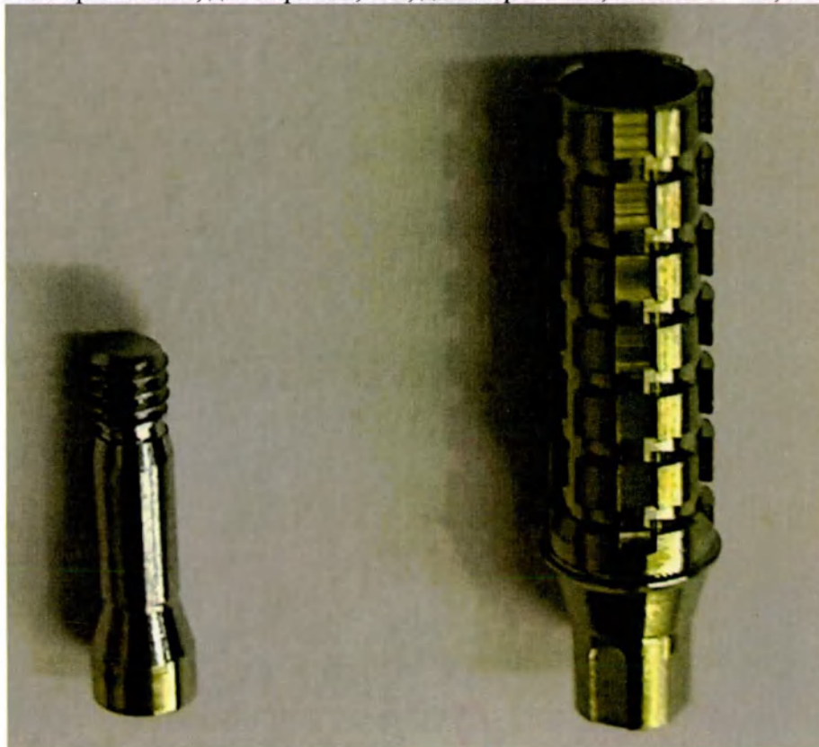
Абатмент временный, для коронки, NC, диаметр 3.5 мм, высота 11 мм, с винтом
