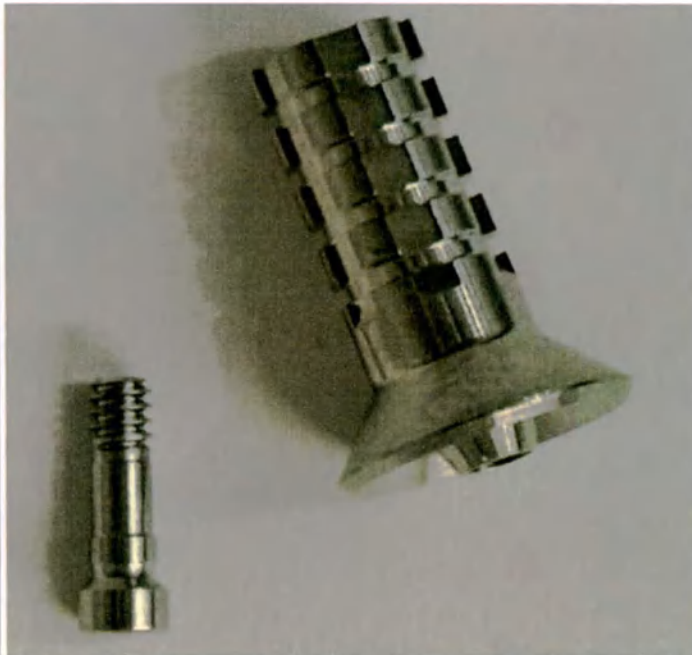
Абатмент временный, для моста, WT, высота 10.3 мм, с винтом
