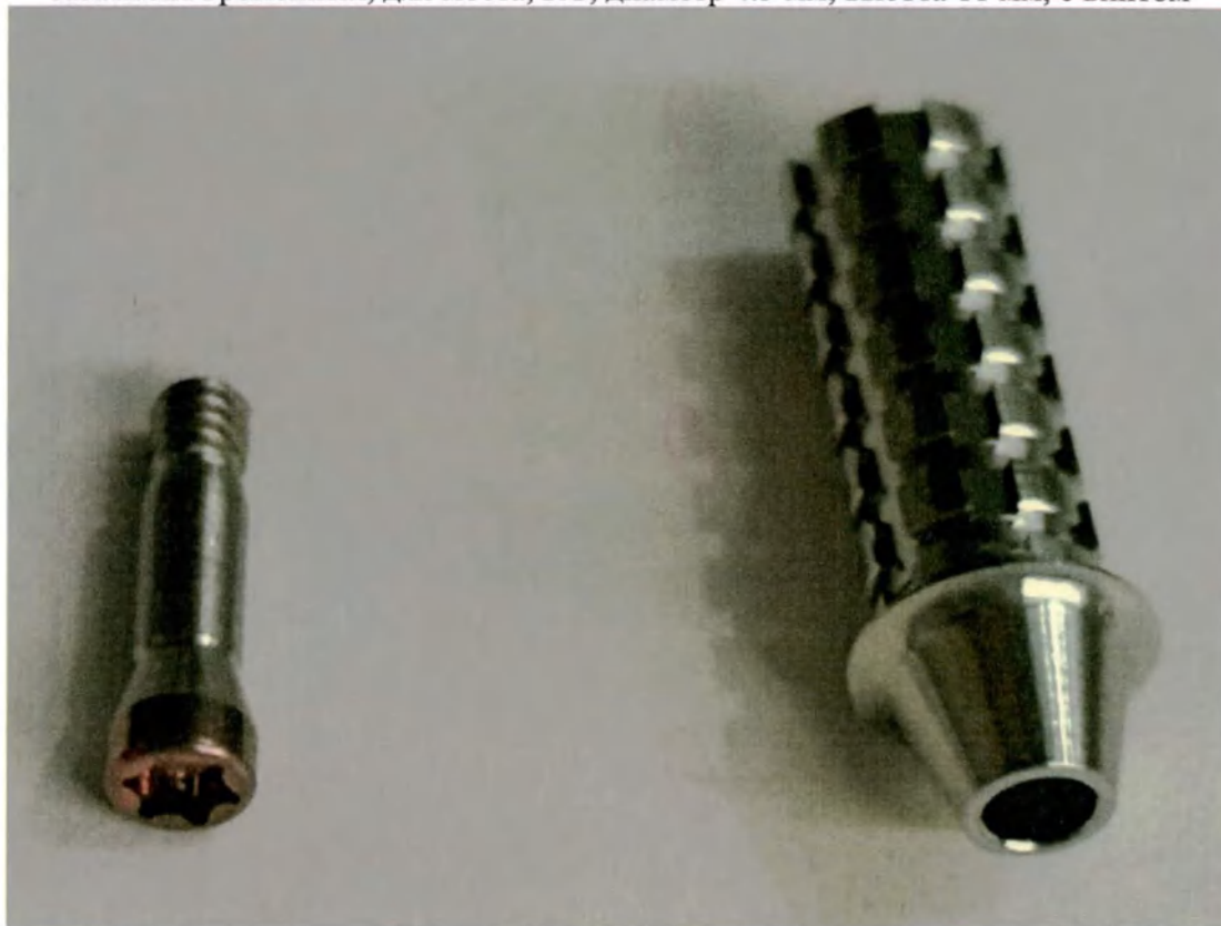
Абатмент SynOcta временный, для коронки, RN, высота 9 мм, с винтом
