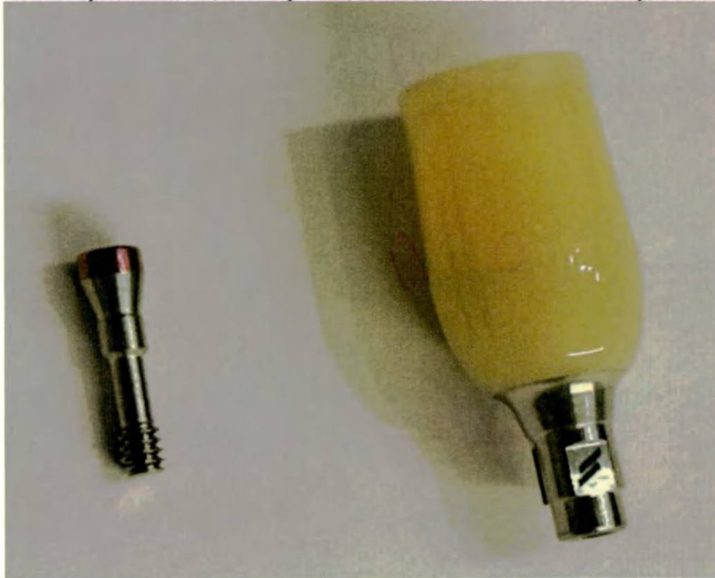
Абатмент временный RC, диаметр 7 мм, высота 12 мм, VITA CAD-Темп, с винтом
