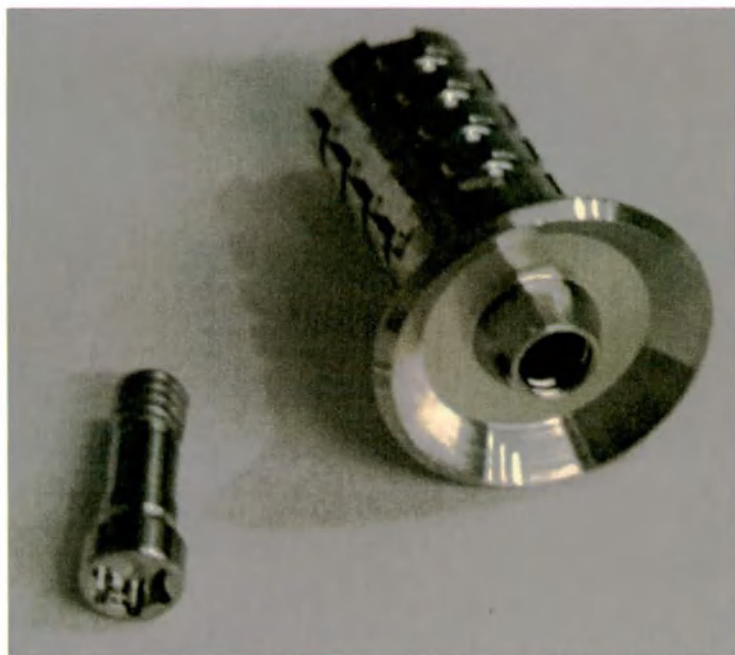
Абатмент временный, для моста, WT, высота 10.3 мм, с винтом
