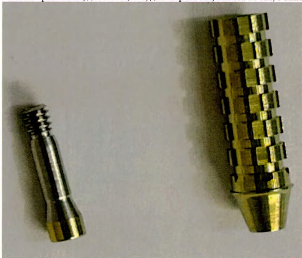
Абатмент временный, для коронки, RC, диаметр 4.5 мм, высота 11 мм, с винтом
