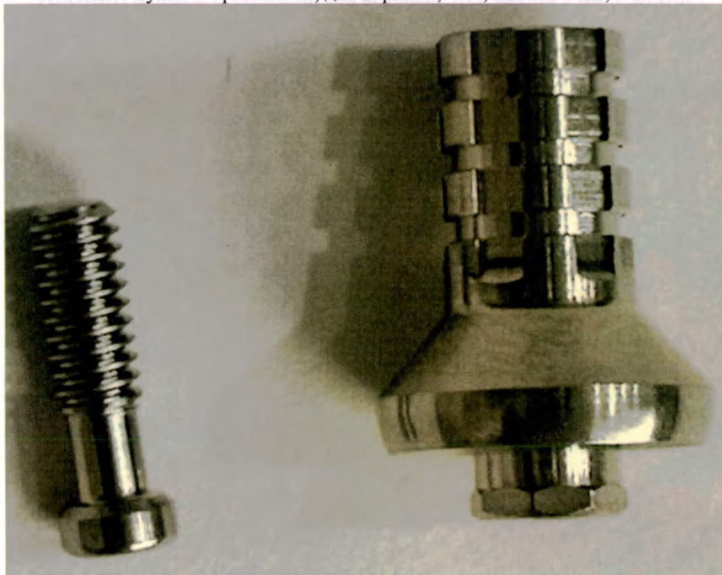
Абатмент SynOcta временный, для коронки, WN, высота 9 мм, с винтом
