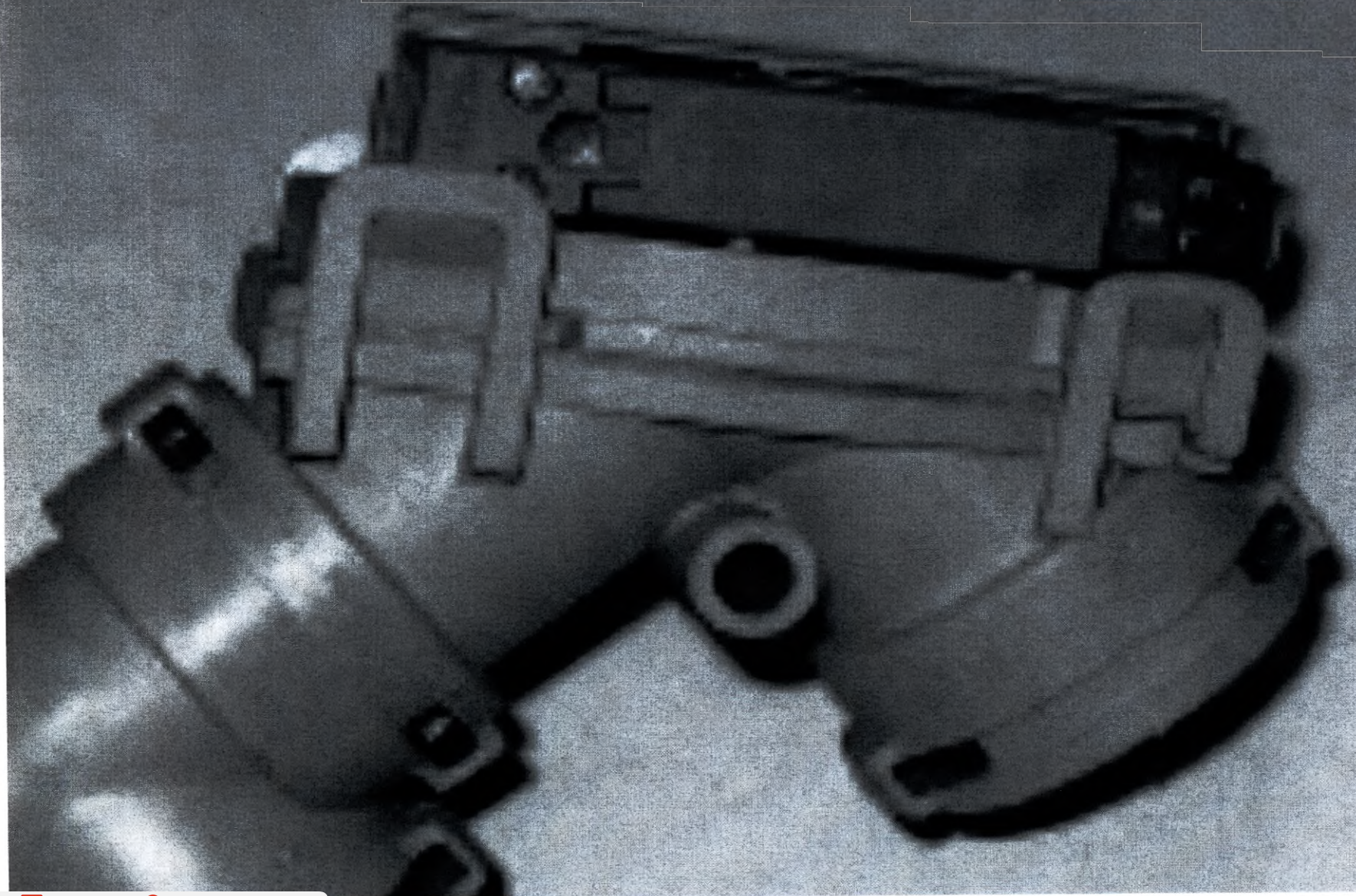
Клапан пневматический для системы влажного типа
