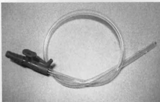
Катетер аспирационный
