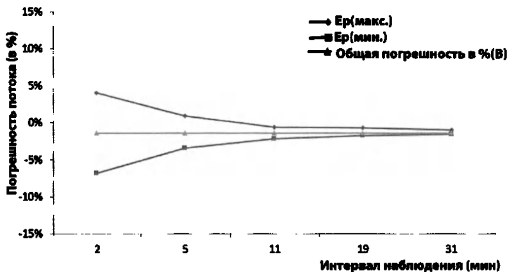
Воронкообразная кривая при скорости 25 мл/ч (последний час)
