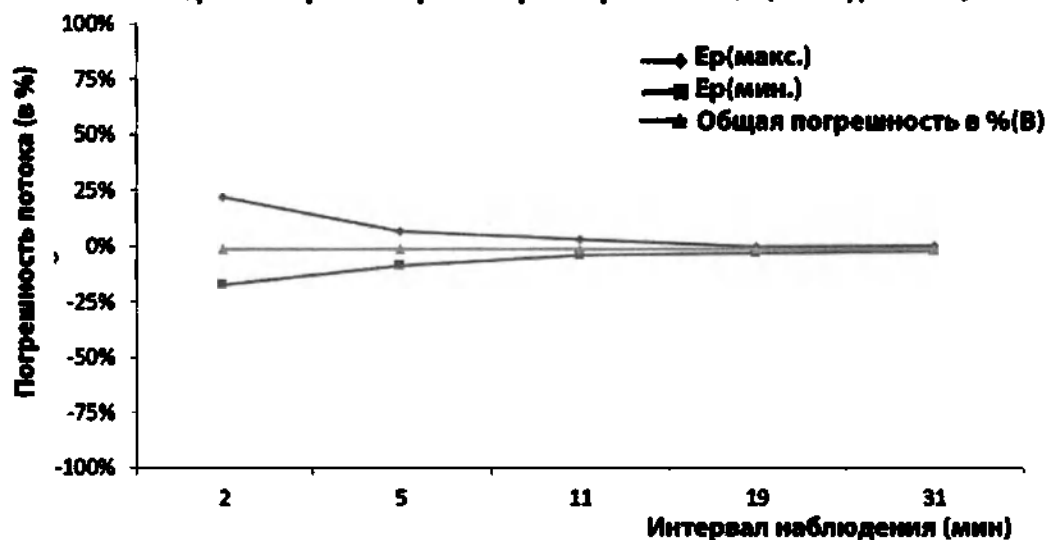
Воронкообразная кривая при скорости 1 мл/ч (последний час)
