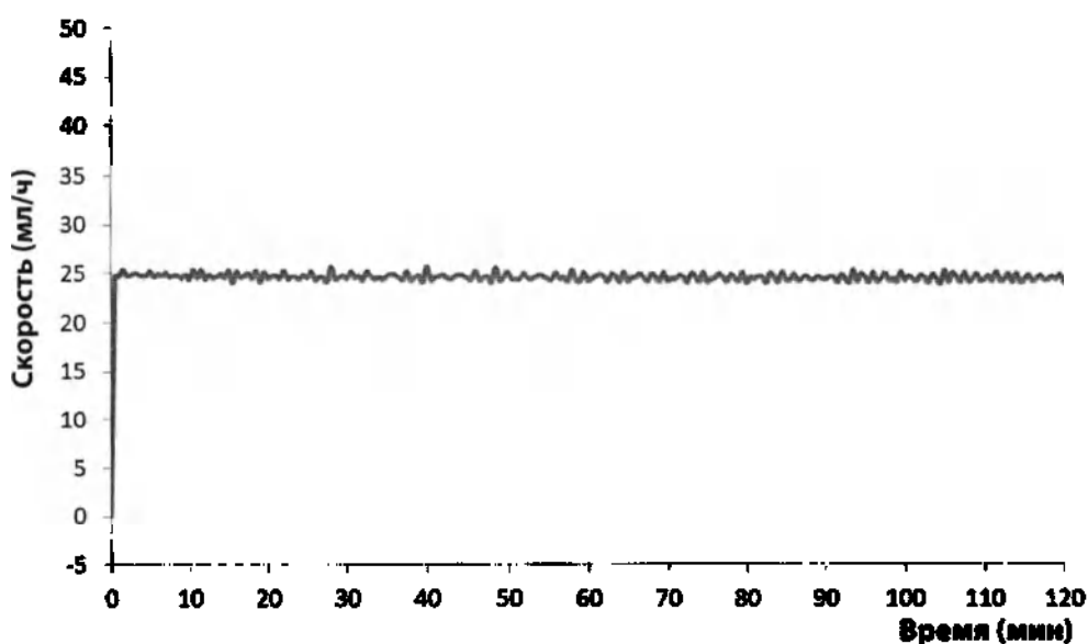
График инфузии при скорости 25 мл/ч в первые 2 часа после запуска
