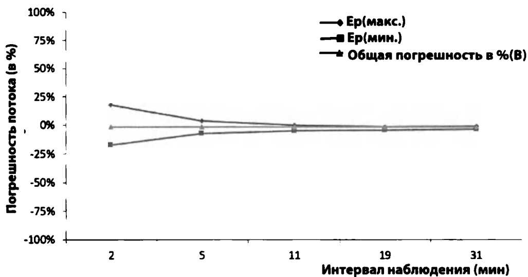
Воронкообразная кривая при скорости 1 мл/ч (последний час)
