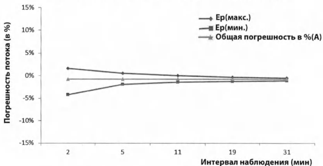
Воронкообразная кривая при скорости 25 мл/ч (последний час)
