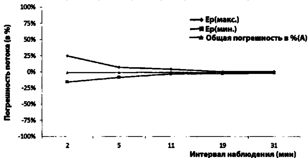
Воронкообразная кривая при скорости 1 мл/ч (второй час)
