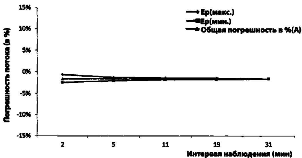
Воронкообразная кривая при скорости 25 мл/ч (второй час)
