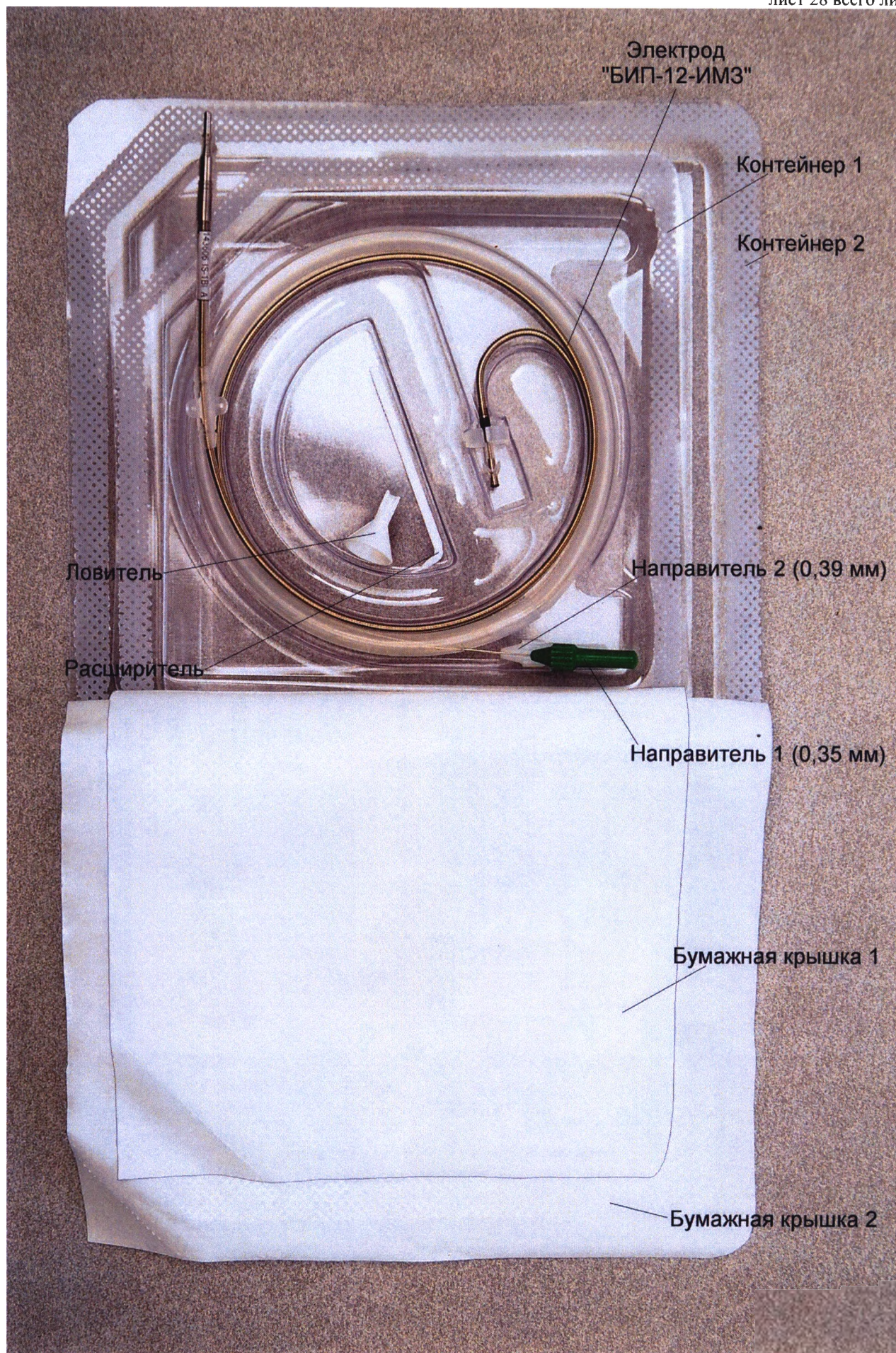
Электрод "БИП-12-ИМЗ" с принадлежностями в стерильной упаковке (упаковка вскрыта)
