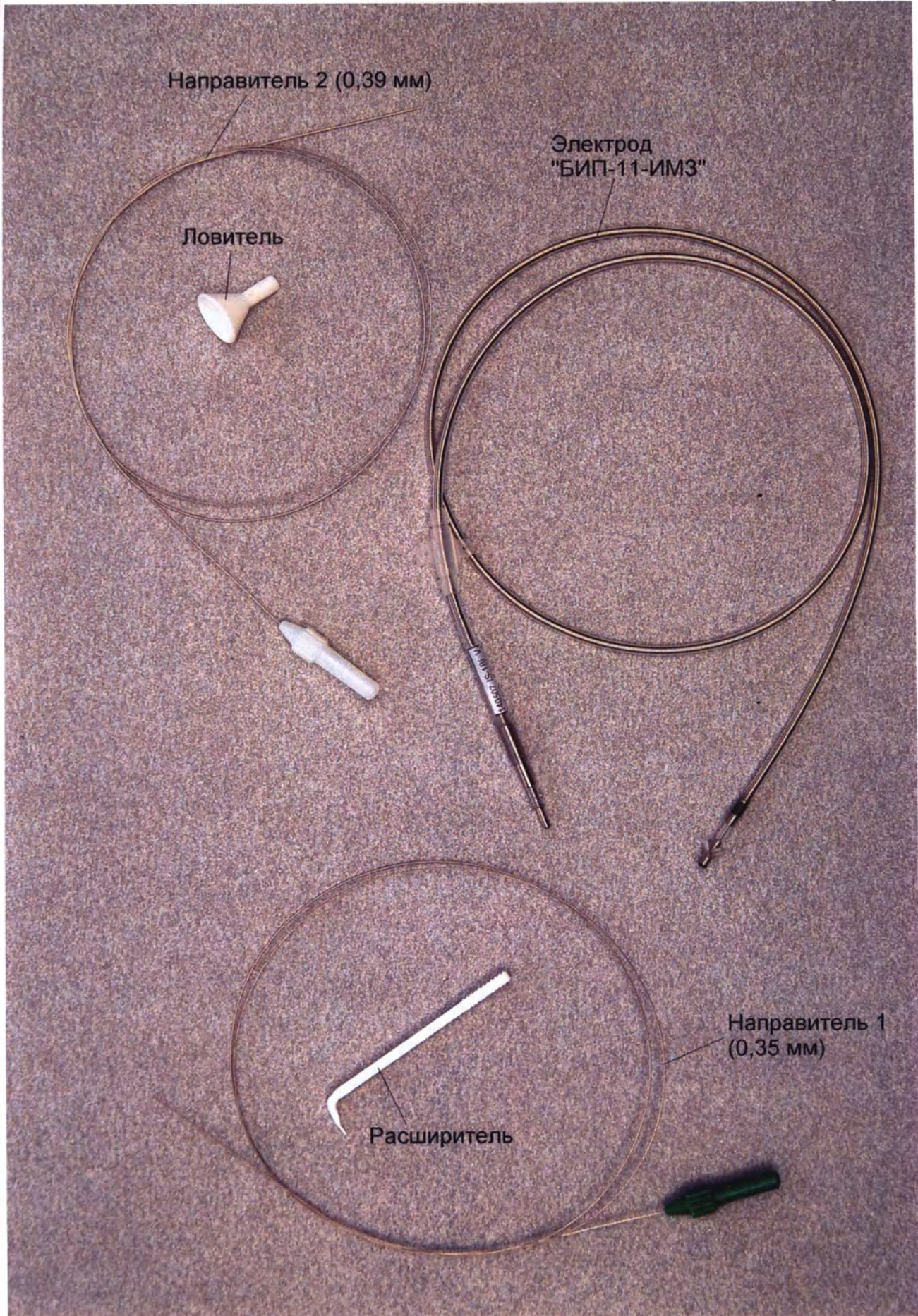
Электрод эндокардиальный постоянный биполярный "БМП-11-ИМЗ" для имплантируемых электрокардиостимуляторов с принадлежностями
