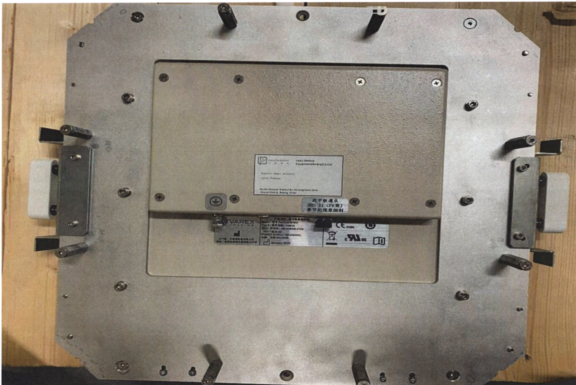
Фотография 98 – Блок датчика серии PaxScan, Varex Imaging (в условиях эксплуатации приемник закрыт кожухом штатива). Вариант внешнего вида
