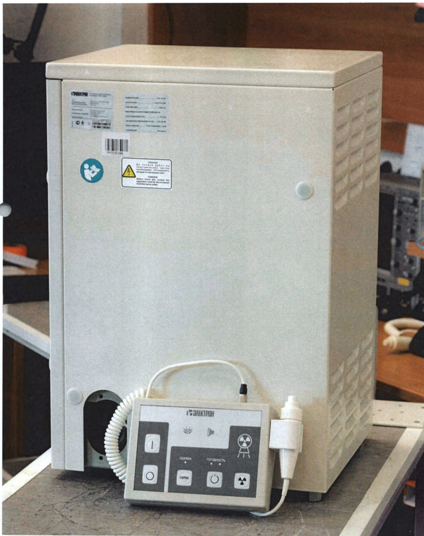
Фотография 75 – Генератор рентгеновский XRPS-10-6380 по спецификации АО «НИПК «Электрон» с пультом управления. Вариант внешнего вида
