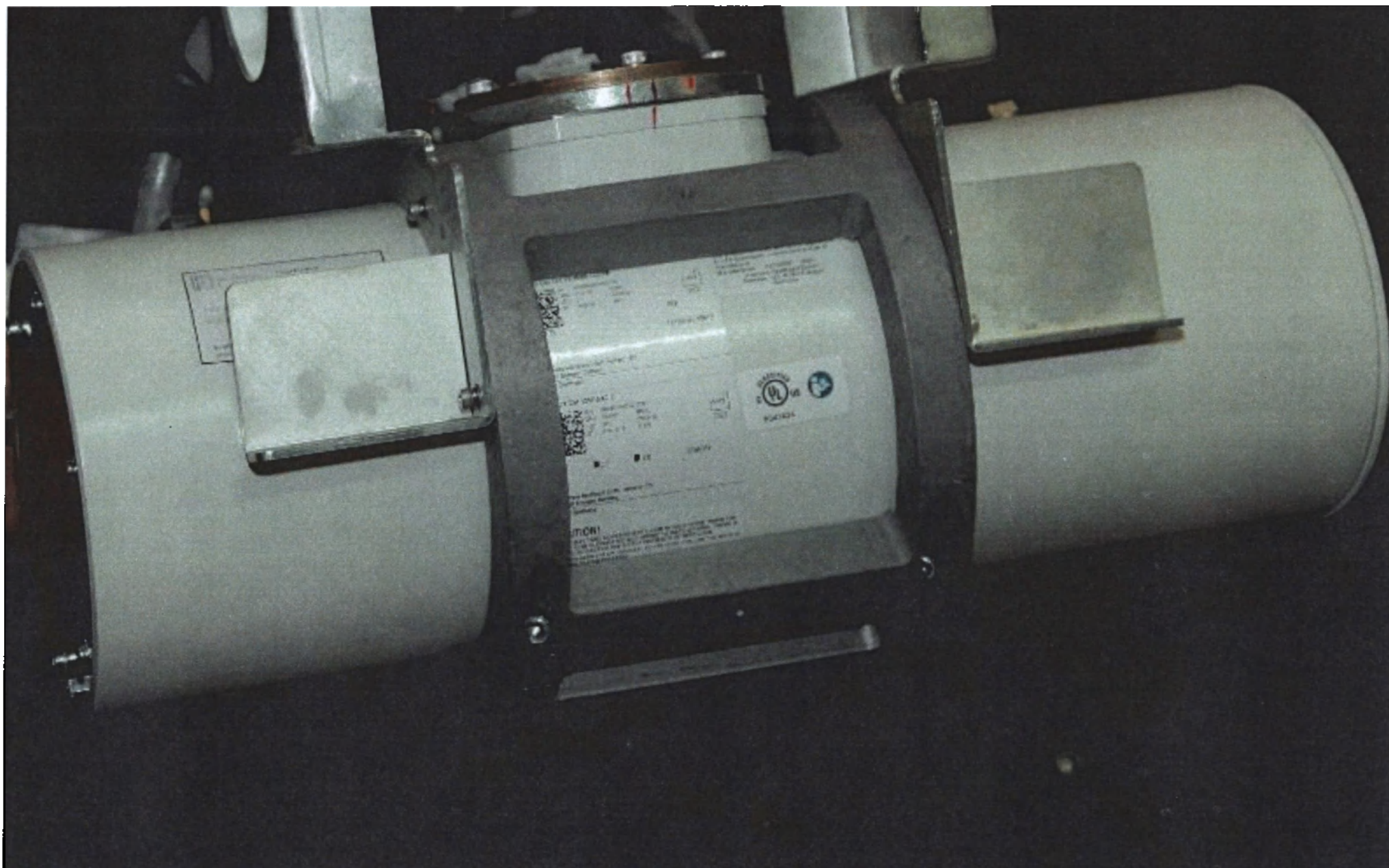
Фотография 30 – Излучатель рентгеновский MegaLix Cat, Siemens Healthcare GmbH (в условиях эксплуатации излучатель закрыт кожухом штатива). Вариант внешнего вида
