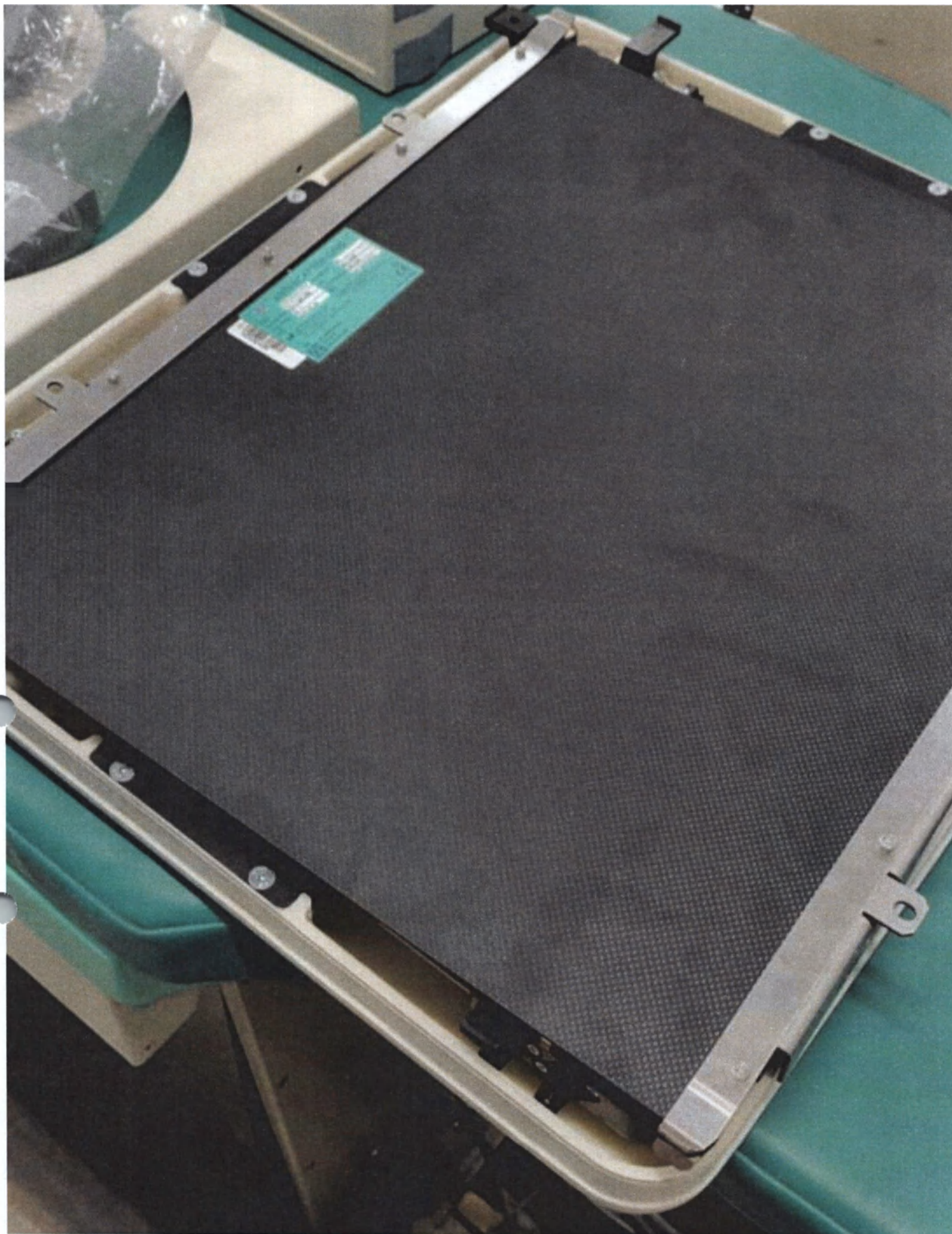
Фотография 20 – Решетка фокусирующая (растр рентгеновский) серии JPI GRID Jungwon Precision Ind. Co., Ltd и место нанесения маркировки (в условиях эксплуатации растр закрыт кожухом штатива). Вариант внешнего вида
