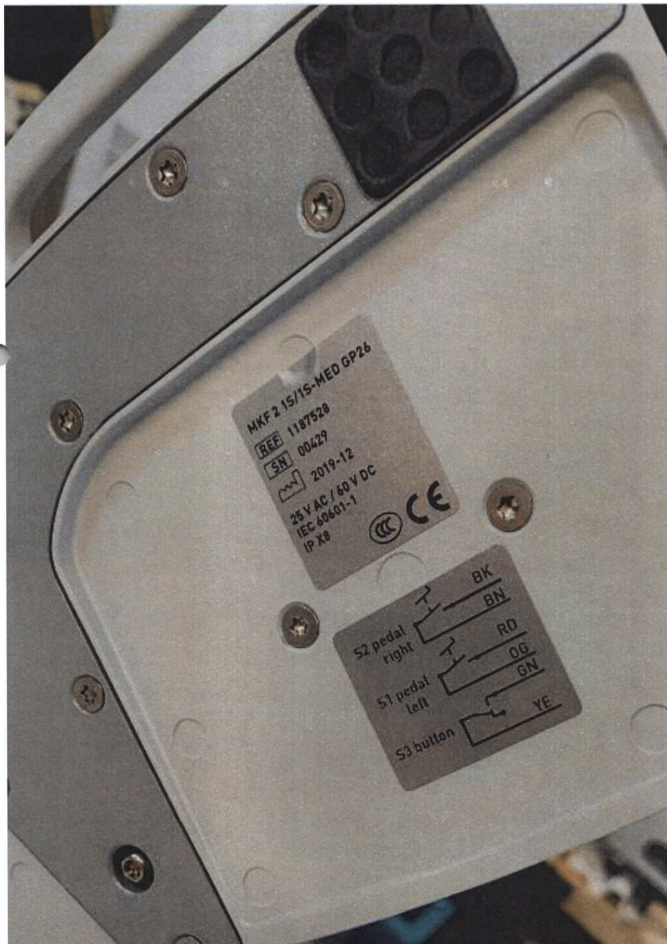
Фотография 14 – Выключатель педальный серии MKF, Lery Medical Equipment (Beijing) Co., Ltd. Образец внешнего вида варианта маркировки
