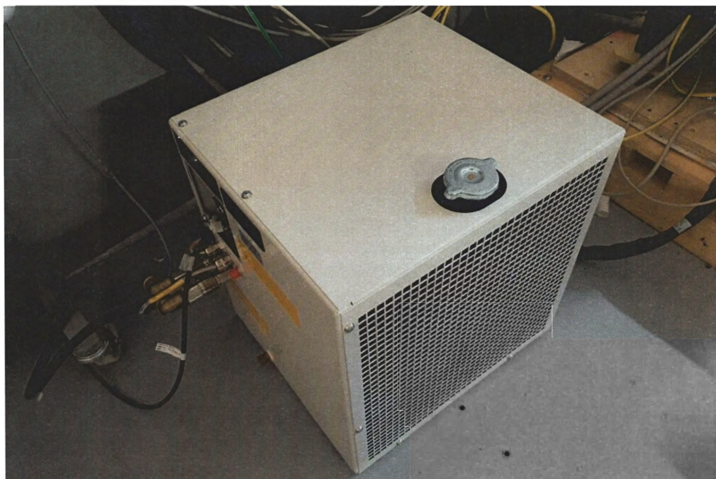
Фотография 32 – Система охлаждения излучателя рентгеновского WL 3000 SU, Siemens Healthcare GmbH (в составе рентгеновского излучателя Siemens Healthcare). Вариант внешнего вида
