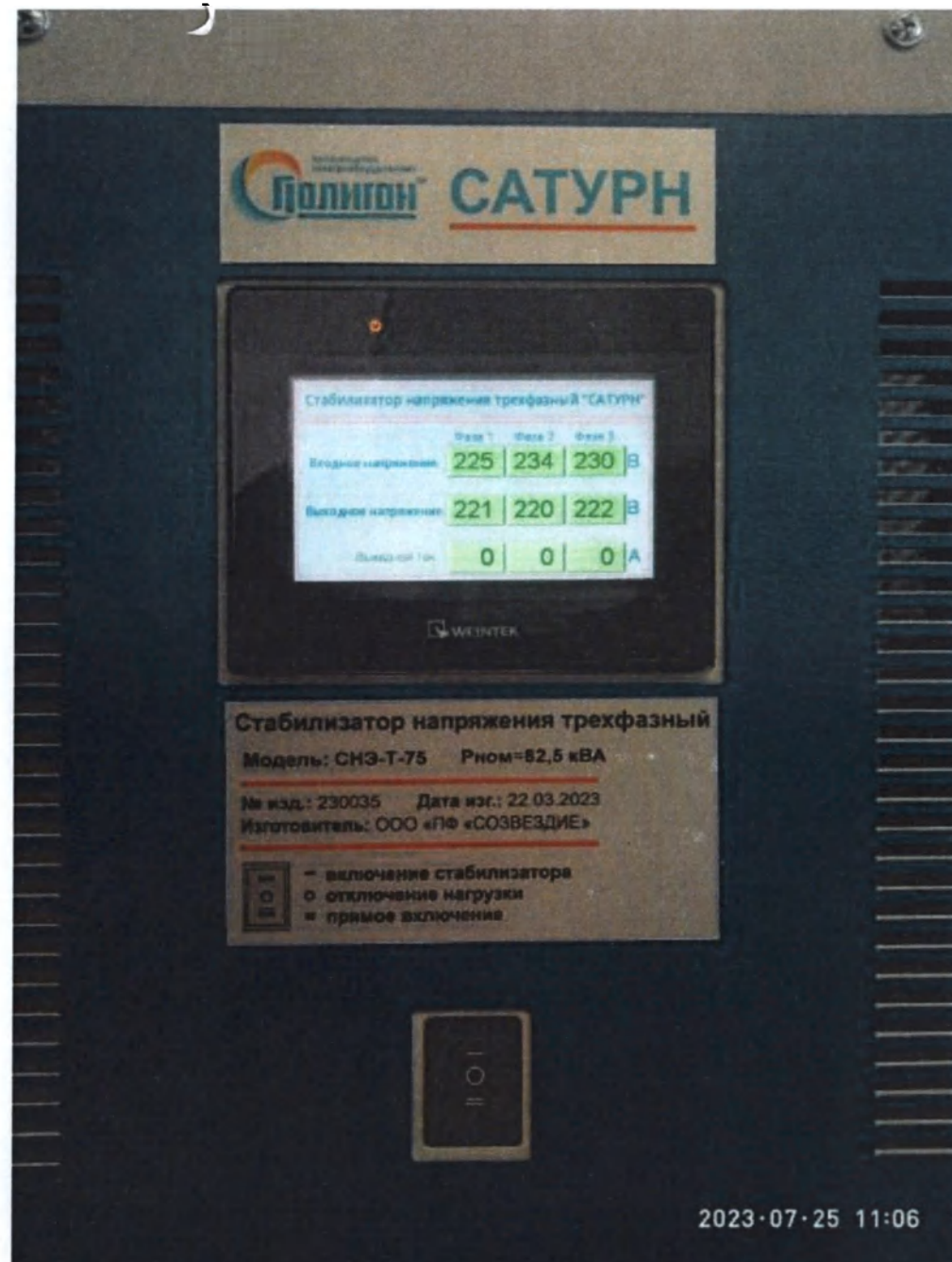
Фотография 153 – Стабилизатор серии СНЗ (вариант внешнего вида) в составе спецификации АРМ WST1-00, АО «НИПК «Электрон»
