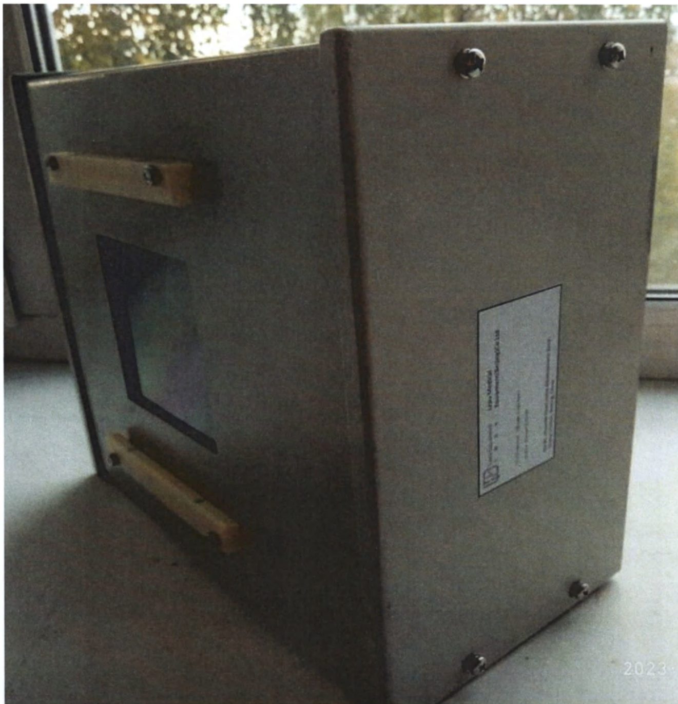
Фотография 47 – Коллиматор (диафрагма) серии Vicor-LD100, Lepu Medical Equipment (Beijing) Co., Ltd (при эксплуатации коллиматор закрыт кожухом штатива). Вариант внешнего вида и место нанесения маркировки
