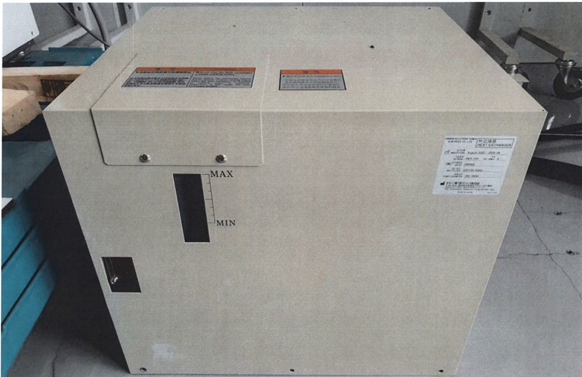
Фотография 26 – Система охлаждения излучателя рентгеновского HEX-125 Canon Electron Tubes & Devices Co., Ltd (в составе излучателя Canon). Вариант внешнего вида
