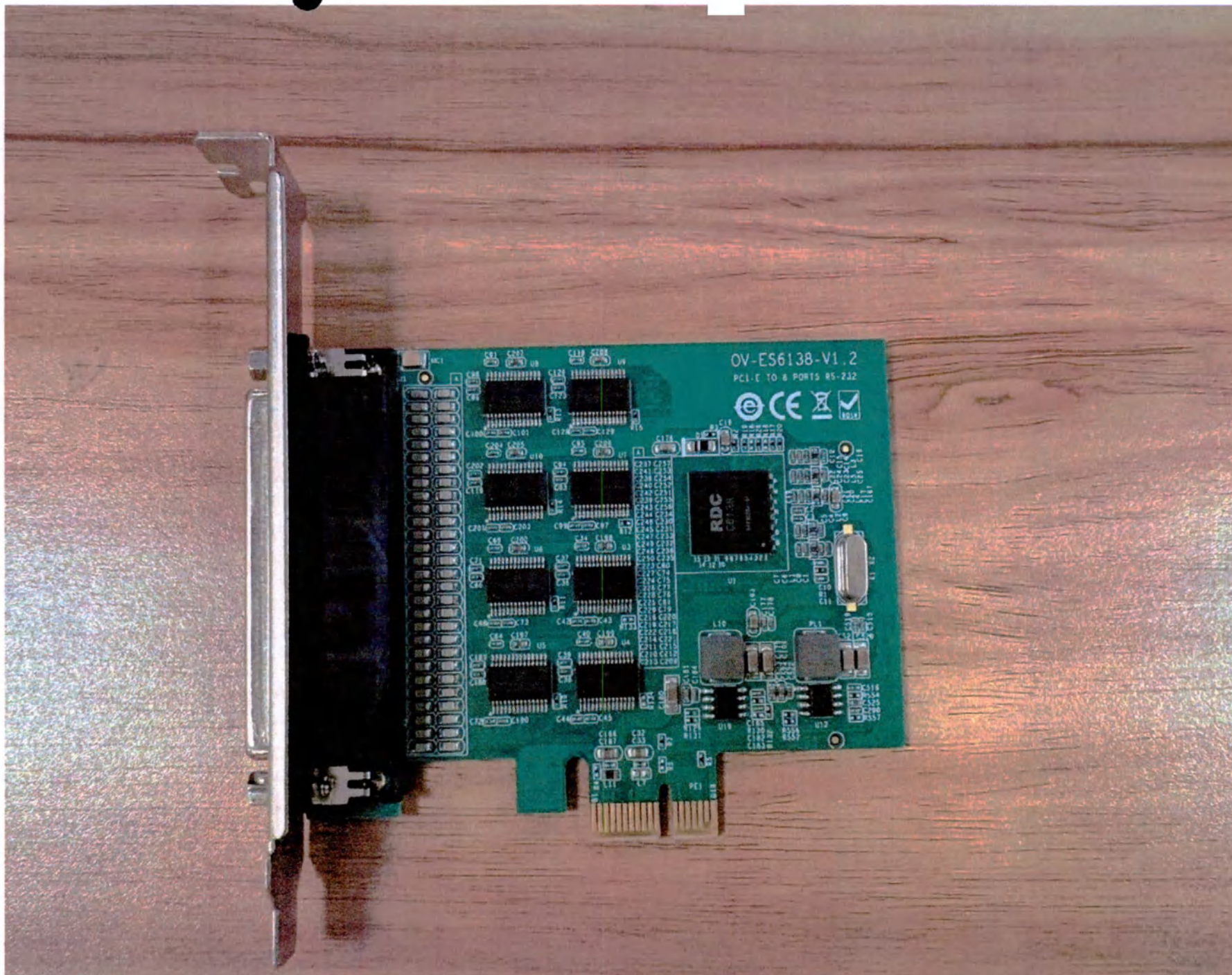
Набор компьютерных комплектующих №2: Плата расширения 1 в 8 (Контроллер)
