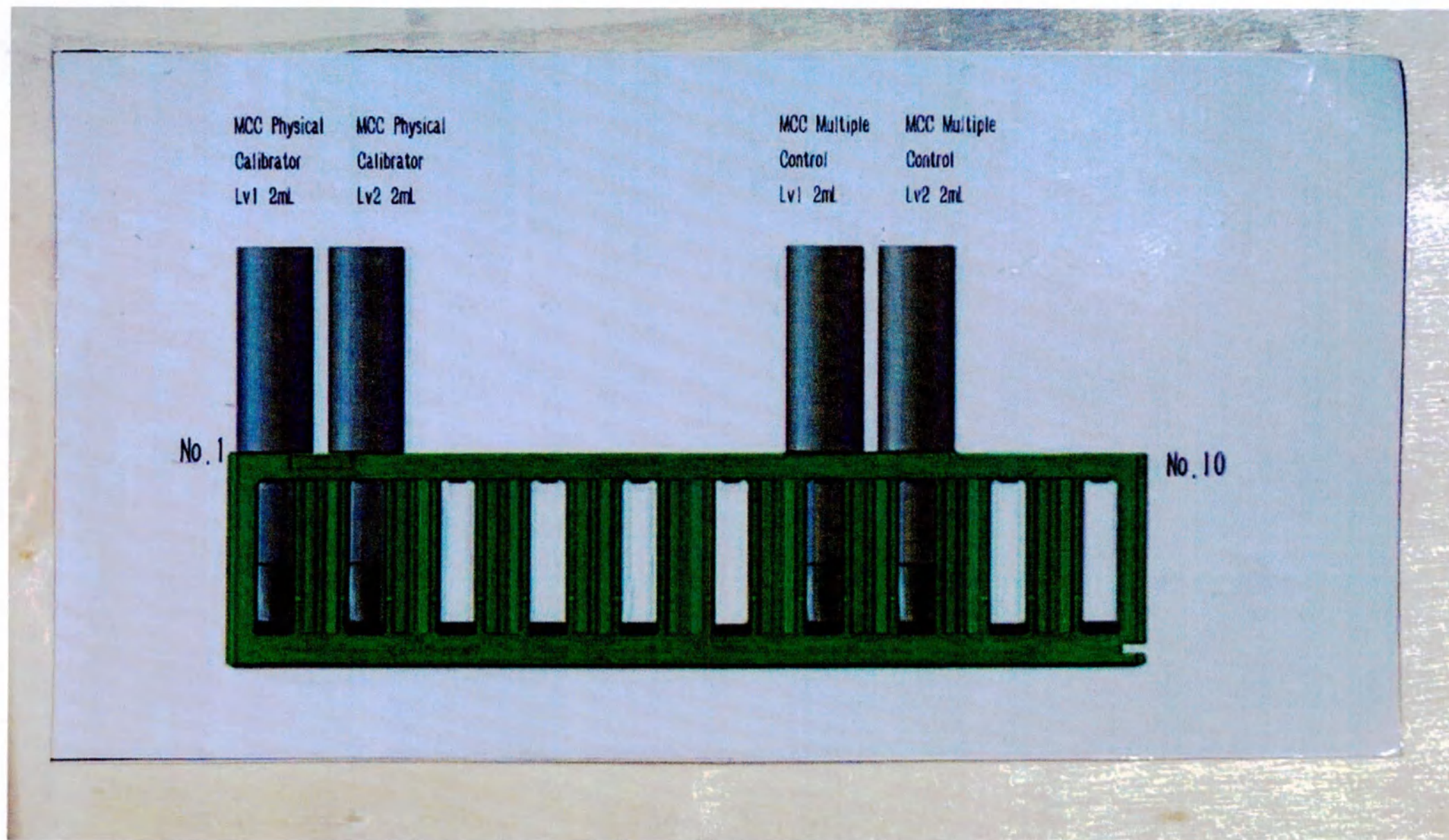
Схема загрузки штатива для контроля и калибровки СА-500
