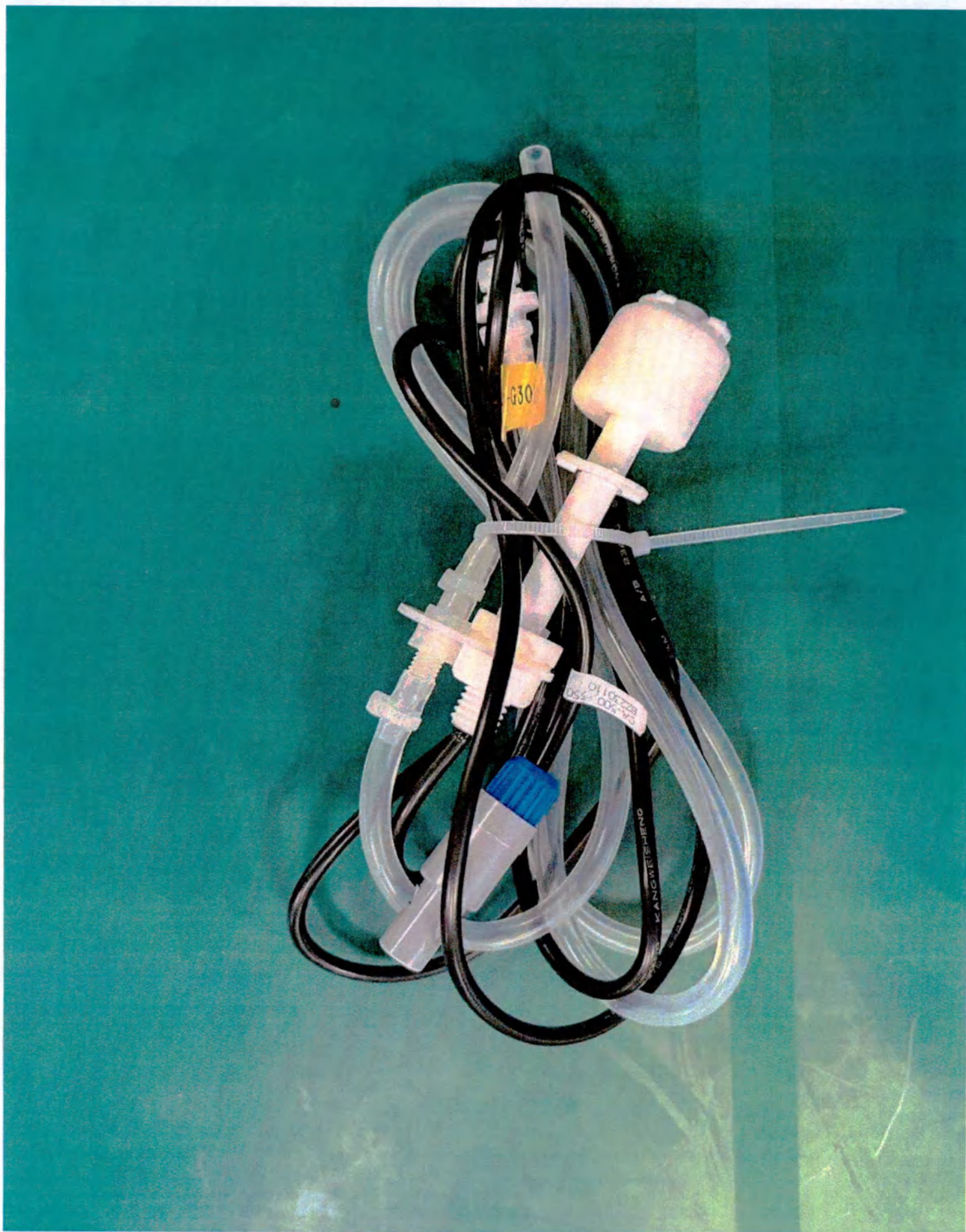
Трубка для слива отработанной жидкости с датчиком
