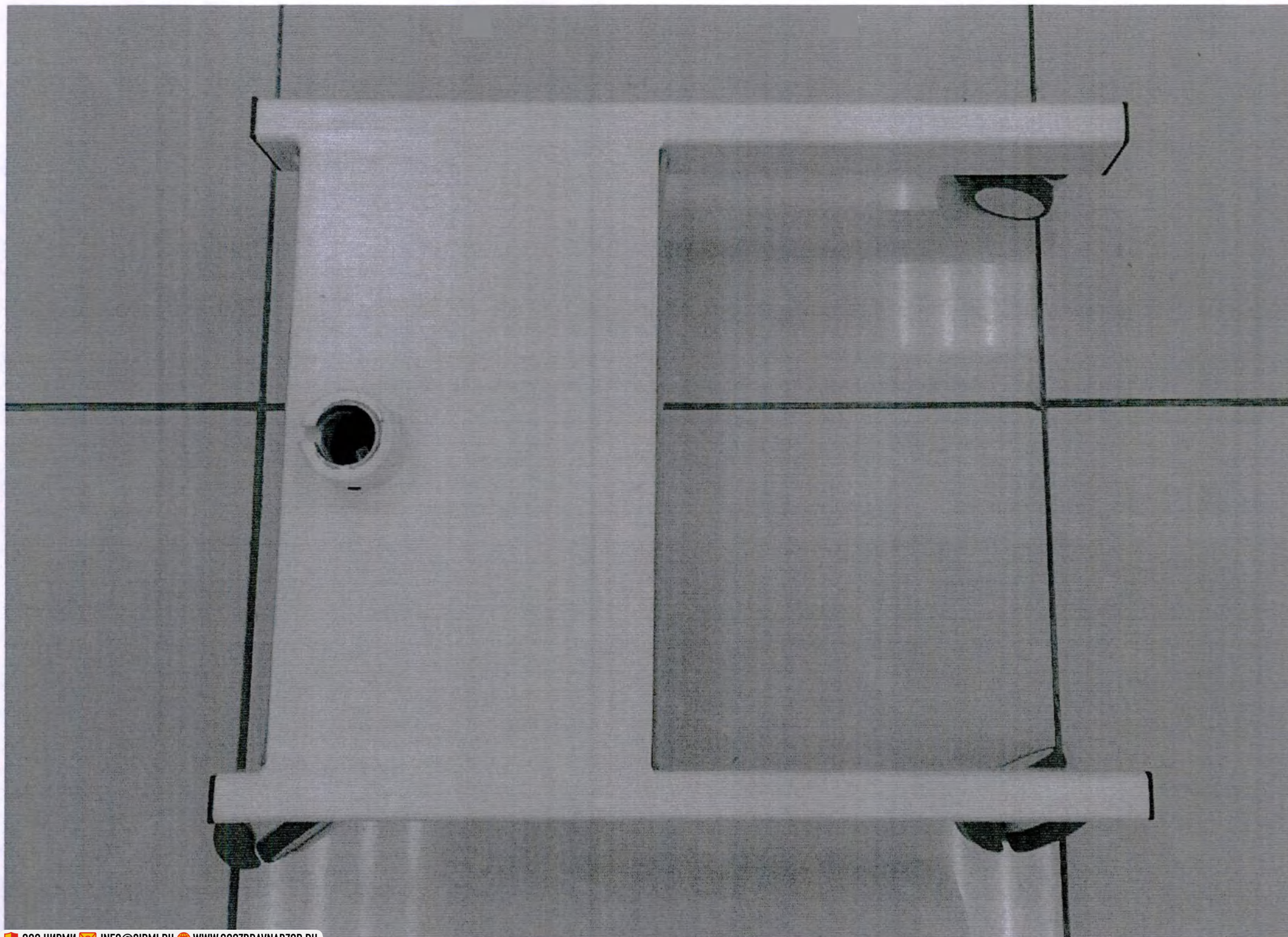
Рис. 6 – Основание с колесами
