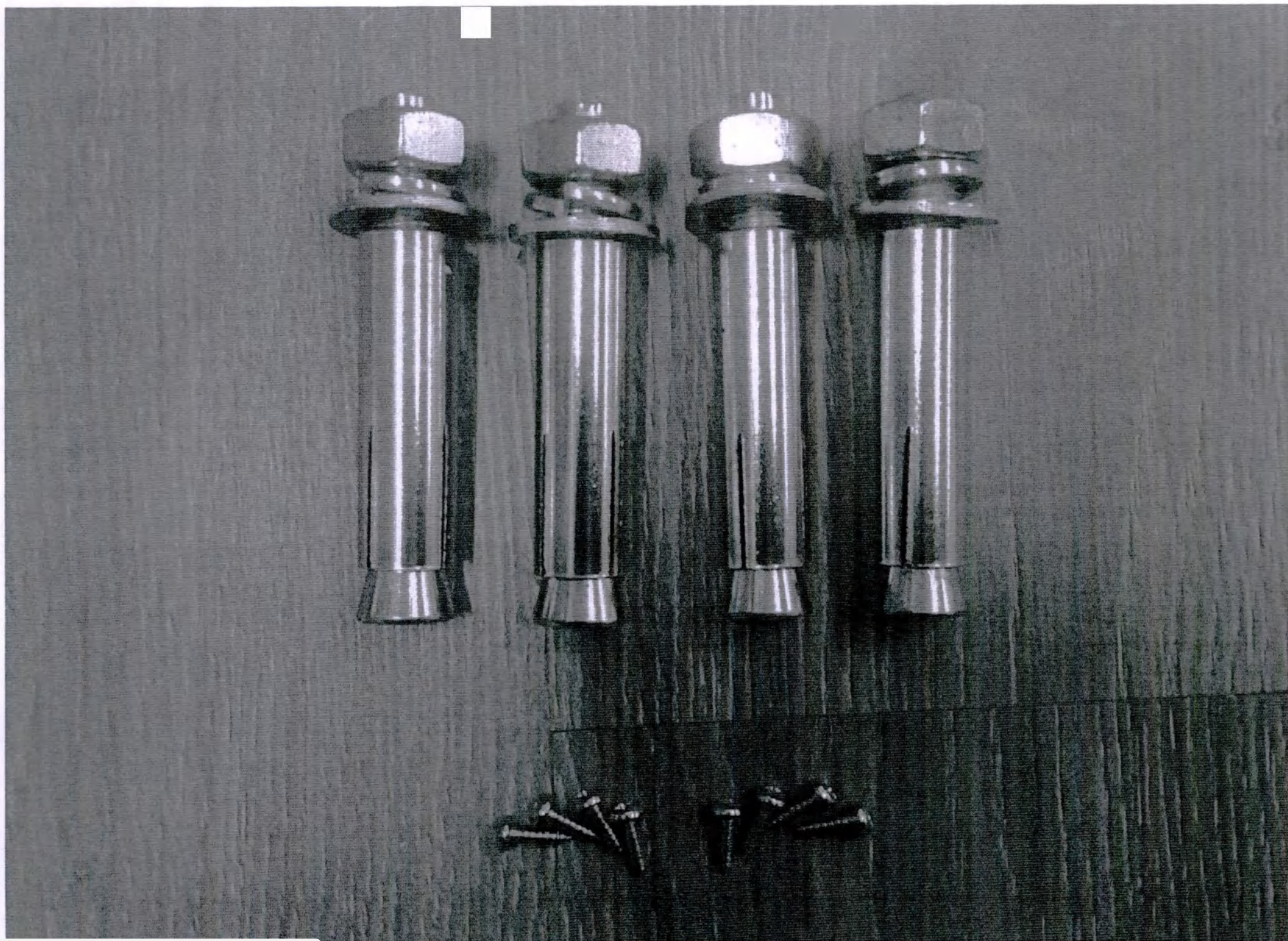
Рис. 44 – Комплект крепежа
