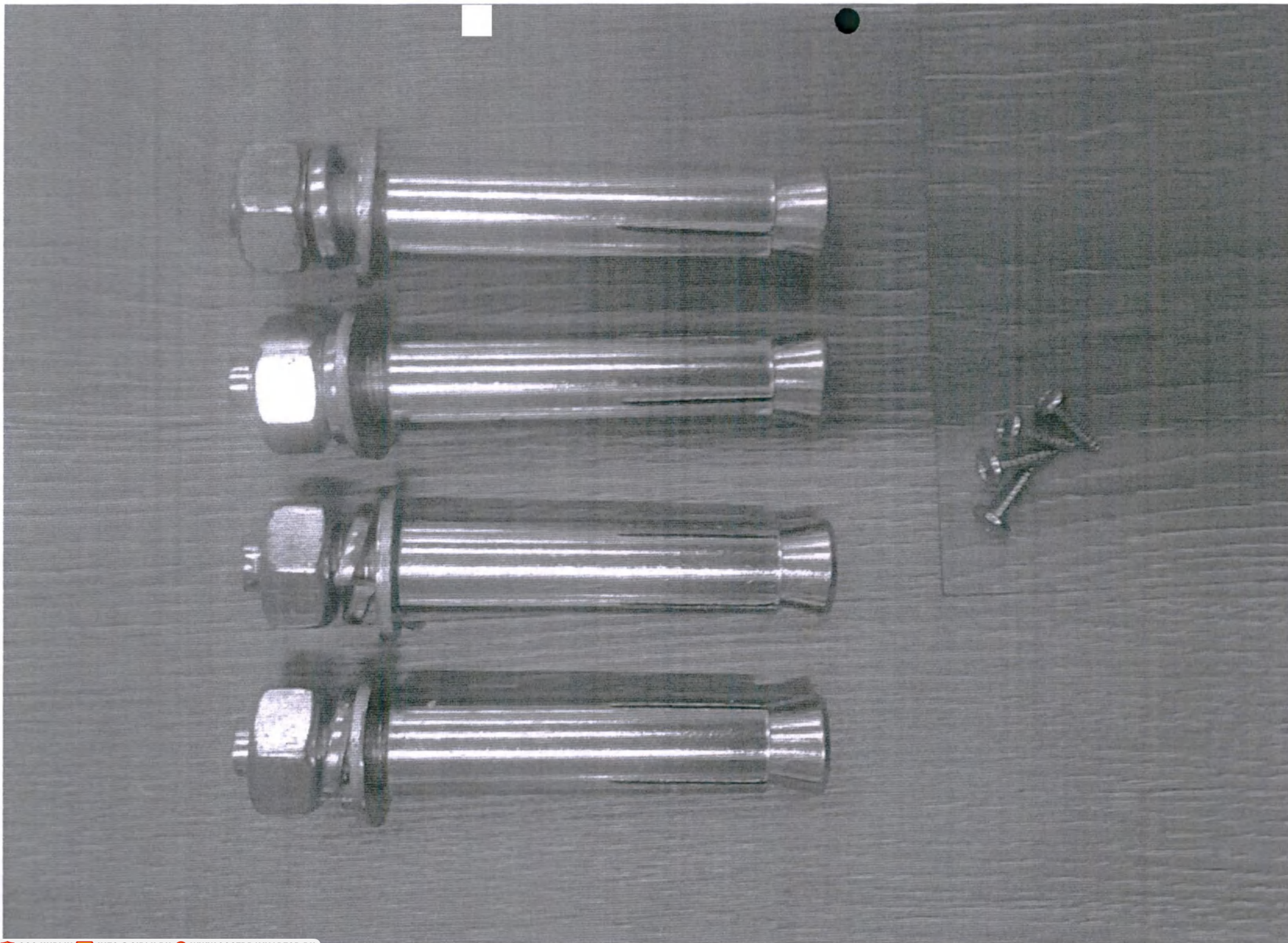
Рис. 22 – Комплект крепежа
