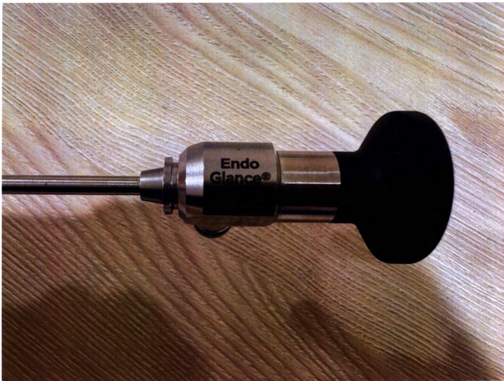
Фото 3. Внешний вид вариантов исполнений: Цистоскоп EndoGlance®, диаметр 4 мм, длина 302 мм, угол 0°, Цистоскоп EndoGlance®, диаметр 2.7 мм, длина 302 мм, угол 0°, Цистоскоп EndoGlance®, диаметр 1.9 мм, длина 302 мм, угол 0°
