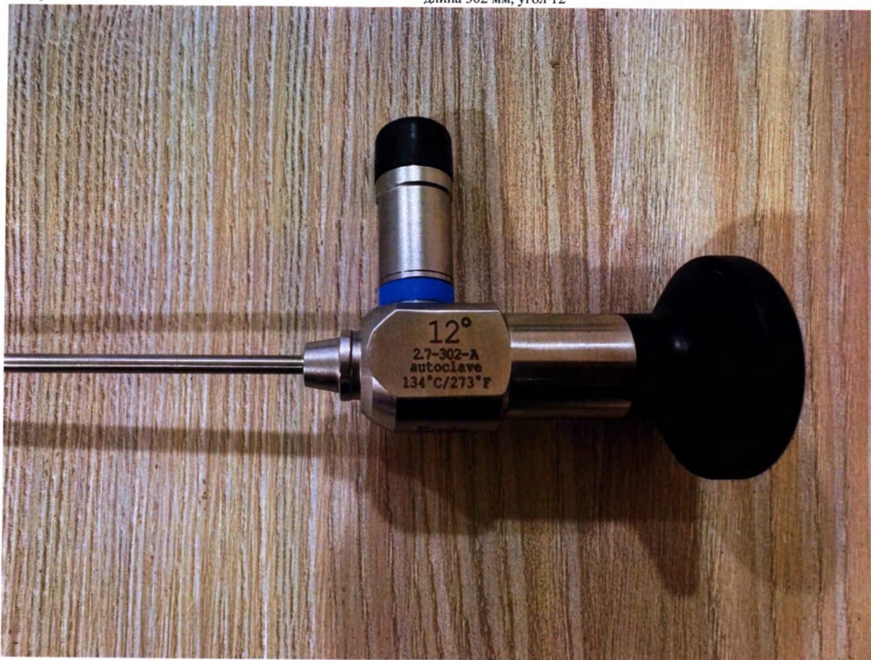
Фото 5. Внешний вид вариантов исполнений: Цистоскоп EndoGlance®, диаметр 4 мм, длина 302 мм, угол 12°, Цистоскоп EndoGlance®, диаметр 2.7 мм, длина 302 мм, угол 12°
