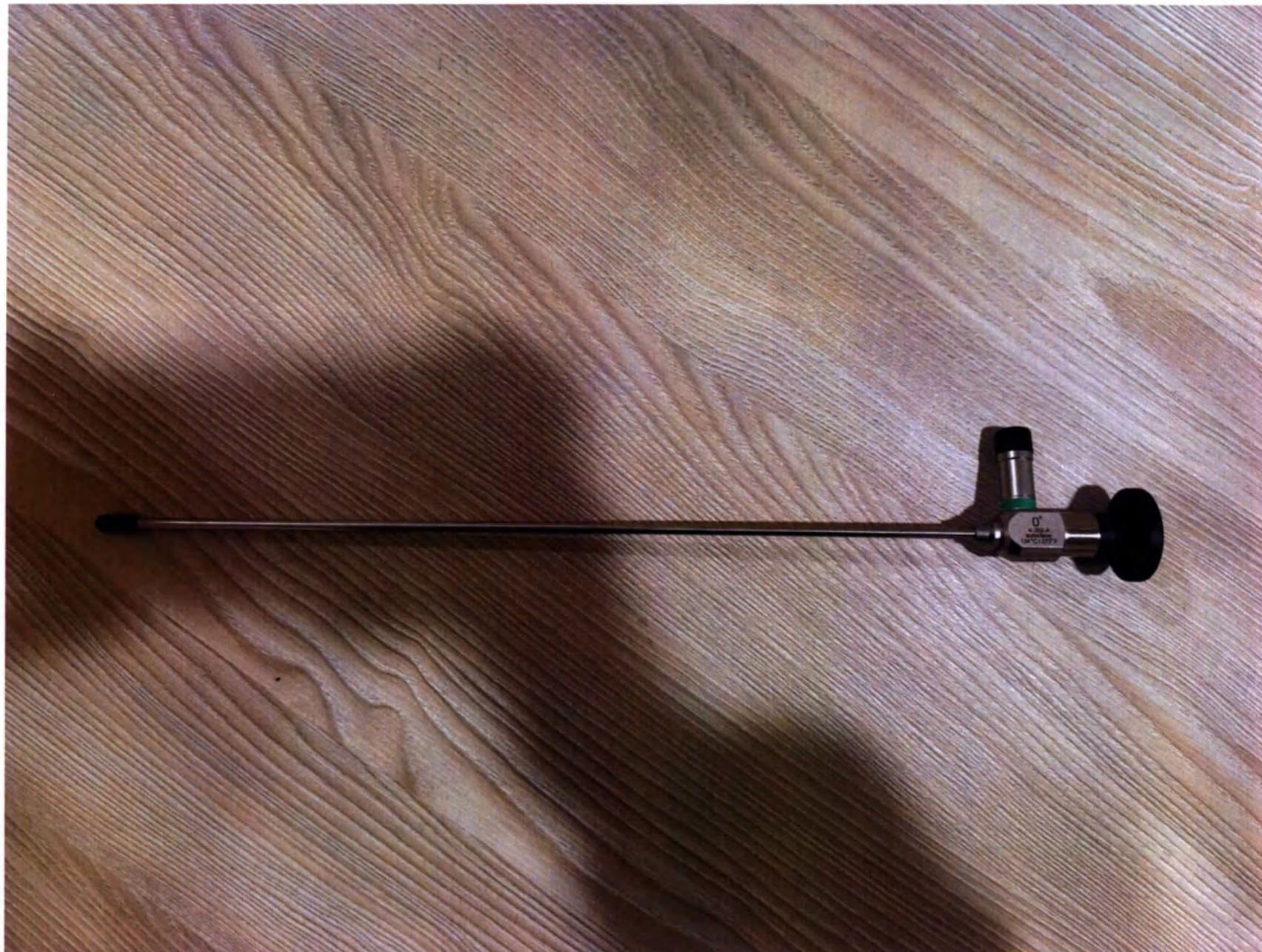
Фото 1. Внешний вид вариантов исполнений: Цистоскоп EndoGlance®, диаметр 4 мм, длина 302 мм, угол 0°, Цистоскоп EndoGlance®, диаметр 2.7 мм, длина 302 мм, угол 0°, Цистоскоп EndoGlance®, диаметр 1.9 мм, длина 302 мм, угол 0°
