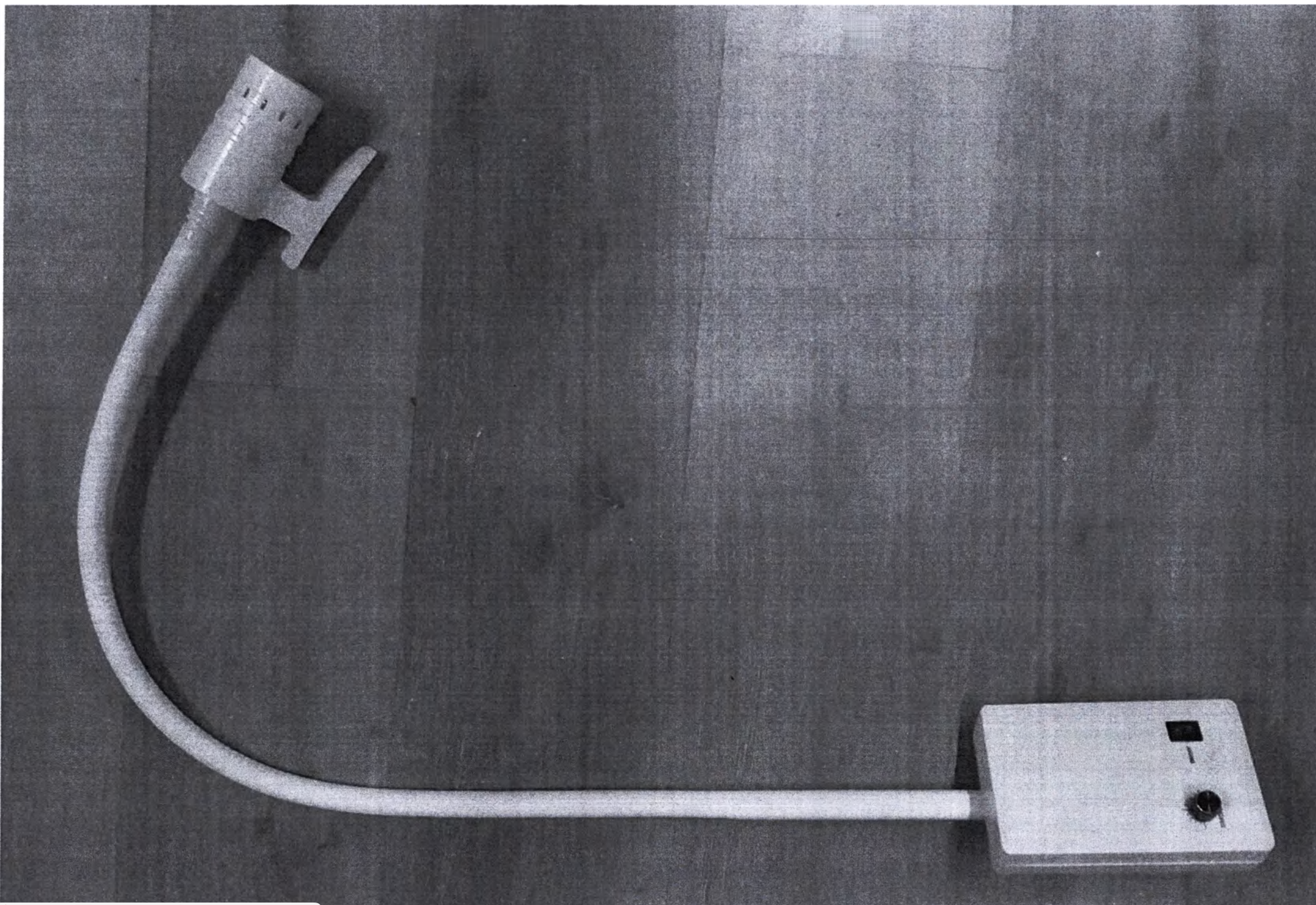
Рис. 2 – Штатив верхний с блоком управления и блоком освещения
