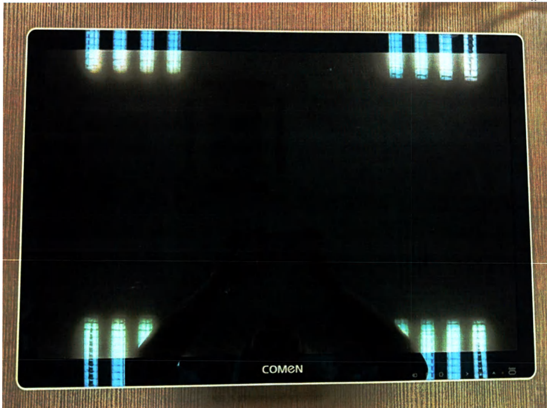
Монитор жидкокристаллический, тип 2 модель S271P (Вид спереди)
