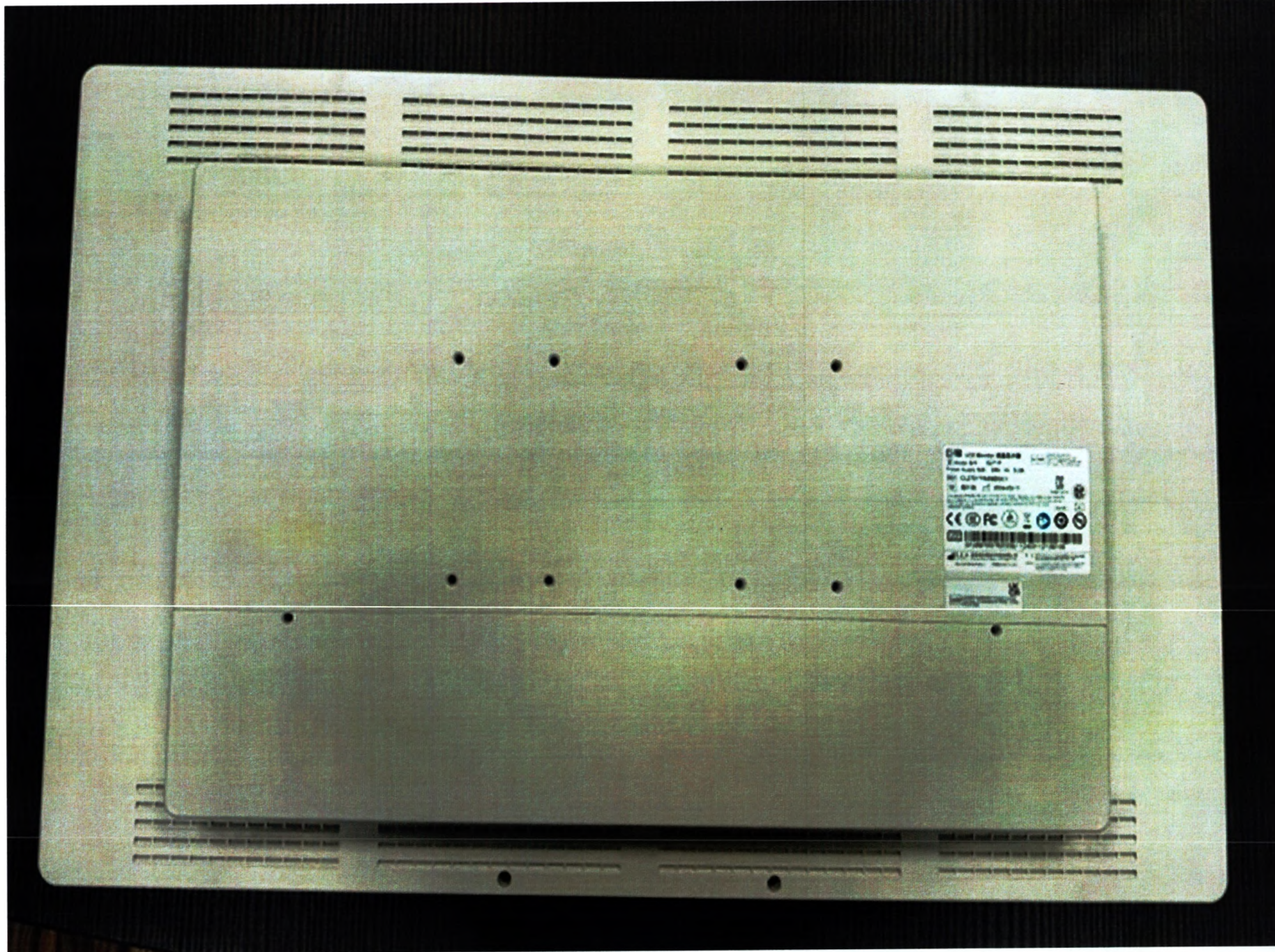
Монитор жидкокристаллический, тип 2 модель S271P (Вид сзади)
