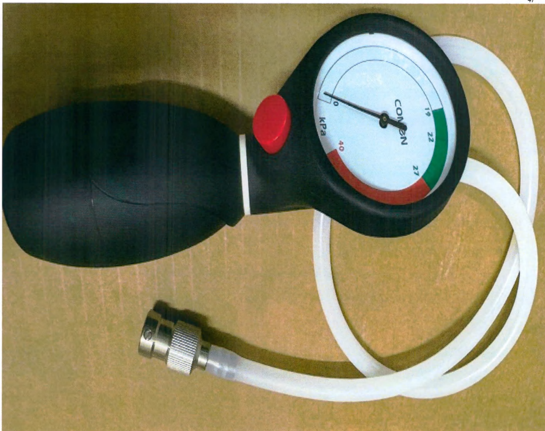
Измеритель утечек LT-001
