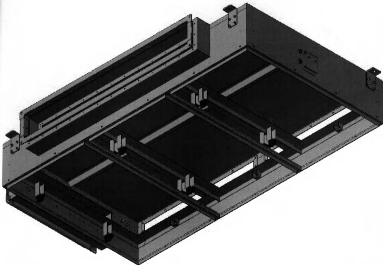
Потолок ламинарный медицинский ЛИТАЭРО по ТУ 32.50.50-007-37247008-2024 в варианте исполнения ЛИТАЭРО 2,0 х 1,8 С. Ячейка ОВП 402.01.01.
