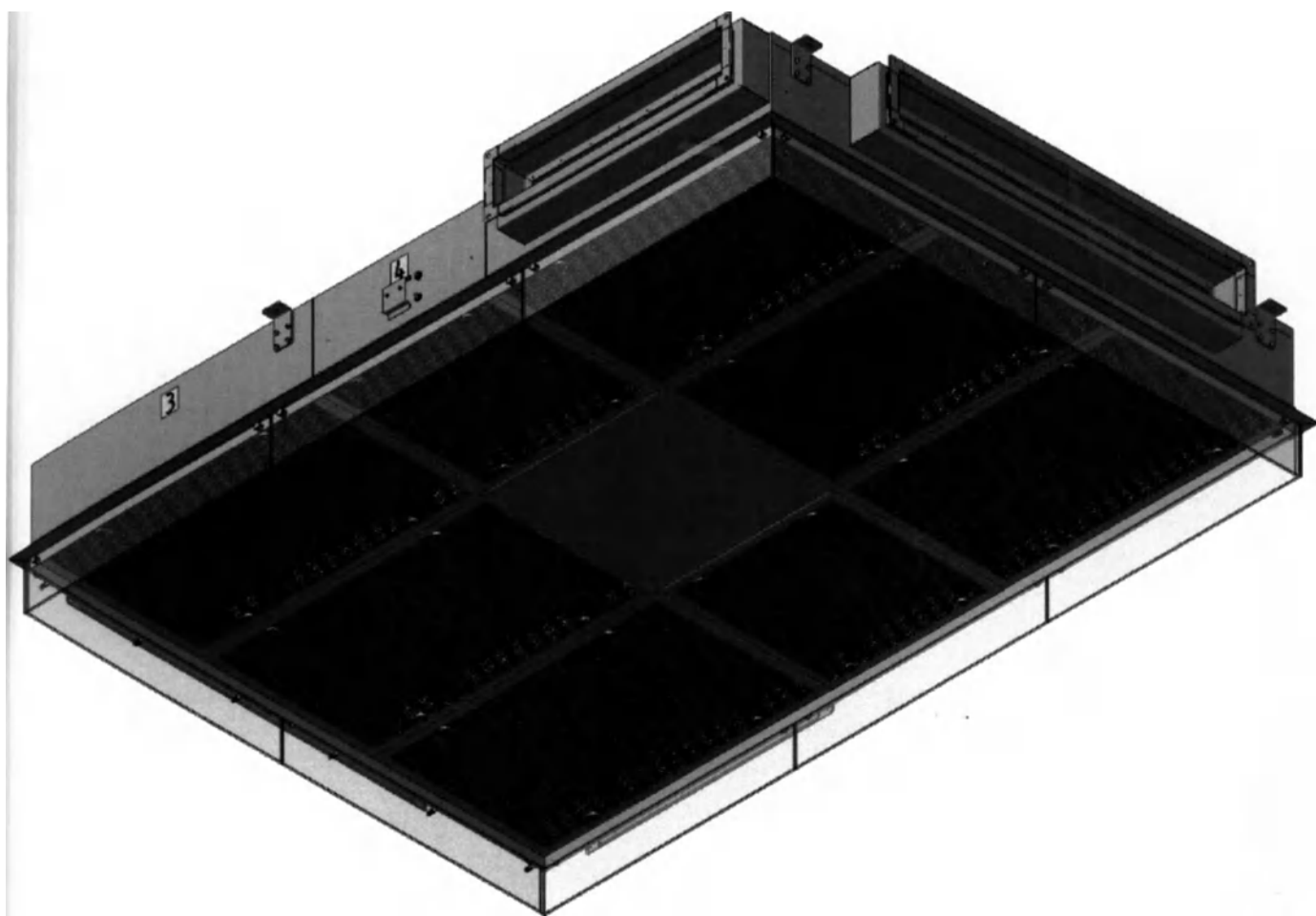
Потолок ламинарный медицинский ЛИТАЭРО по ТУ 32.50.50-007-37247008-2024 в варианте исполнения ЛИТАЭРО 2,6 x 1,8 С. Общий вид изделия
