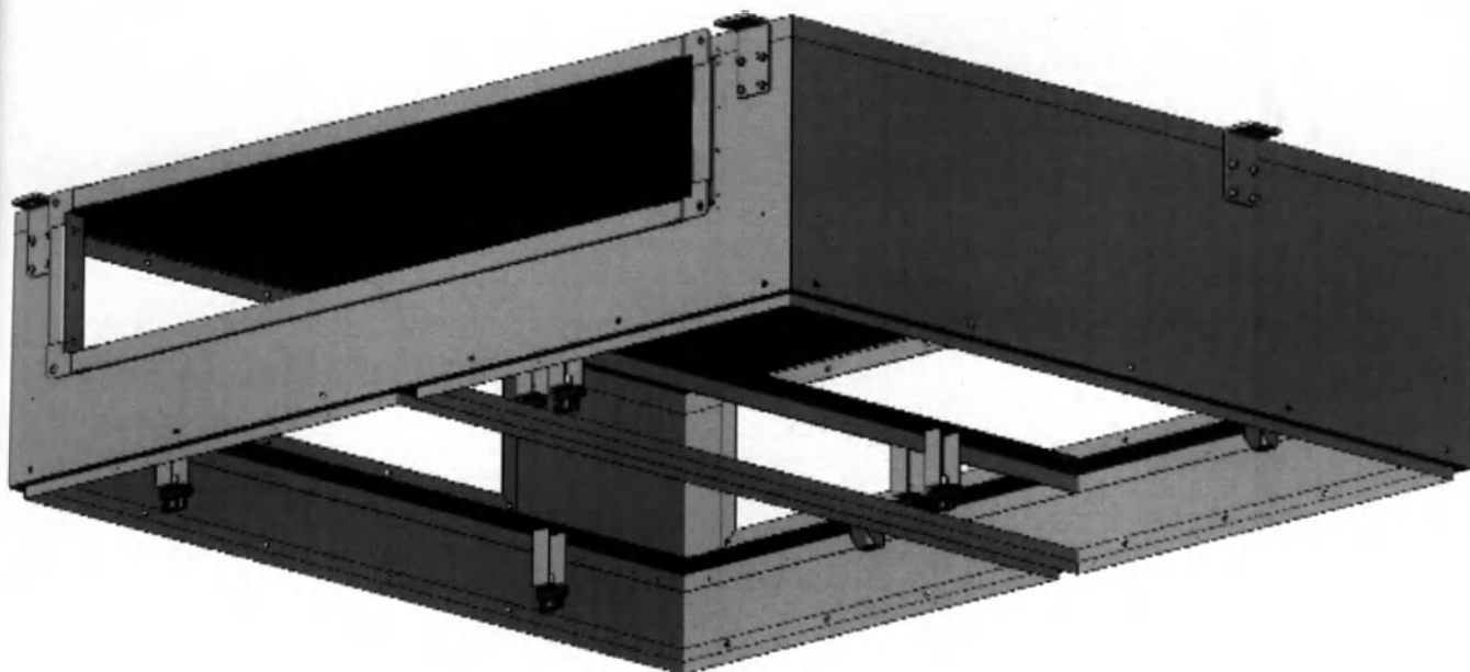
Потолок ламинарный медицинский ЛИТАЭРО по ТУ 32.50.50-007-37247008-2024 в варианте исполнения ЛИТАЭРО 3,6 х 2,6. Ячейка ОВП 383.01.01..
