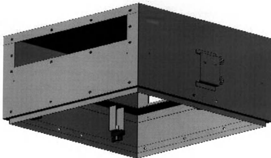
Потолок ламинарный медицинский ЛИТАЭРО по ТУ 32.50.50-007-37247008-2024 в варианте исполнения ЛИТАЭРО 2,6х 1,8 С. Ячейка ОВП 401.01.02.
