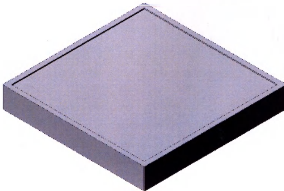
Потолок ламинарный медицинский ЛИТАЭРО по ТУ 32.50.50-007-37247008-2024 в варианте исполнения ЛИТАЭРО 2,6 х 1,8 С. Фильтр ОВП 381.05.
