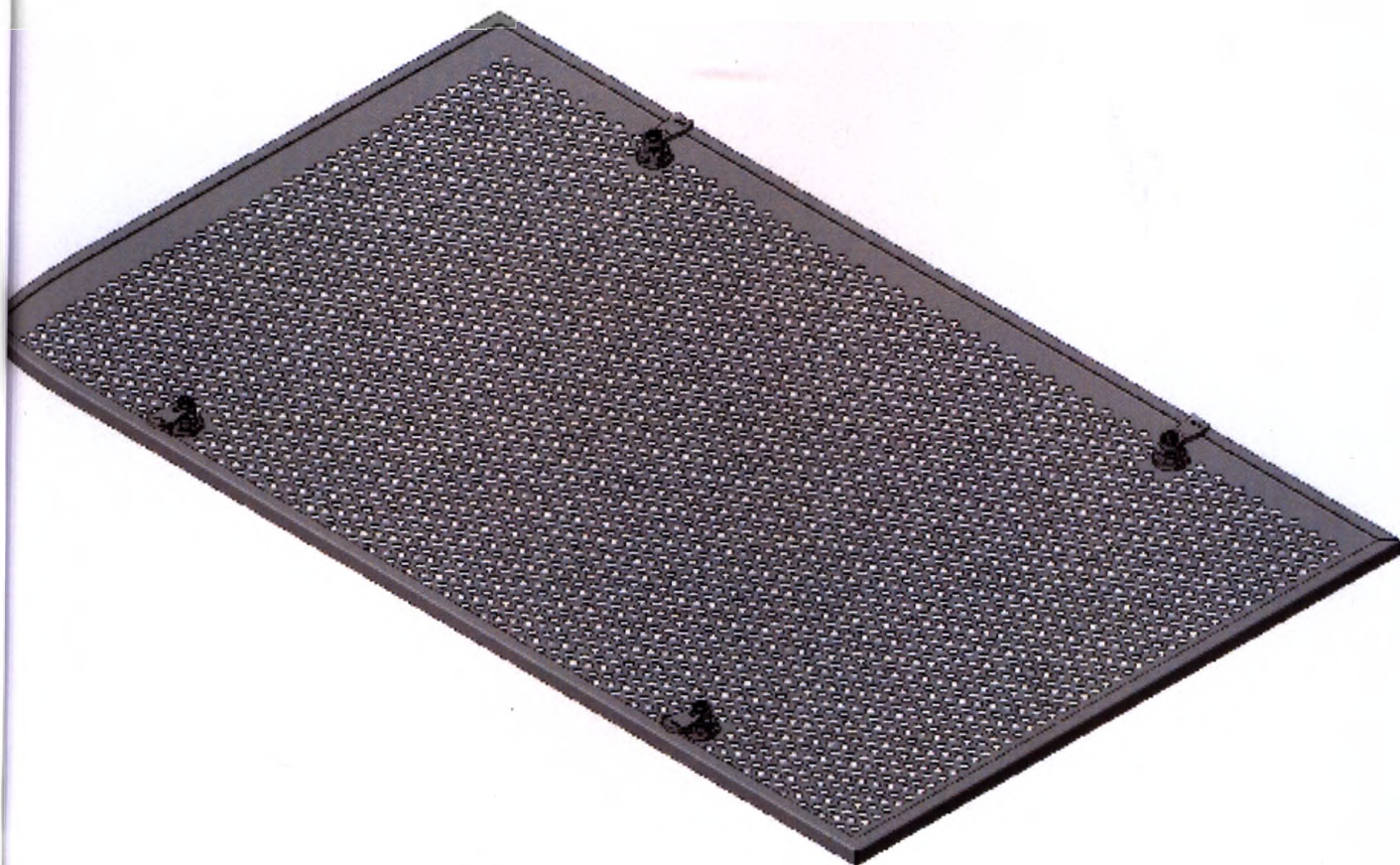
Потолок ламинарный медицинский ЛИТАЭРО по ТУ 32.50.50-007-37247008-2024 в варианте исполнения ЛИТАЭРО 1,8 х 1,0 С. Воздухораспределительная панель ОВП 378.02.
