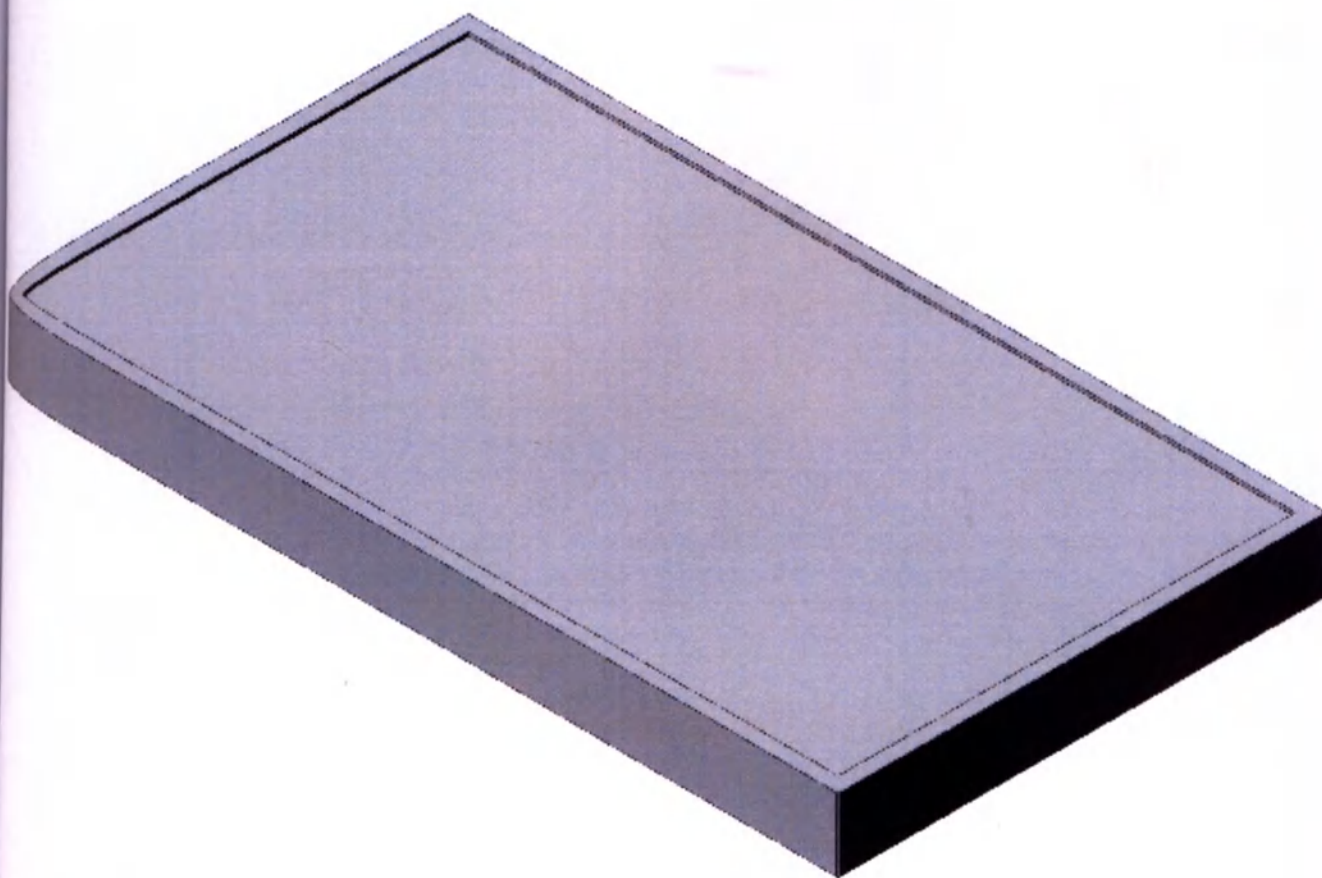
Потолок ламинарный медицинский ЛИТАЭРО по ТУ 32.50.50-007-37247008-2024 в варианте исполнения ЛИТАЭРО 2,6 х 1,8 С. Фильтр ОВП 378.05.
