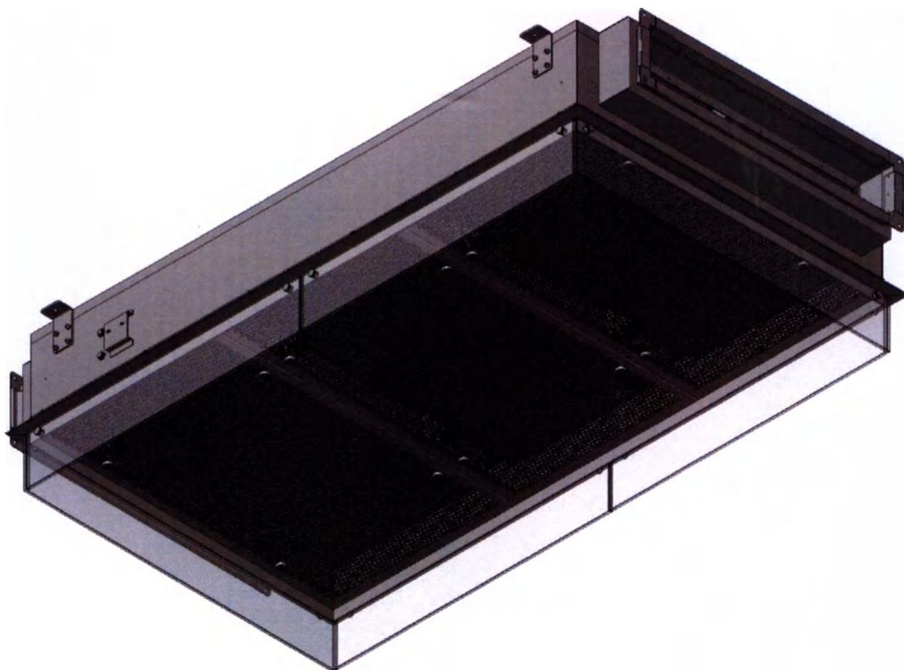
Потолок ламинарный медицинский ЛИТАЭРО по ТУ 32.50.50-007-37247008-2024 в варианте исполнения ЛИТАЭРО 1,8 x 1,0 С. Общий вид изделия
