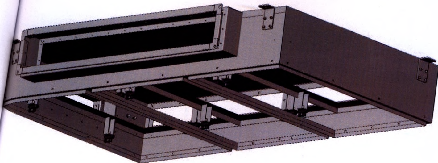
Потолок ламинарный медицинский ЛИТАЭРО по ТУ 32.50.50-007-37247008-2024 в варианте исполнения ЛИТАЭРО 2,0 х 1,8 С. Ячейка ОВП 402.01.02.
