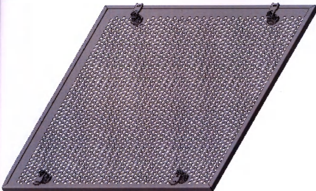
Потолок ламинарный медицинский ЛИТАЭРО по ТУ 32.50.50-007-37247008-2024 в варианте исполнения ЛИТАЭРО 2,6 x 1,8. Воздухораспределительная панель ОВП 381.02.
