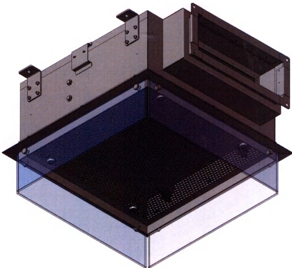
Потолок ламинарный медицинский ЛИТАЭРО по ТУ 32.50.50-007-37247008-2024 в варианте исполнения ЛИТАЭРО 0,6х0,6 С. Общий вид изделия
