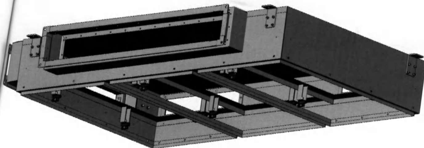
Потолок ламинарный медицинский ЛИТАЭРО по ТУ 32.50.50-007-37247008-2024 в варианте исполнения ЛИТАЭРО 2,6 x 1,8 С. Ячейка ОВП 401.01.01.
