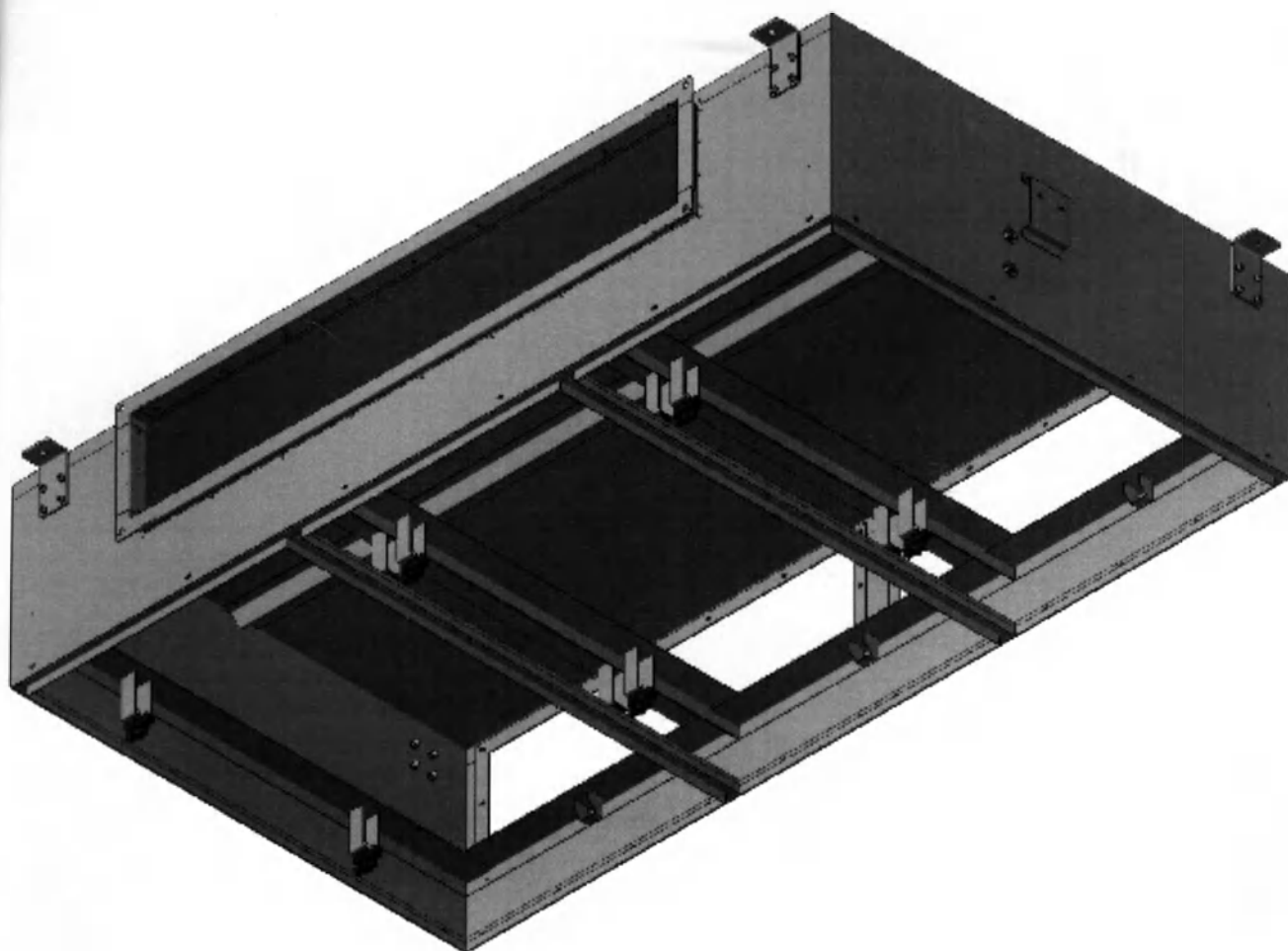
Потолок ламинарный медицинский ЛИТАЭРО по ТУ 32.50.50-007-37247008-2024 в варианте исполнения ЛИТАЭРО 2,0 x 1,8. Ячейка ОВП 379.01.01.
