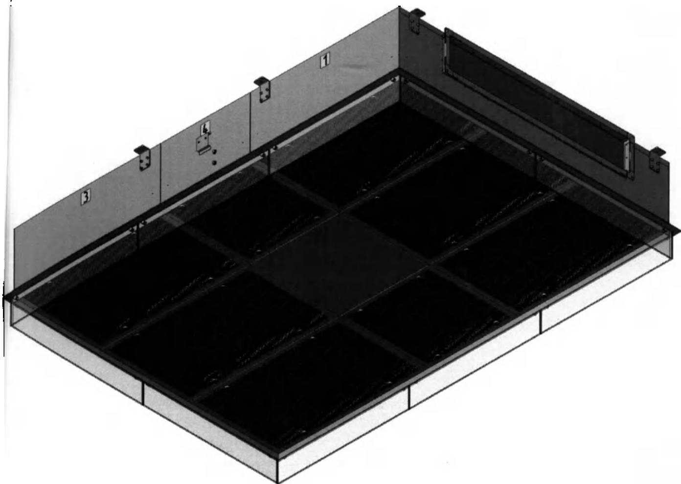
Потолок ламинарный медицинский ЛИТАЭРО по ТУ 32.50.50-007-37247008-2024 в варианте исполнения ЛИТАЭРО 2,6 х 1,8. Общий вид изделия
