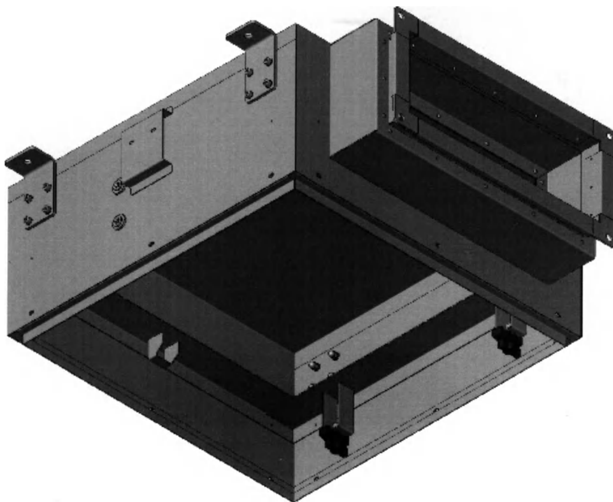
Потолок ламинарный медицинский ЛИТАЭРО по ТУ 32.50.50-007-37247008-2024 в варианте исполнения ЛИТАЭРО 0,6х0,6 С. Ячейка ОВП 405.01.
