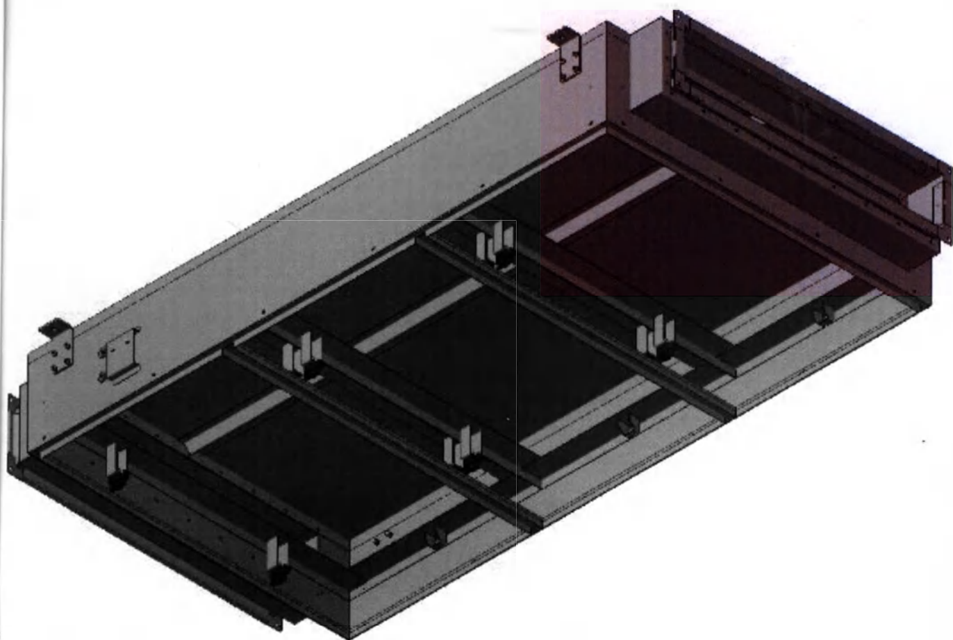
Потолок ламинарный медицинский ЛИТАЭРО по ТУ 32.50.50-007-37247008-2024 в варианте исполнения ЛИТАЭРО 1,8 x 1,0 С. Ячейка ОВП 403.01
