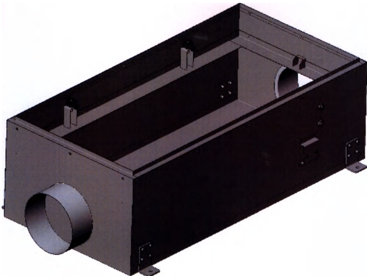
Потолок ламинарный медицинский ЛИТАЭРО по ТУ 32.50.50-007-37247008-2024 в варианте исполнения ЛИТАЭРО 1,2x0,6. Ячейка ОВП 380.01
