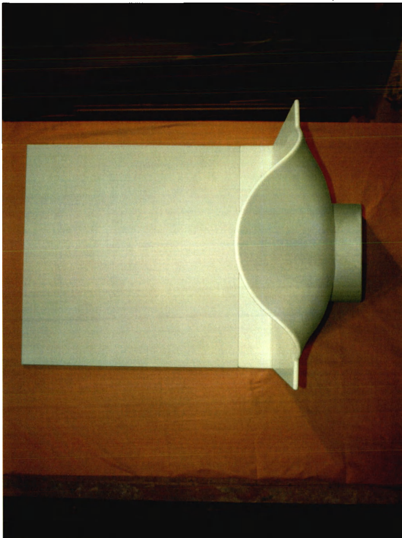
Мойка медицинская хирургическая макси с одной чашей ММХМ-1-В со стеновой панелью С-1-В, с защитным кожухом К-В
