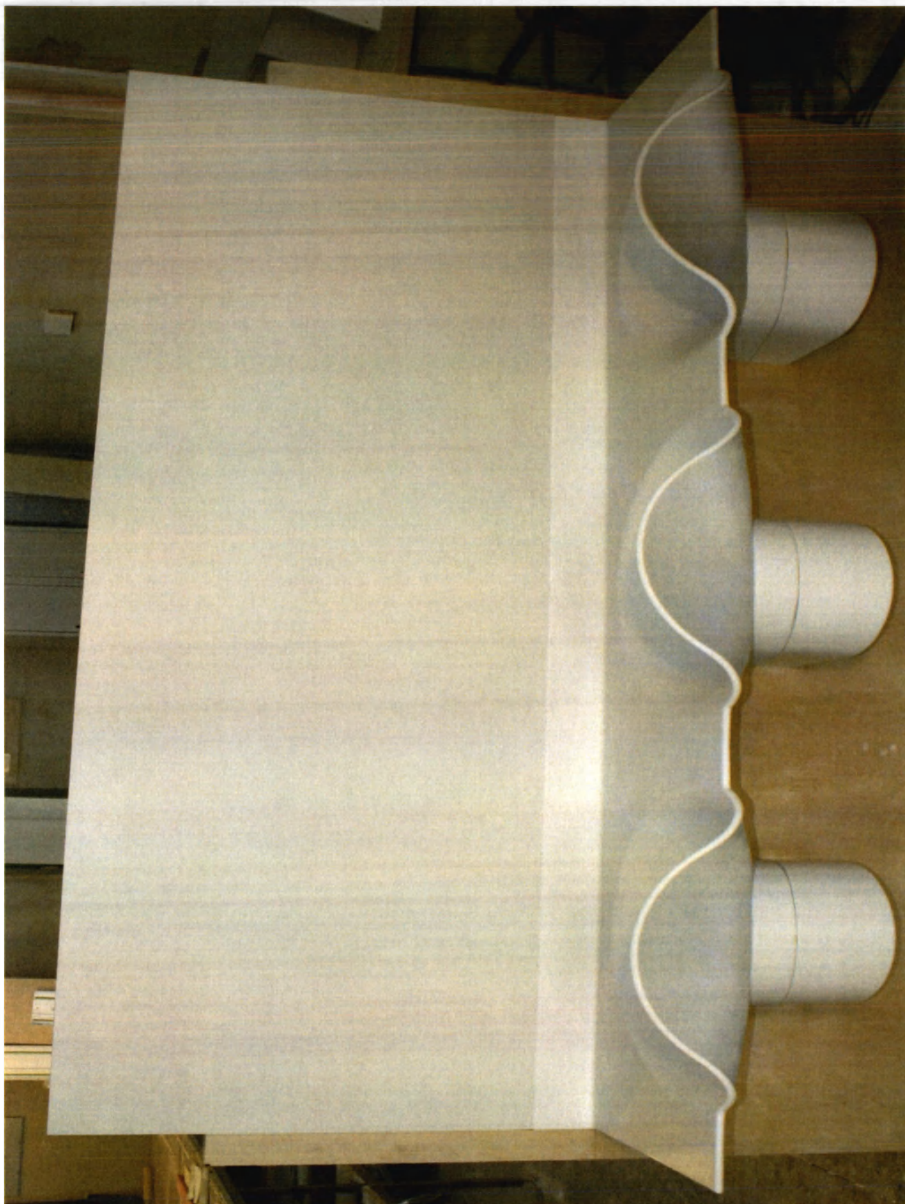
Мойка медицинская хирургическая глубокая с тремя чашами ММХГ-3-А со стеновой панелью С-3-А, с защитным кожухом К-А
