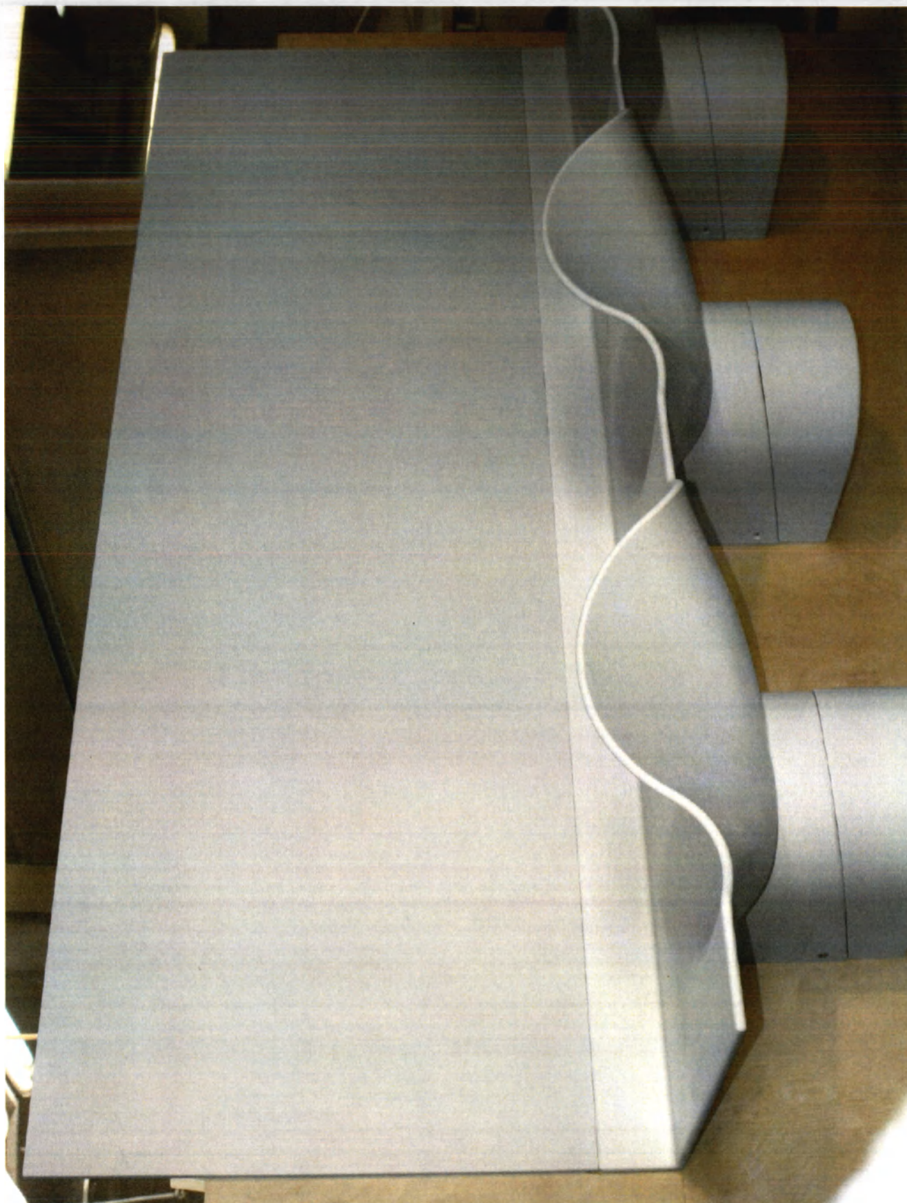
Мойка медицинская хирургическая стандарт с тремя чашами ММХС-3-Б со стеновой панелью С-3-Б, с защитным кожухом К-Б
