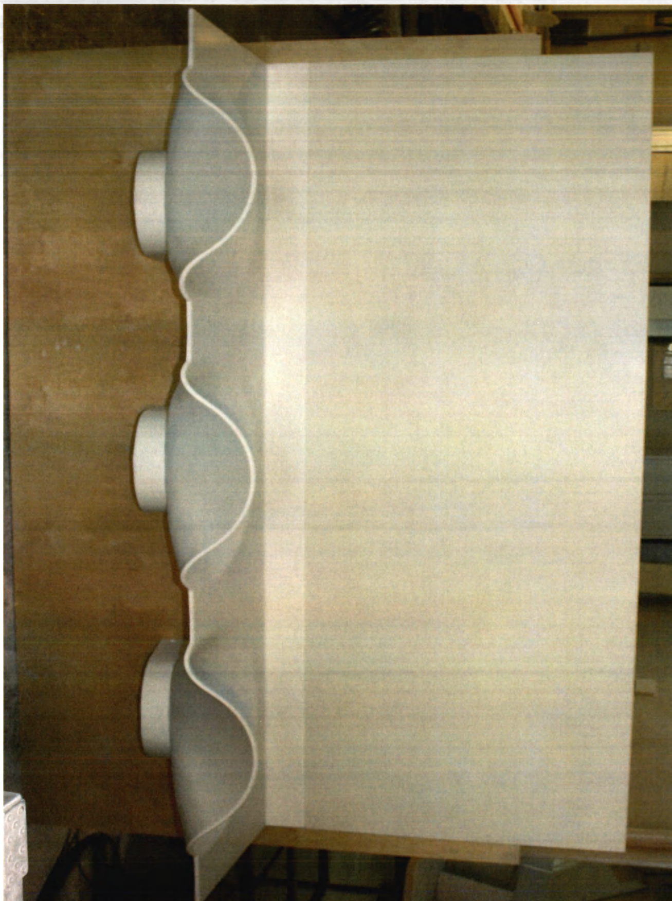
Мойка медицинская хирургическая макси с тремя чашами ММХМ-3-А со стеновой панелью С-3-А
