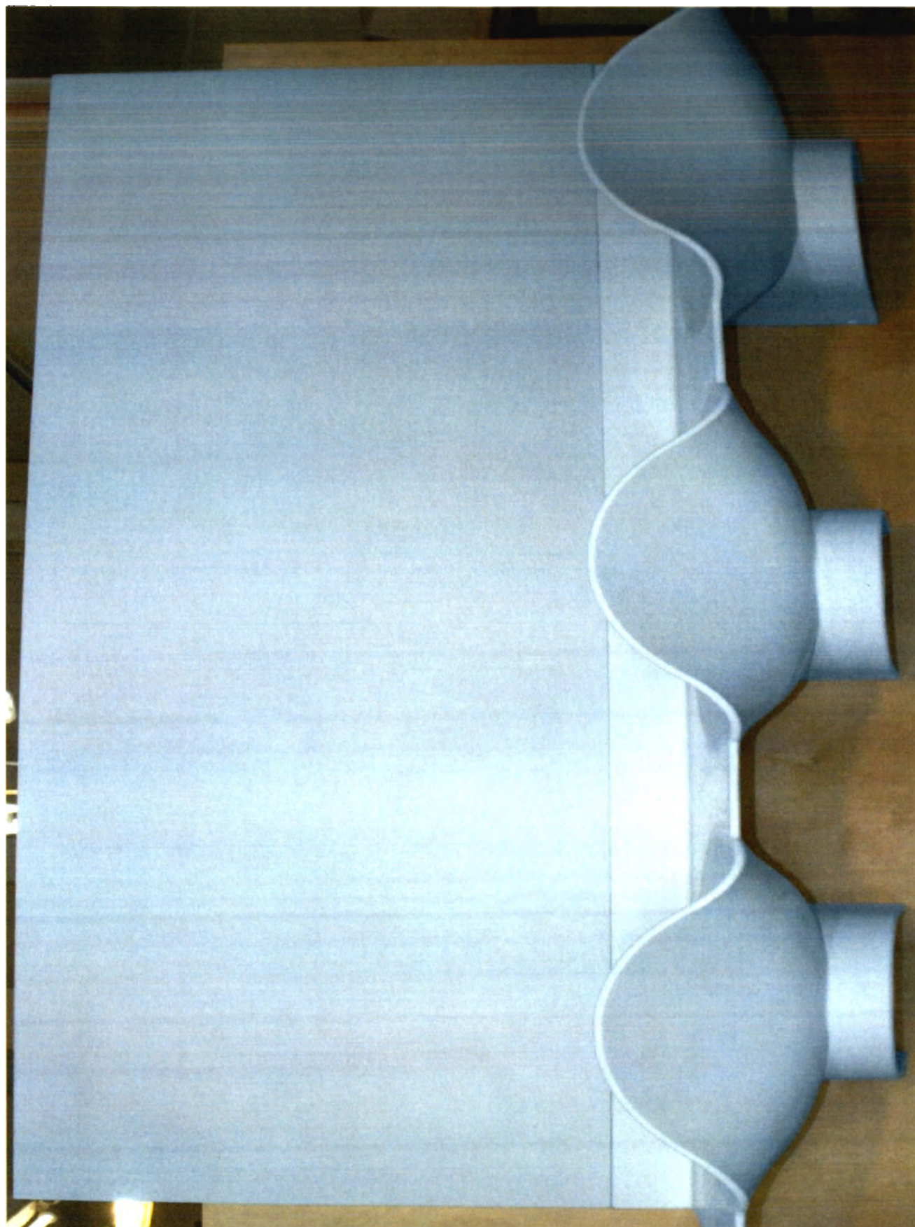
Мойка медицинская хирургическая глубокая с тремя чашами ММХГ-3-Г со стеновой панелью С-3-Г
