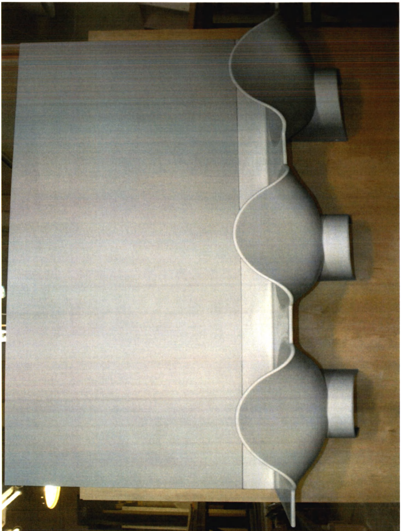
Мойка медицинская хирургическая макси с тремя чашами ММХМ-3-Б со стеновой панелью С-3-Б
