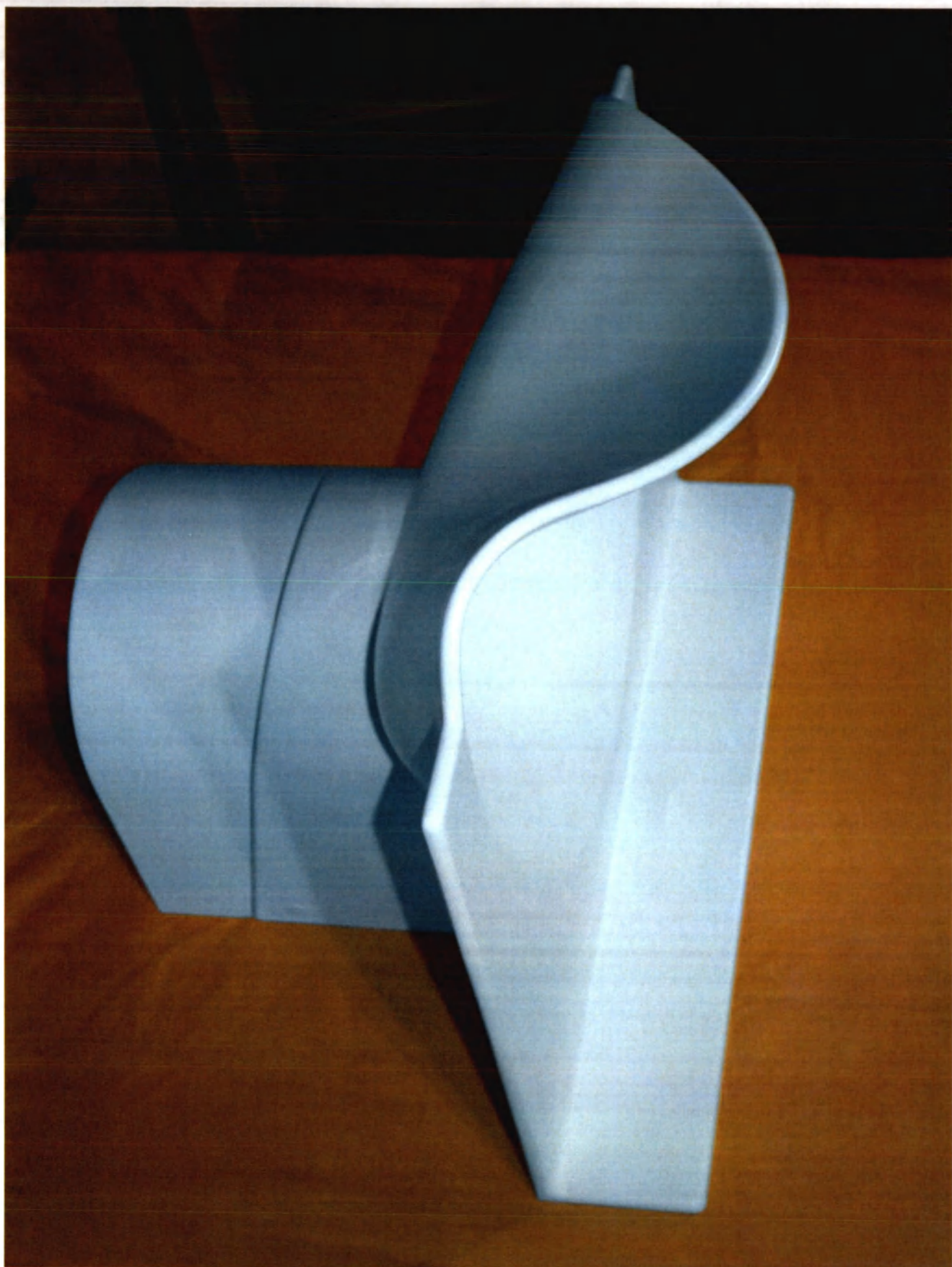
Мойка медицинская хирургическая стандарт с одной чашей ММХС-1-Г с защитным кожухом К-Г
