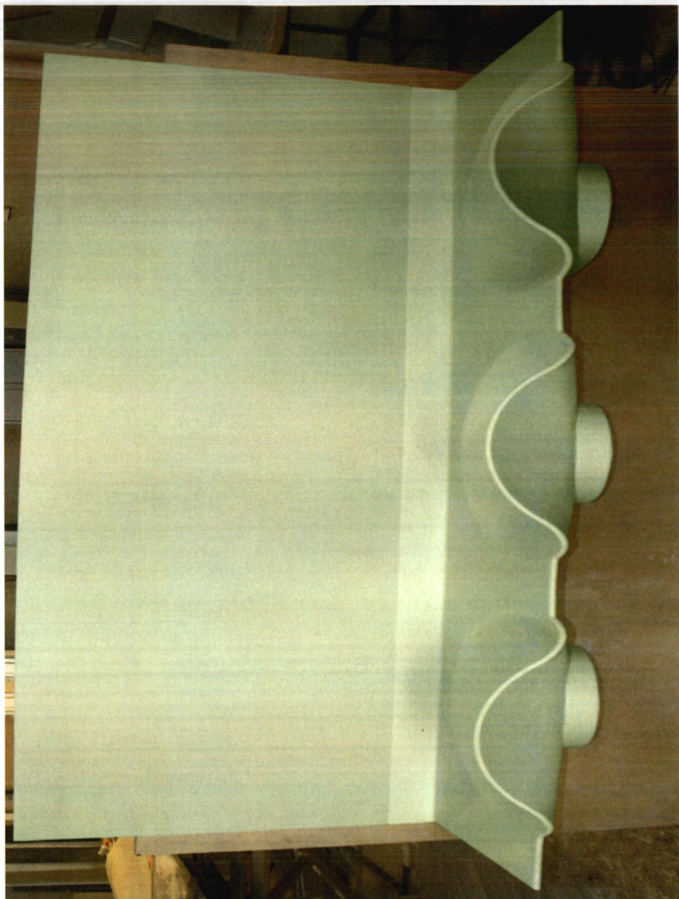
Мойка медицинская хирургическая стандарт с тремя чашами ММХС-3-В со стеновой панелью С-3-В
