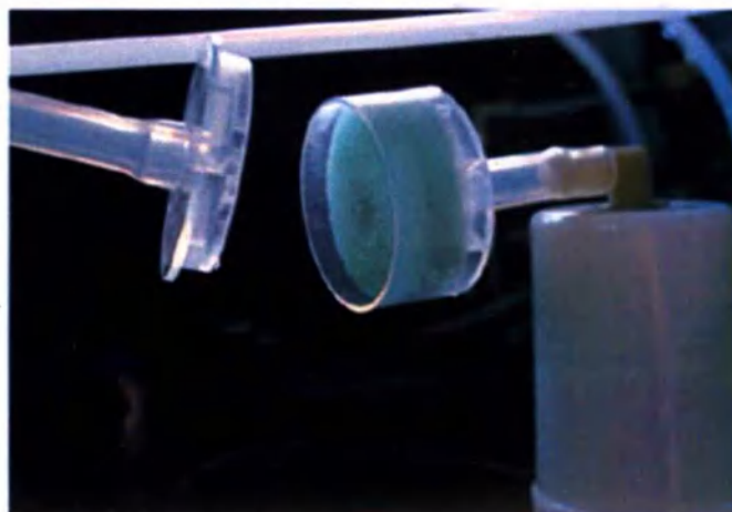
Рис.24. Второй воздушный фильтр (Фильтр тонкой очистки). Концентратор медицинский кислородный Longfian Jay-10D
