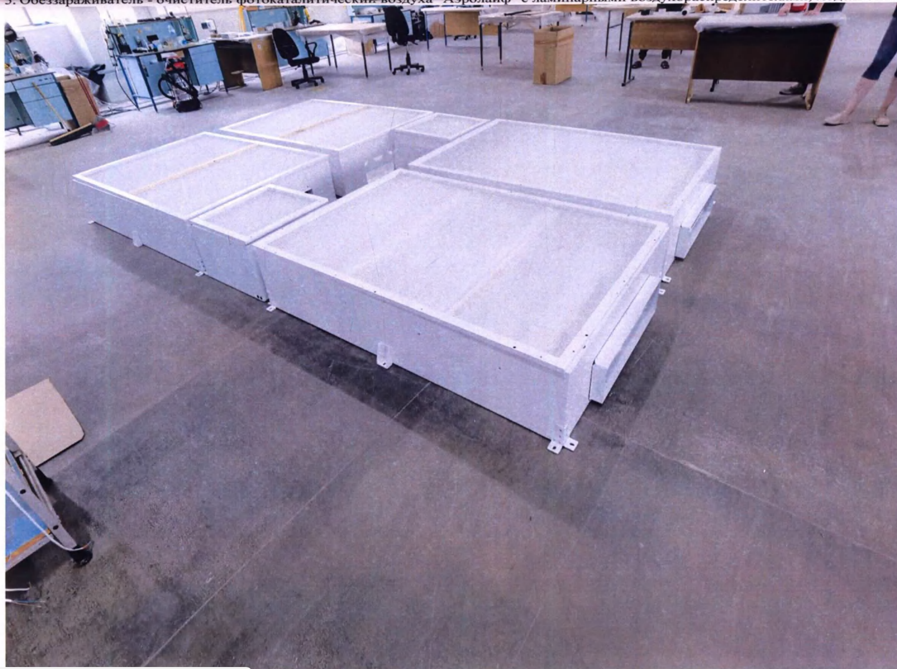
5. Обеззараживатель - очиститель фотокаталитический воздуха "Аэролайф" с ламинарными воздушными распределителями, модель ЛАМ 7002
