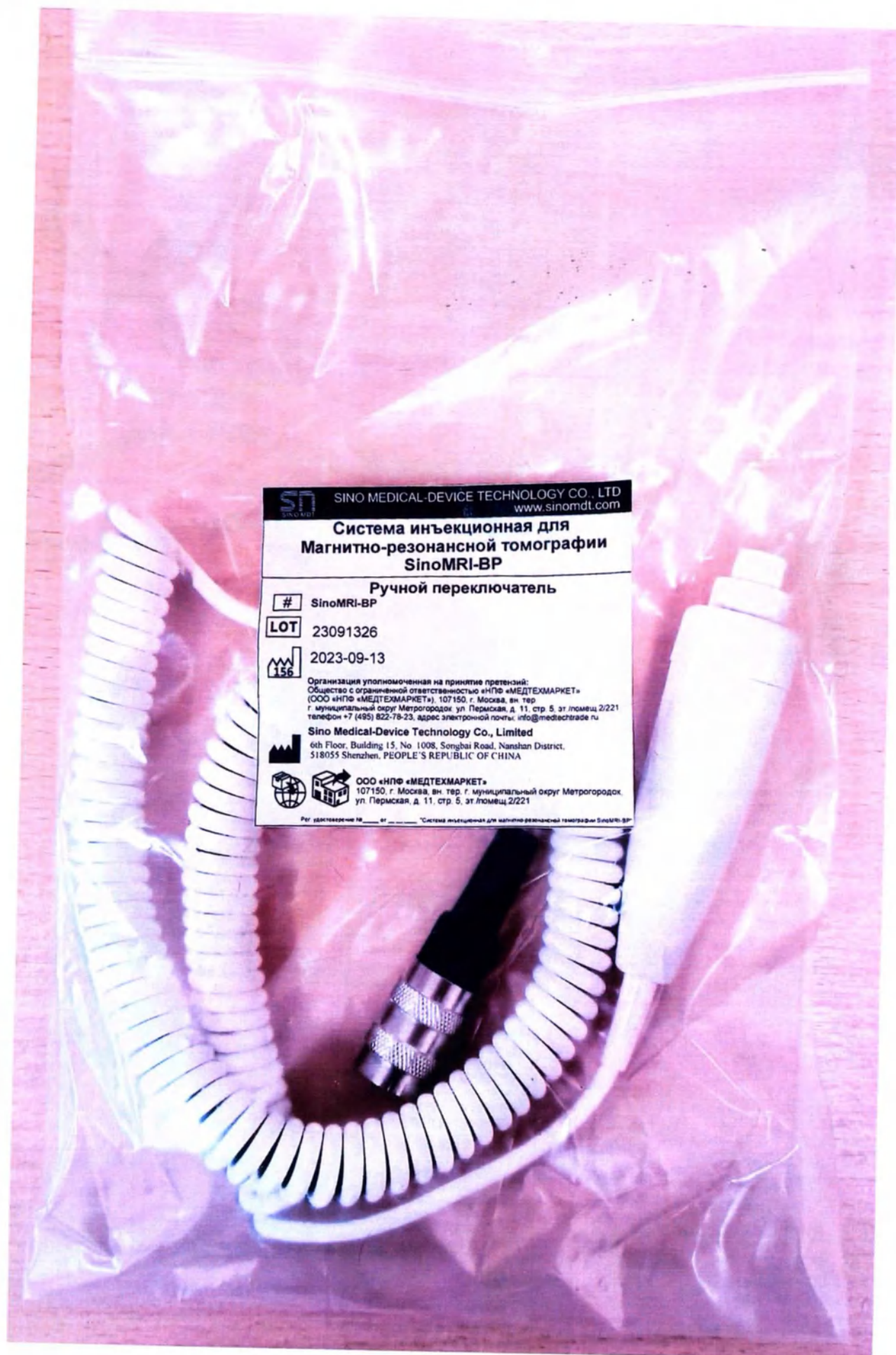
Фотографическое изображение ручного переключателя в упаковке.
