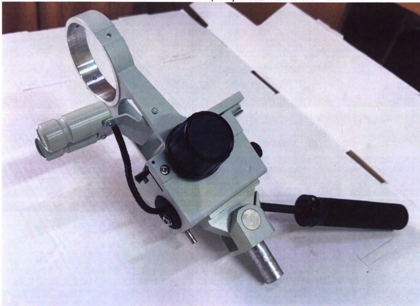
Кронштейн оптической головки с механизмом точной фокусировки и осветителем и зелёным фильтром БАВ-089.005.000
