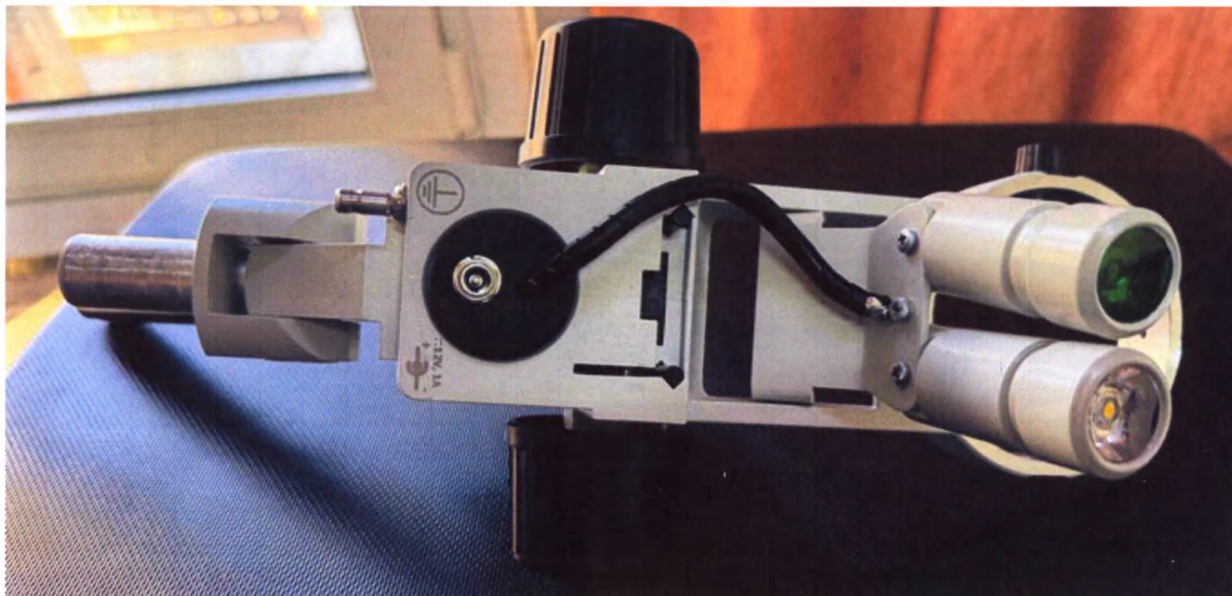
Кронштейн оптической головки с механизмом точной фокусировки и осветителем и зелёным фильтром БАВ-089.005.000 (маркировка)
