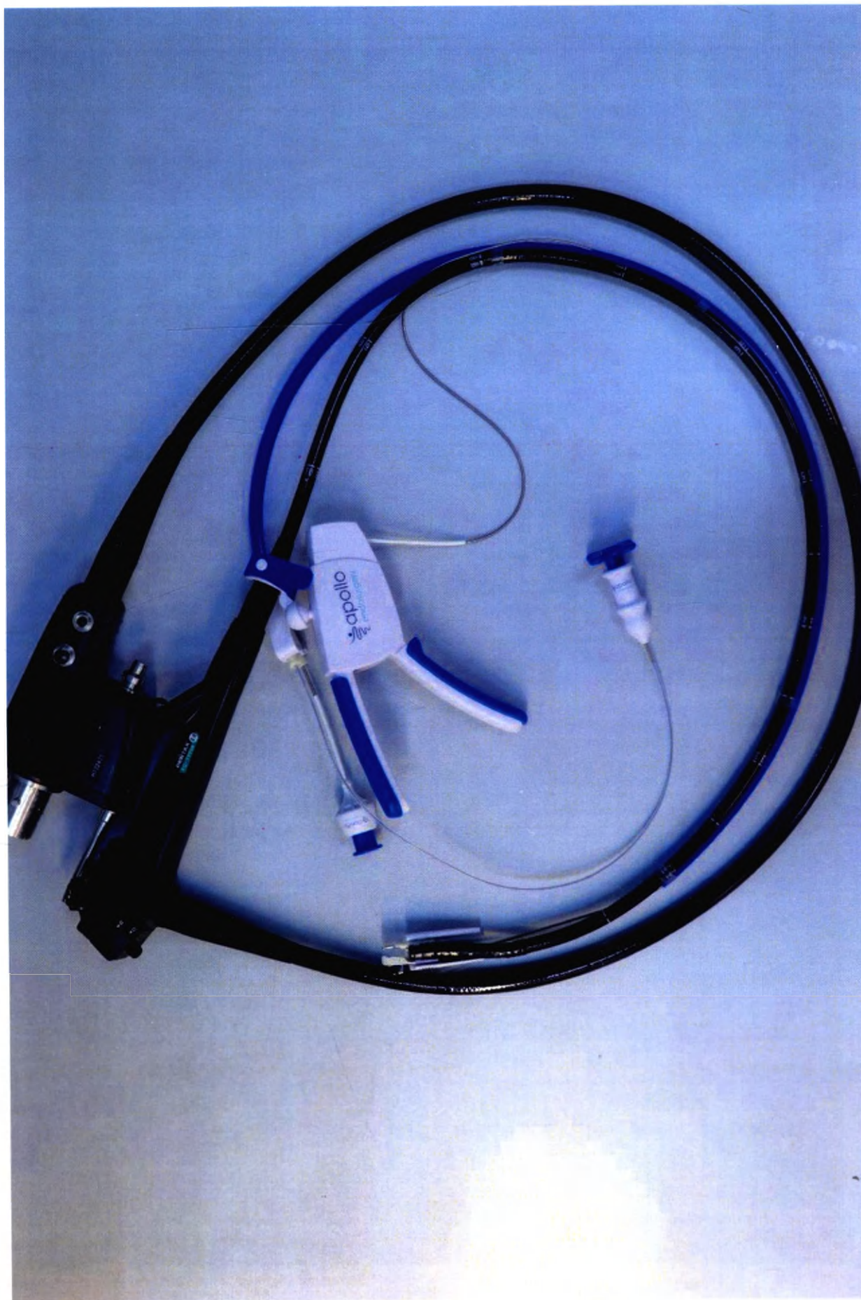
Система сшивающая эндоскопическая OverStitch Sx, установлена на эндоскоп
