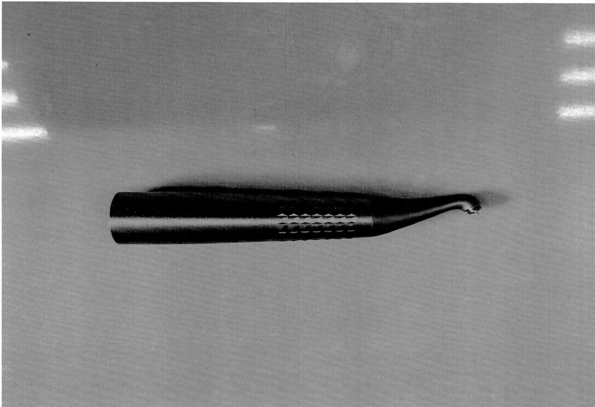
Наконечник воздушно-абразивный для полировки зубов со съемной головкой (Air polishing handpiece) AP-2
