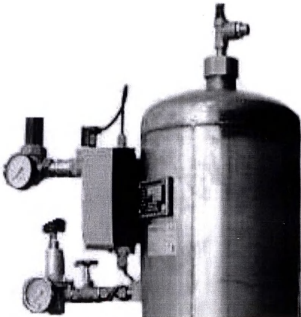
19. Аппарат для обогащения воды O2 (отличие в управлении и давлении )
