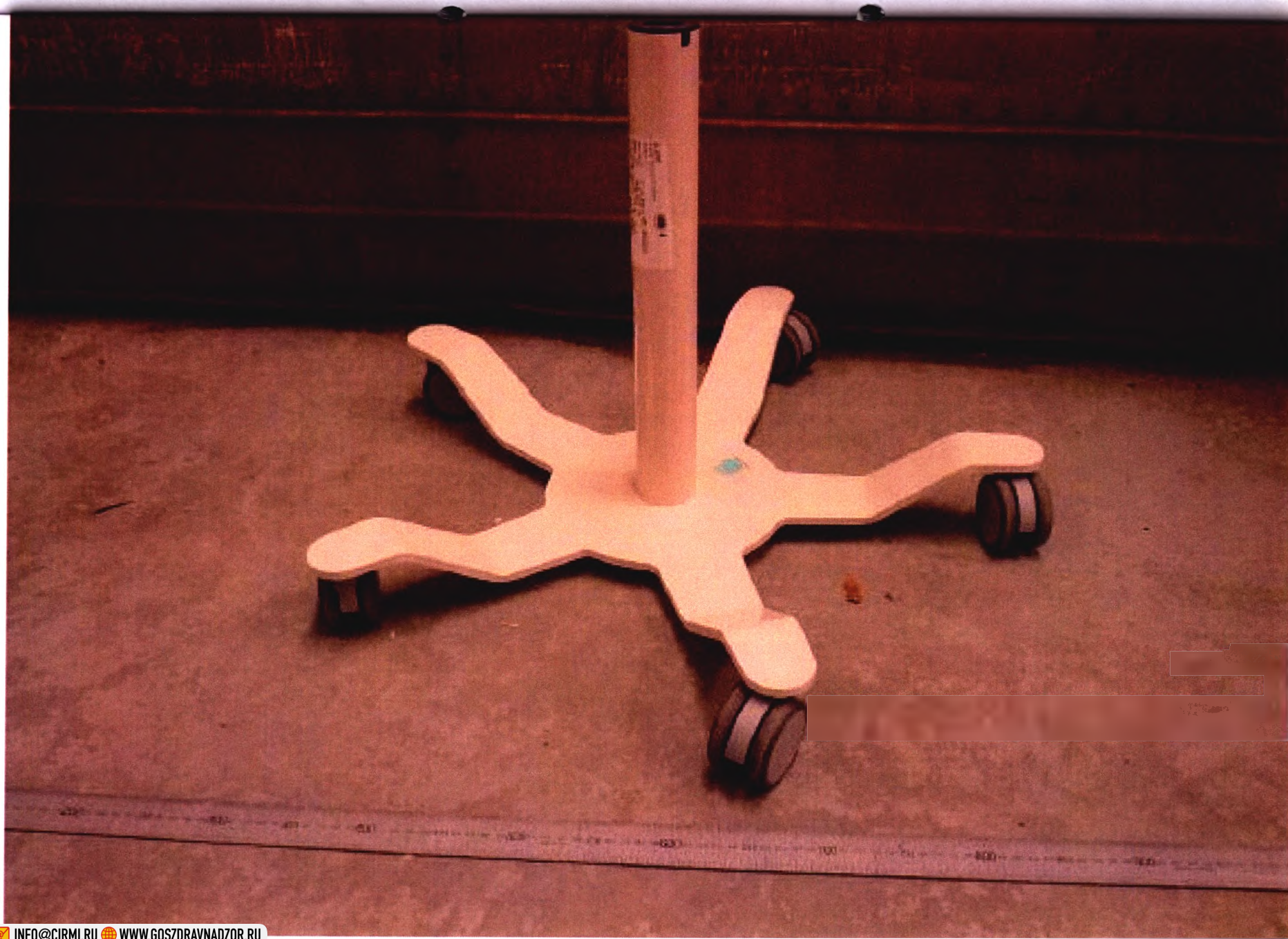
Рис. 14 Передвижной держатель для кислородного баллона (Mobile oxygen cylinder carrier base)
