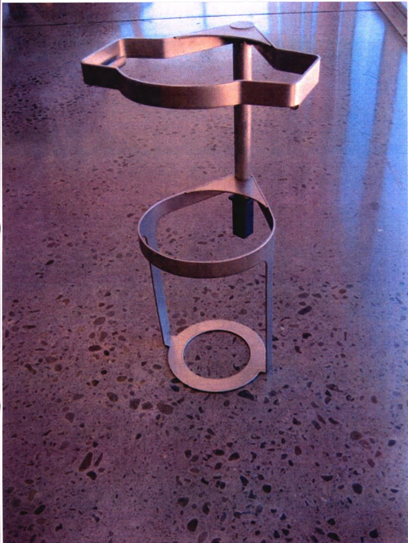
Рис. 16 Держатель для кислородного баллона размер D (Oxygen cylinder carrier for "D" size)
