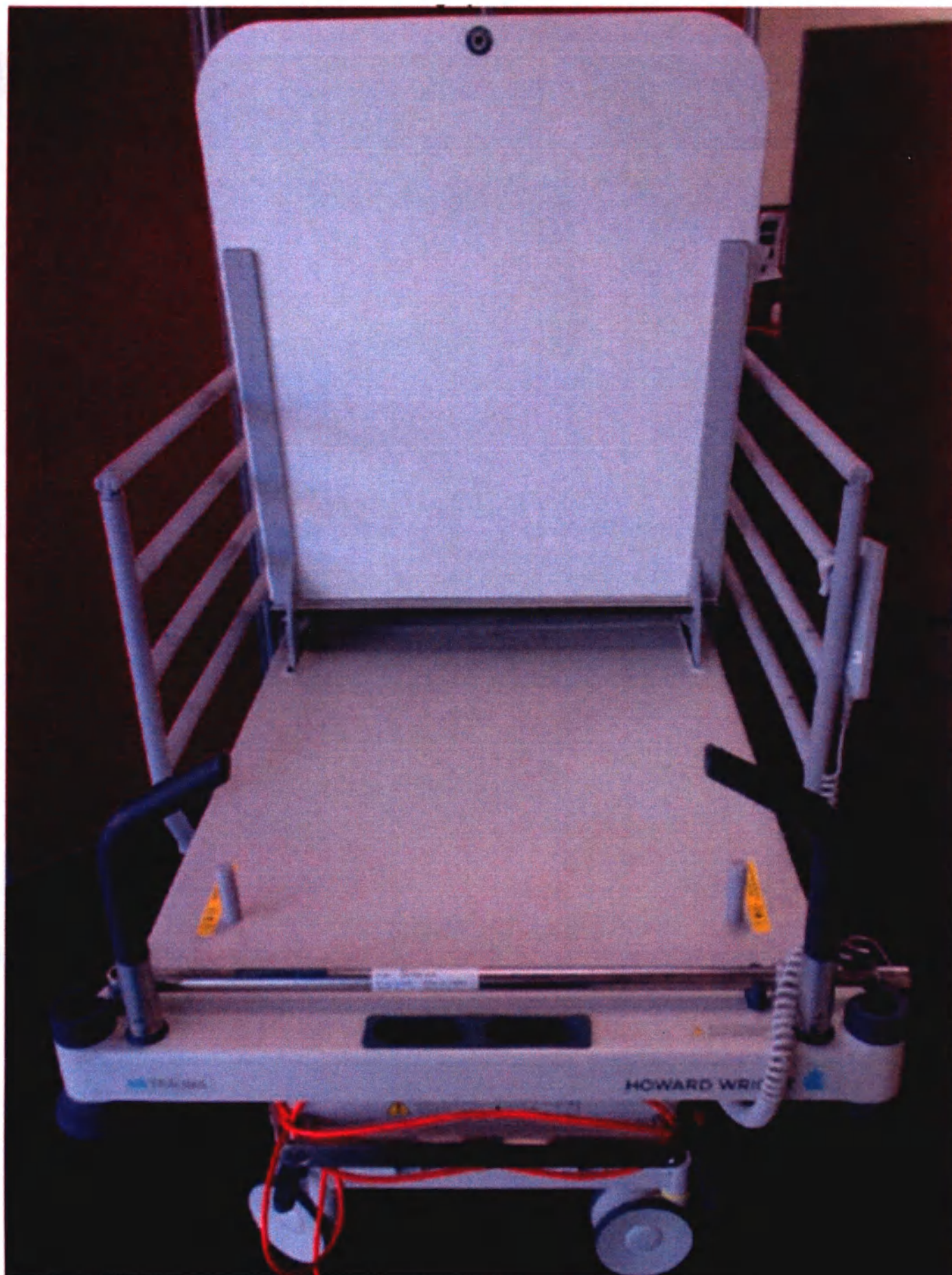
Рис. 3 Каталка медицинская функциональная М9 TRAUMA с принадлежностями (вид со стороны изголовья)
