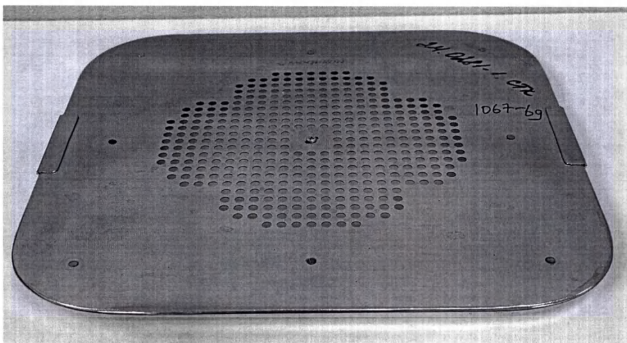
Фото 8 – Крышка контейнера ККУ-«МЕДИКОН» (общий вид)
