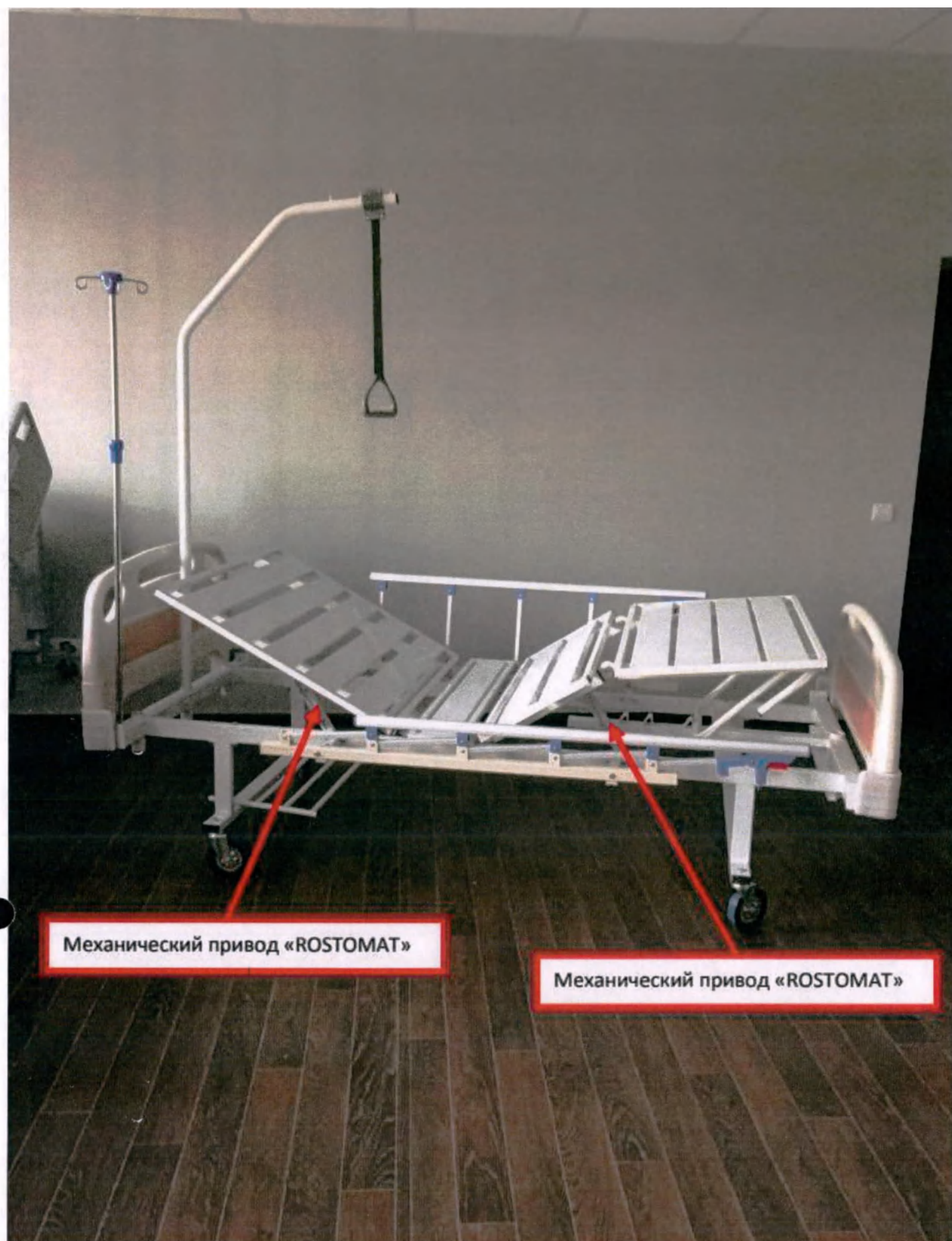
Фотографическое изображение 107 – Механический привод регулировки секций МК701.0М0.0011 Кровать медицинская функциональная, модель 4М2
