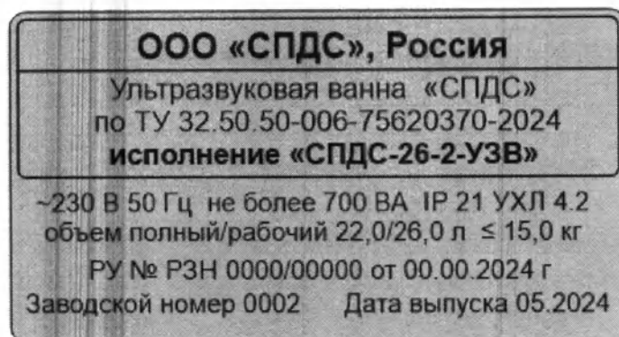
Фотография 43. Ультразвуковая ванна «СПДС – 26-2 - УЗВ».
