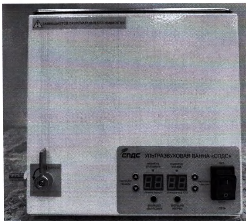
Фотография 1. Ультразвуковая ванна «СПДС - 4 - УЗВ». Вид спереди.
