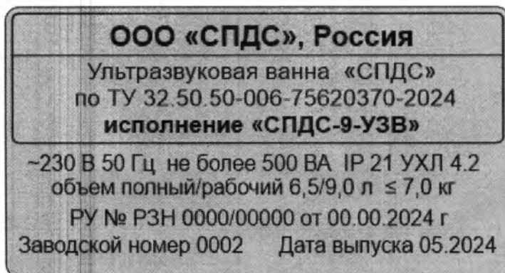
Фотография 20. Ультразвуковая ванна «СПДС - 9 - УЗВ». Маркировка изделия.
