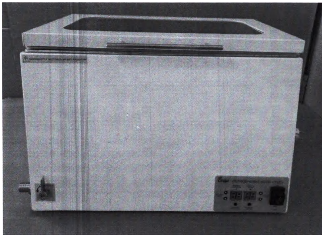
Фотография 36. Ультразвуковая ванна «СПДС - 26 -2- УЗВ». Вид спереди
