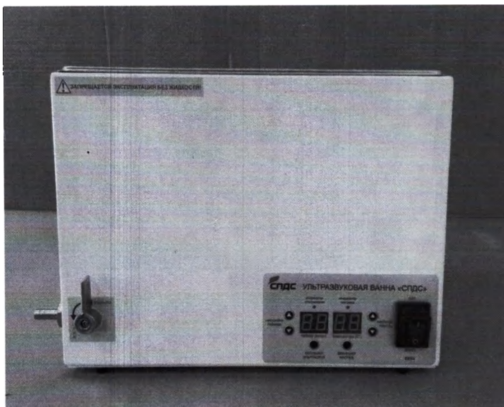
Фотография 13. Ультразвуковая ванна «СПДС - 9 - УЗВ». Вид спереди.
