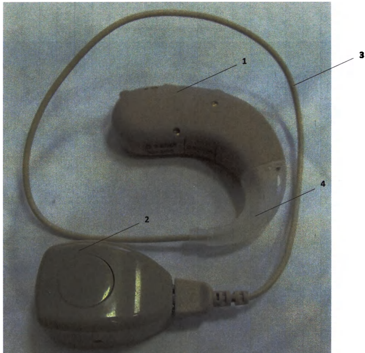
Аппарат слуховой электронный реабилитационный костного звукопроведения цифровой программируемый «Лурика» «Дорема» вид (2) на примере модели T4DM в составе: 1 – аппарат слуховой, 2 - телефон костной проводимости, 3 - соединительный шнур, 4 – розжок.
